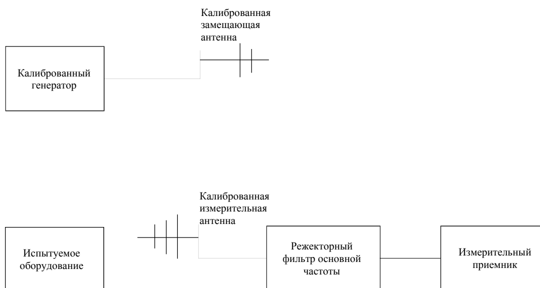
Установка для измерения э.и.и.м. излучений в области побочных излучений
