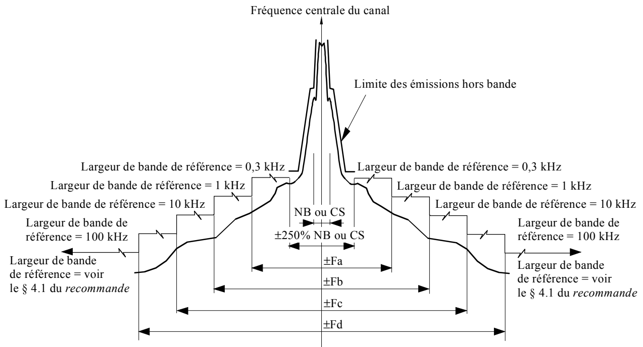
FIGURE 3 Gabarit générique des rayonnements non désirés dans le domaine des rayonnements non essentiels pour des stations du service fixe relevant de la catégorie B (voir le Tableau 11)
