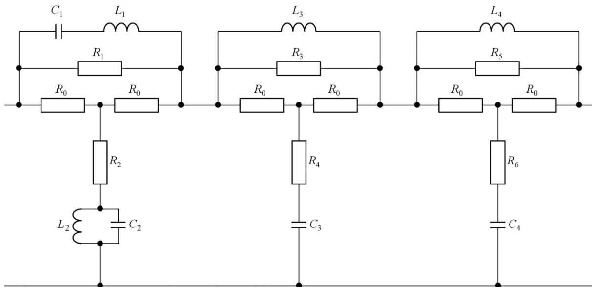
Red ponderadora del generador de la señal telefónica convencional
