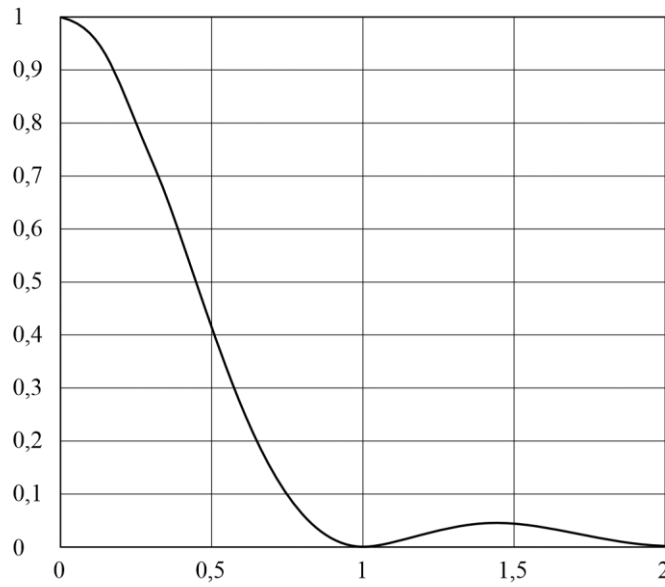
FIGURA 26 Espectro MDP-2
