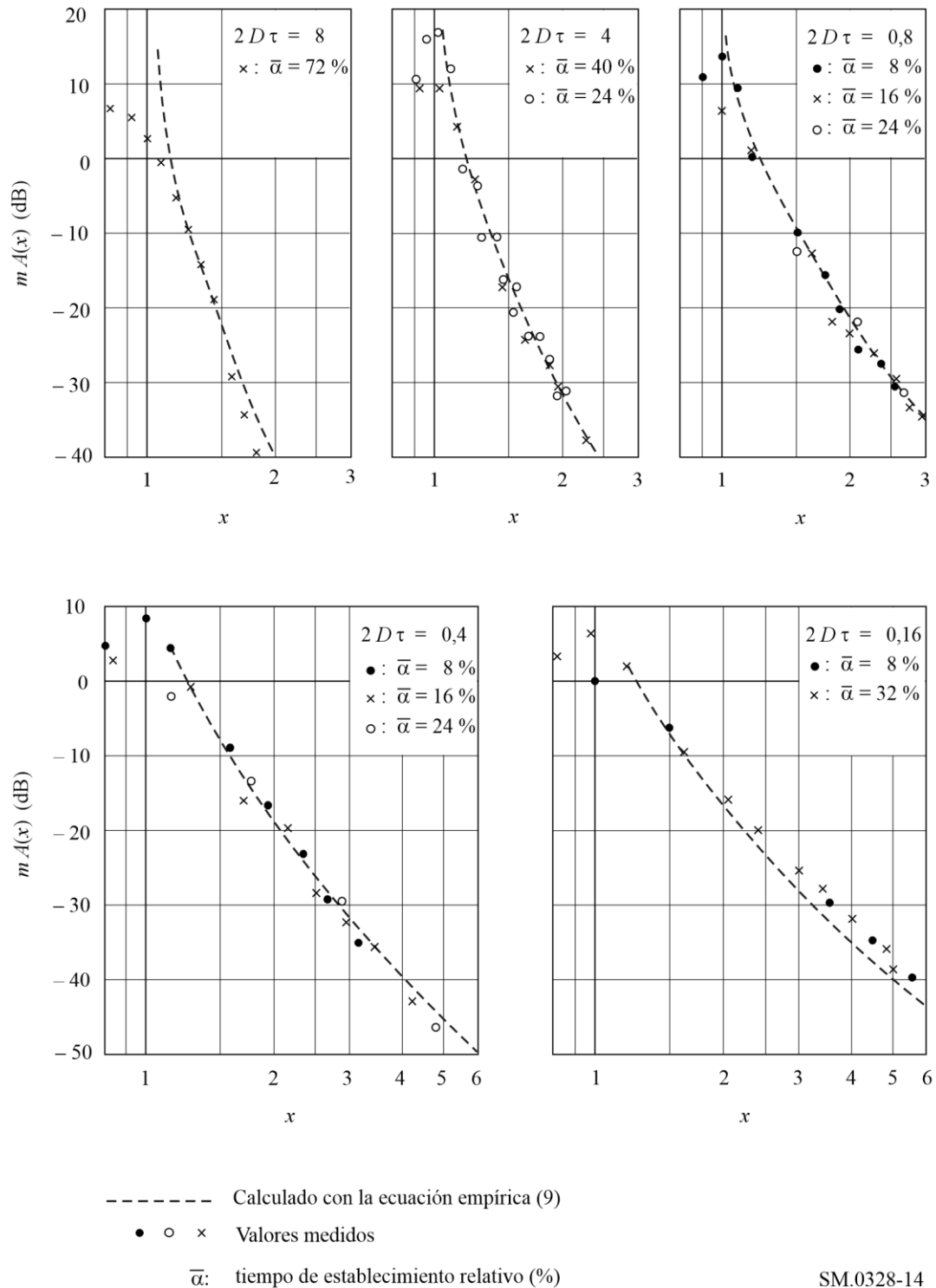
FIGURA 14 Espectro de las emisiones de tipo F1B
