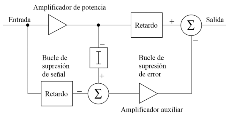
FIGURA 46 Precompensación
