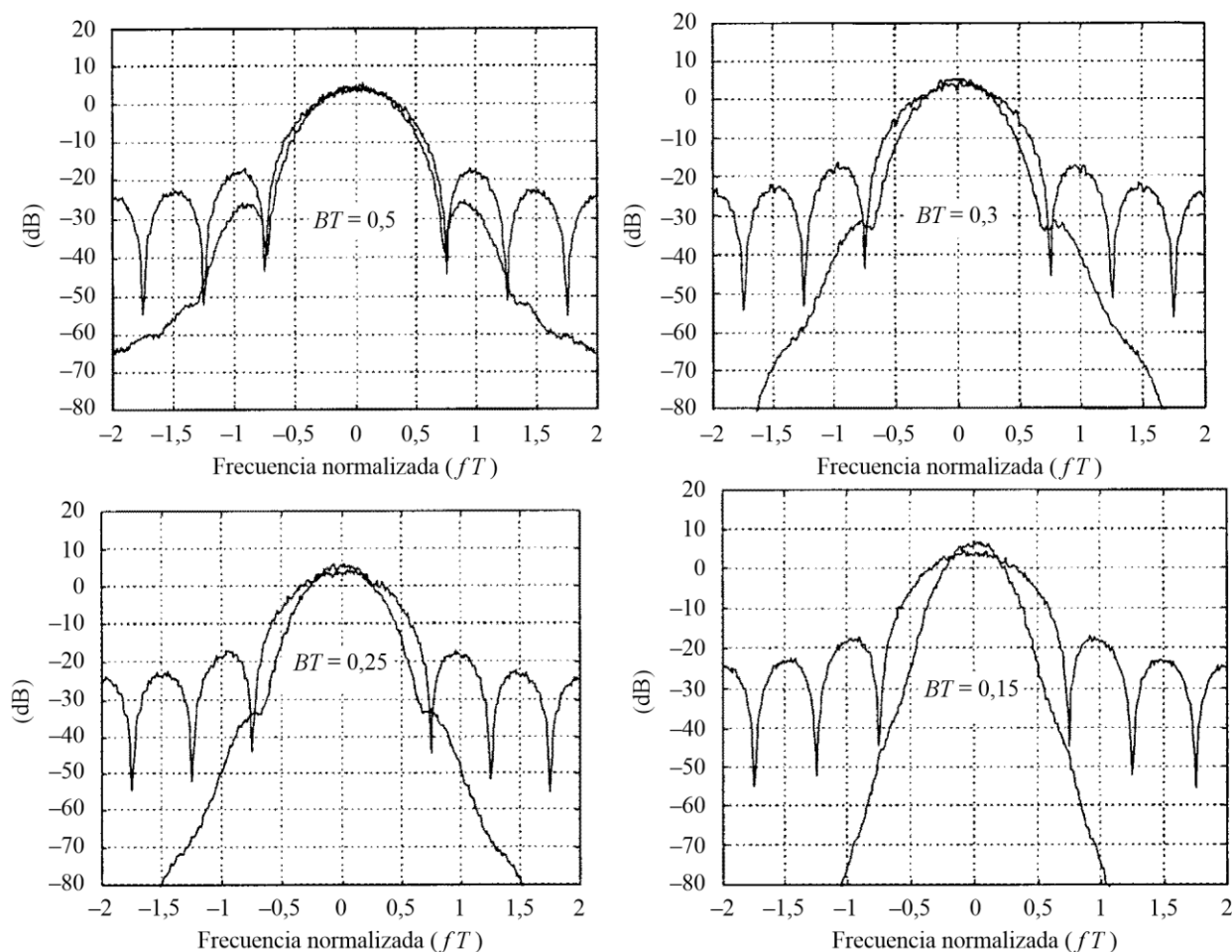
FIGURA 32 Espectros de MDMG para BT = 0,5, 0,3, 0,25 y 0,15
