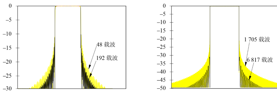
图36 OFDM功率谱密度
