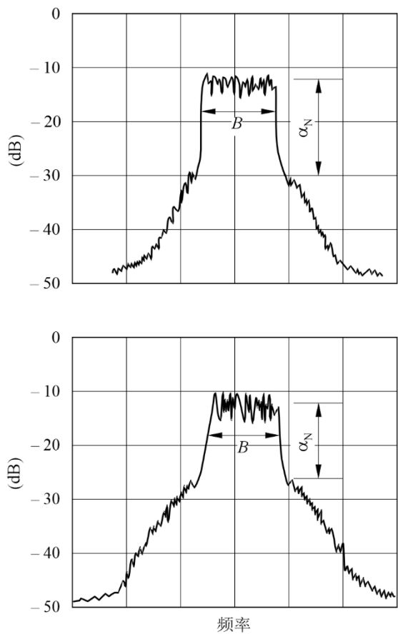
白噪声调制的J3E类发射的频谱包络
