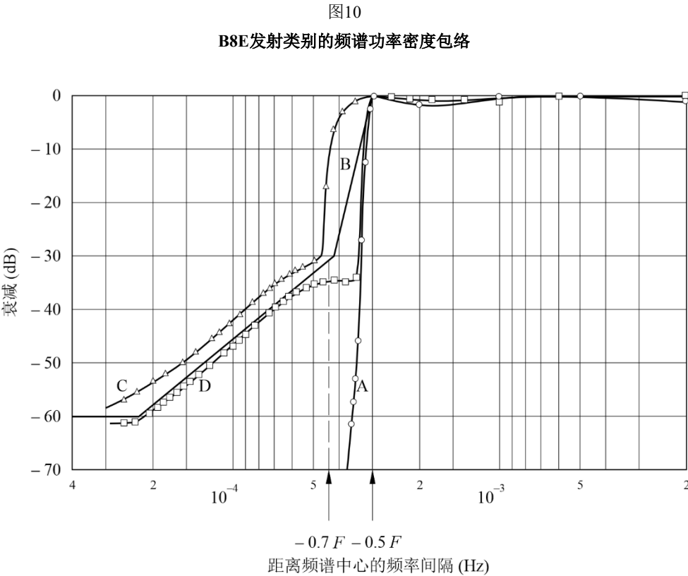
F : 必要带宽 (6 000 Hz) 曲线 A: 发射机的滤波器特性 B: 附件1的§ 5.4.3 规定的限制曲线 C: 使用通带为 3 800 Hz的分析仪测量得到的曲线 D: 使用通带为100 Hz左右的分析仪测量得到的曲线
