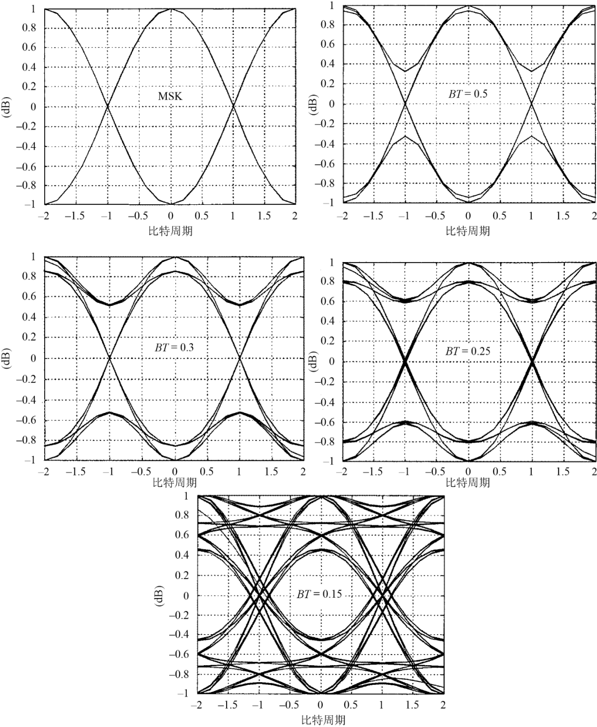
图33 眼图
