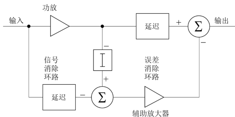
图46 前馈
