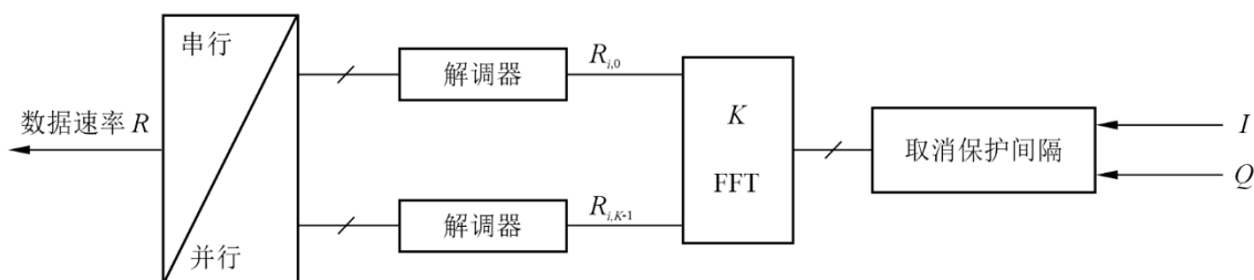
图35 OFDM接收机
