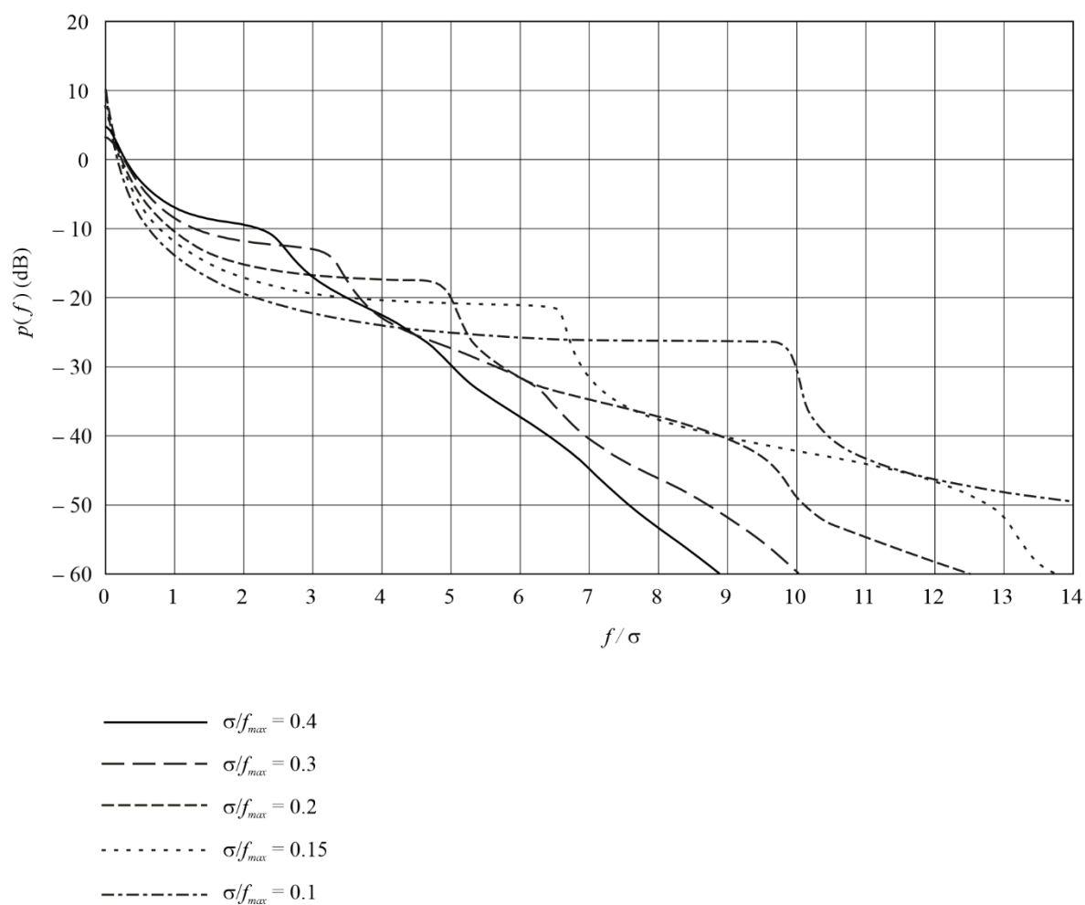
图18 \sigma / f_{max} < 0.5 时的功率谱分布
