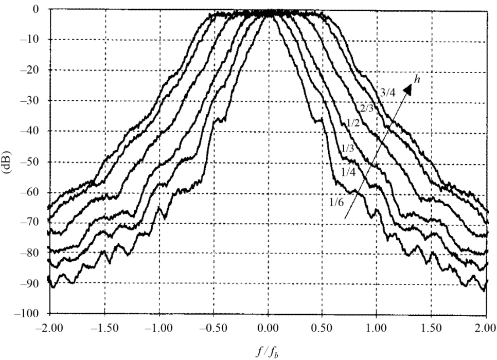
图31 4状态CPM的模拟功率密度谱（2RC脉冲）
