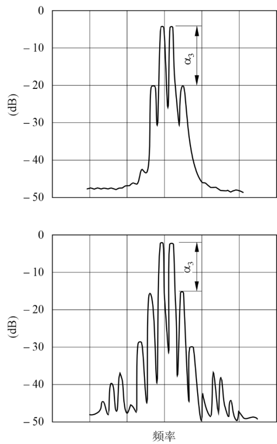
两个正弦信号调制的J3E类发射的频谱包络
