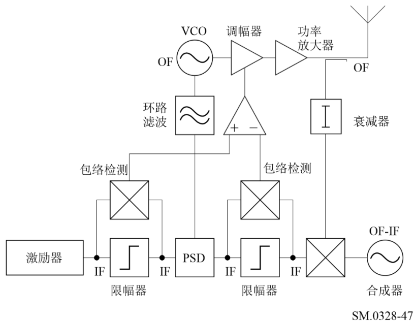
图47 极化环技术
