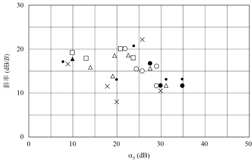
图25 不同的 \alpha_3 值对应的带宽附近的斜率值
