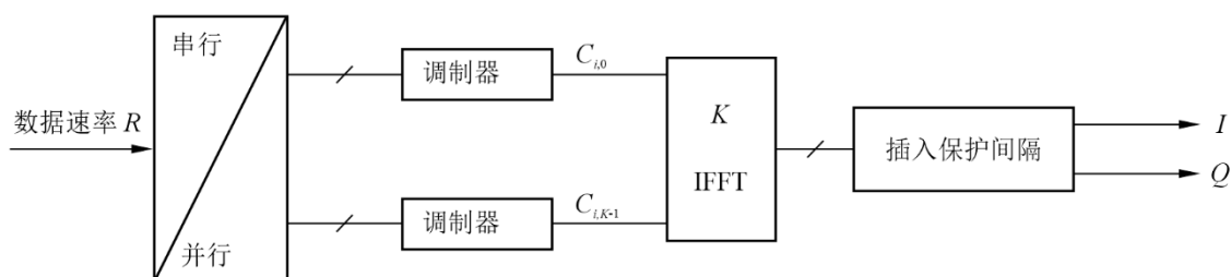
图34 OFDM发射机
