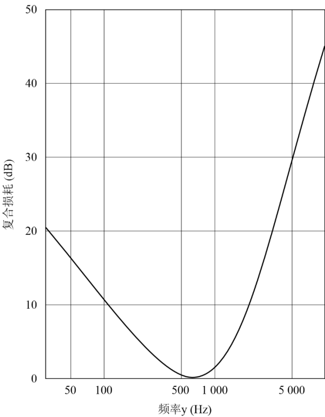
图4 常规电话信号发生器整形网络的相对响应曲线
