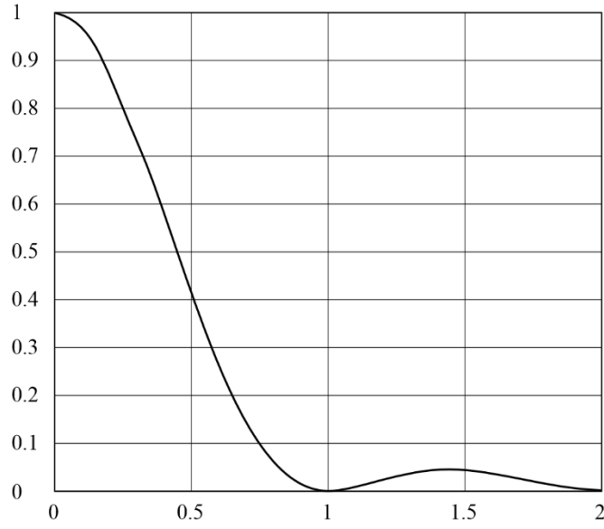
图26 BPSK频谱
