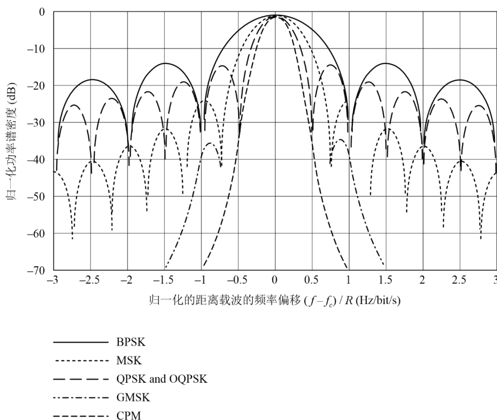
一些调制方法示例的功率谱密度
