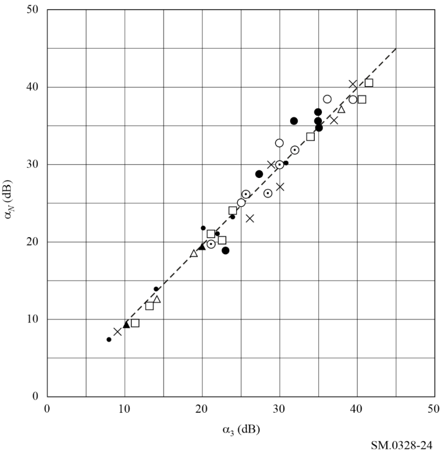
图23中不同的 \alpha_3 值对应的 \alpha_N 值
