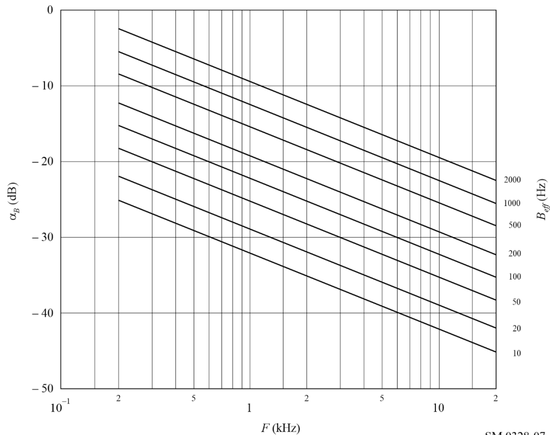
在均方根调制系数为35%的条件下，以分析设备的有效噪声带宽( B_{eff} )为参数，A3E类发射的带外频谱限制曲线的 0 \text{ dB} 基准电平与载波电平之比 \alpha_B(\text{dB}) 随必要带宽 F(\text{kHz}) 的变化
