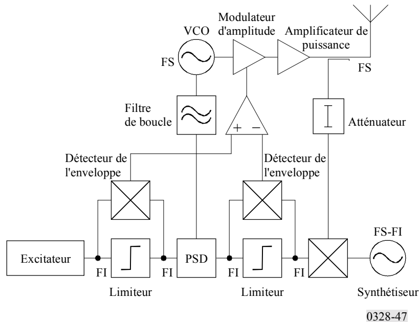
Technique à boucle polaire
