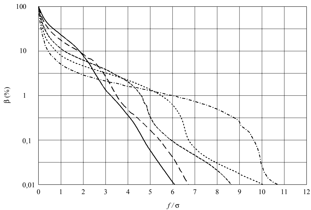
FIGURE 20 Puissance hors bande du spectre pour \sigma/f_{max} < 0,5
