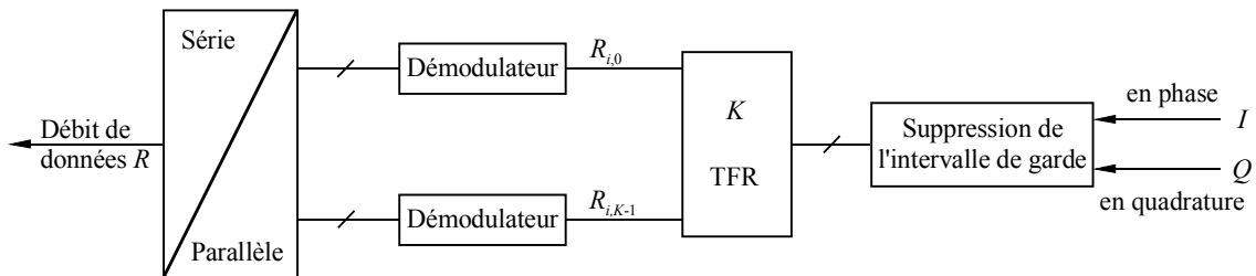
FIGURE 35 Récepteur MFO
