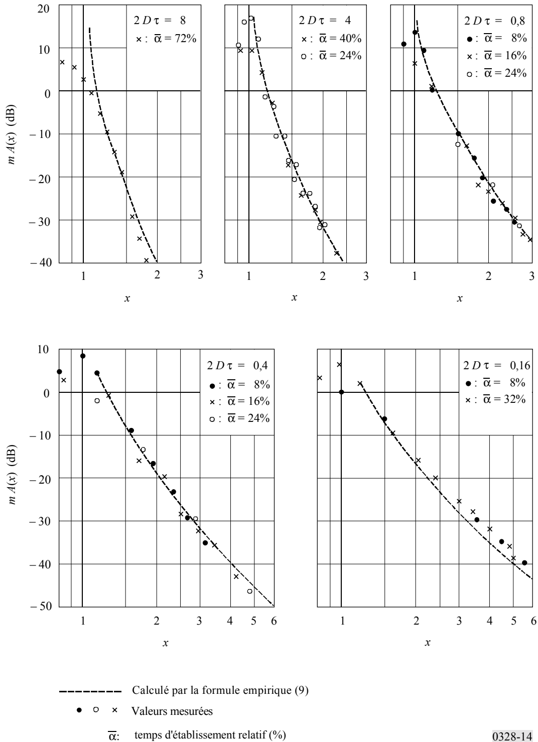
FIGURE 14 Spectre des émissions de classe F1B
