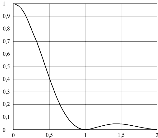
Spectre correspondant à la modulation MDP-2
