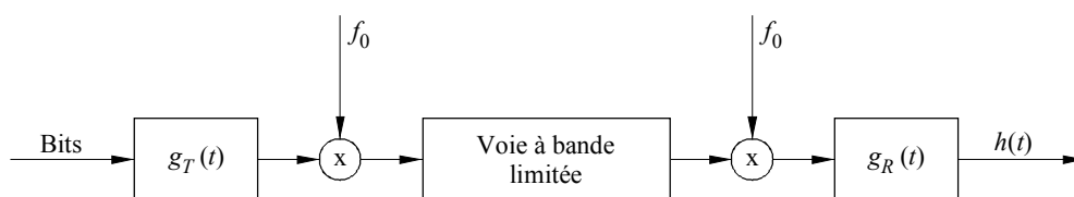
Emission sur une voie à bande limitée
