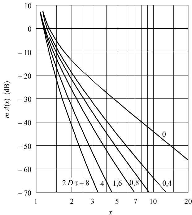
FIGURE 13 Distribution spectrale des émissions de classe F1B calculée par la formule empirique (9)
