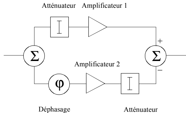
FIGURE 45 Prédistorsion à limiteur souple
