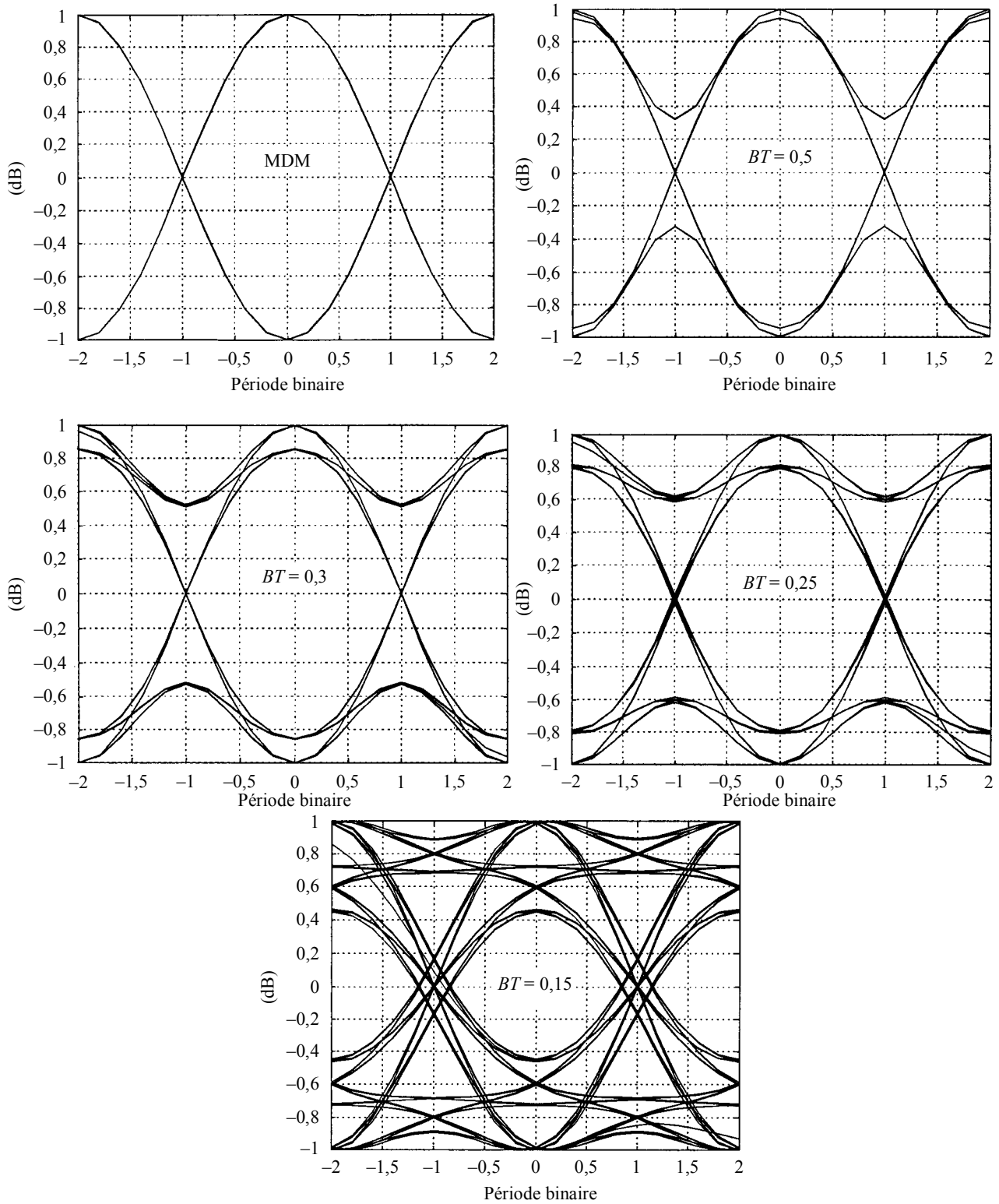
FIGURE 33 Diagrammes en oeil
