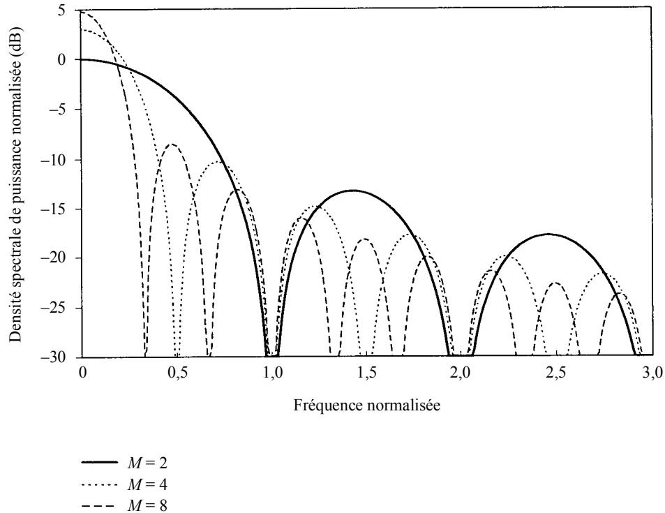
Spectres correspondant aux modulations MDP-2, MDP-4 et MDP-8
