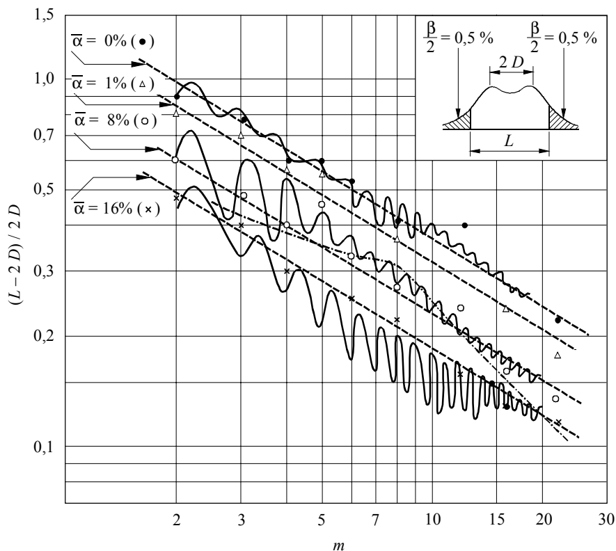
FIGURE 16 Comparaison entre les résultats des calculs et les mesures de la largeur de bande occupée
