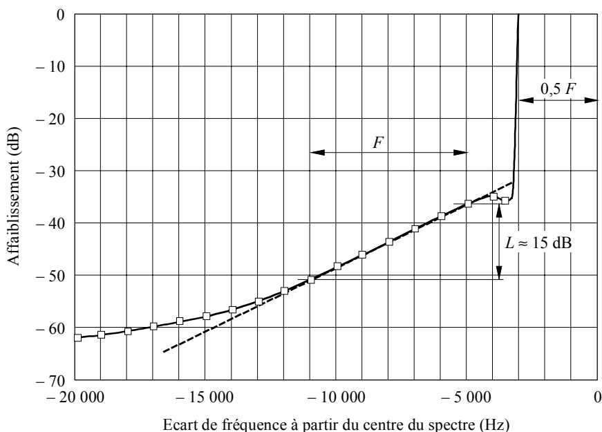
Courbe D de la Fig. 10 représentée sur une échelle de fréquence linéaire
