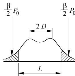
FIGURE 15 Largeur de bande calculée par la formule empirique (10)
