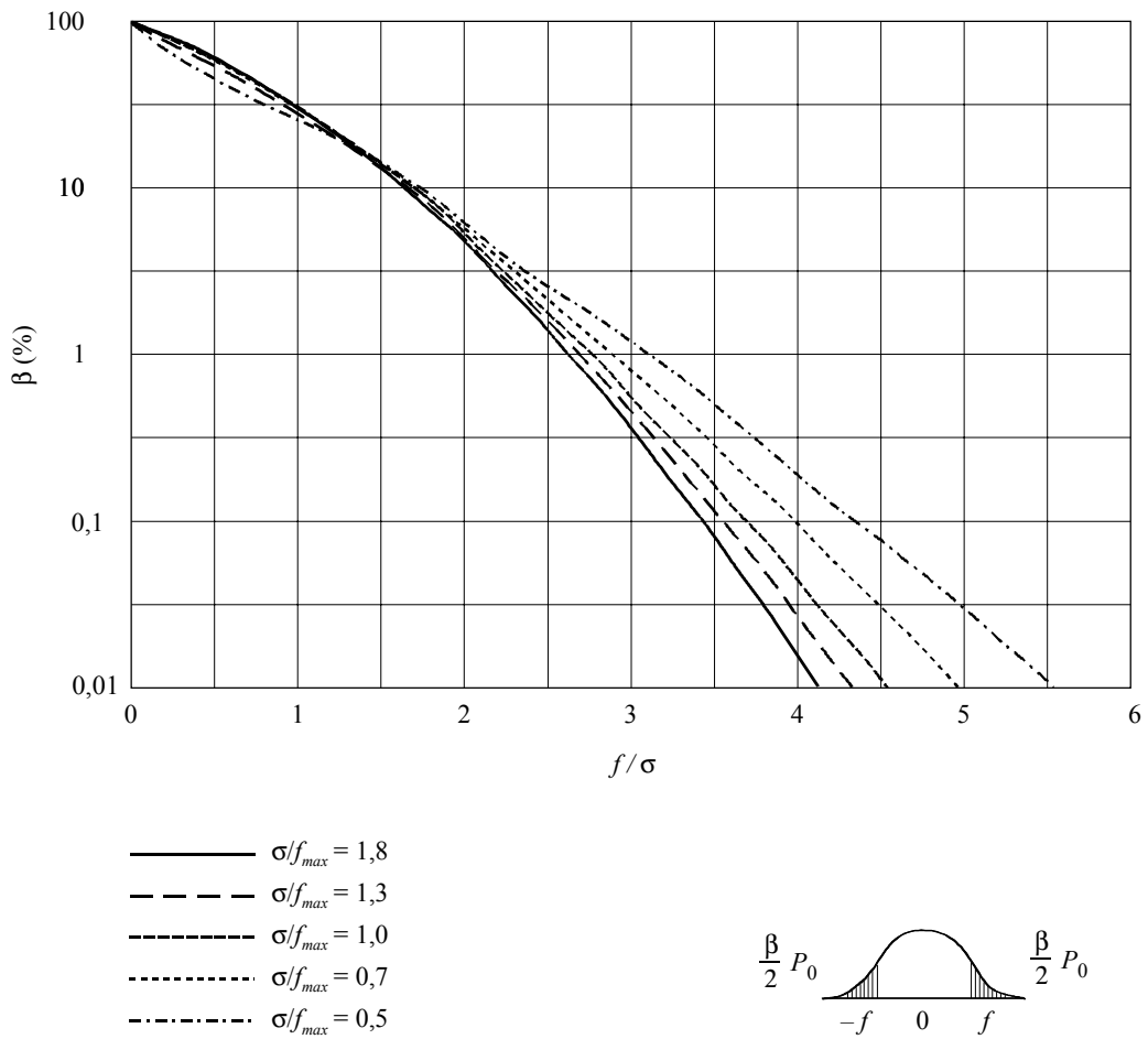
FIGURE 19 Puissance hors bande du spectre pour \sigma/f_{max} \geq 0,5
