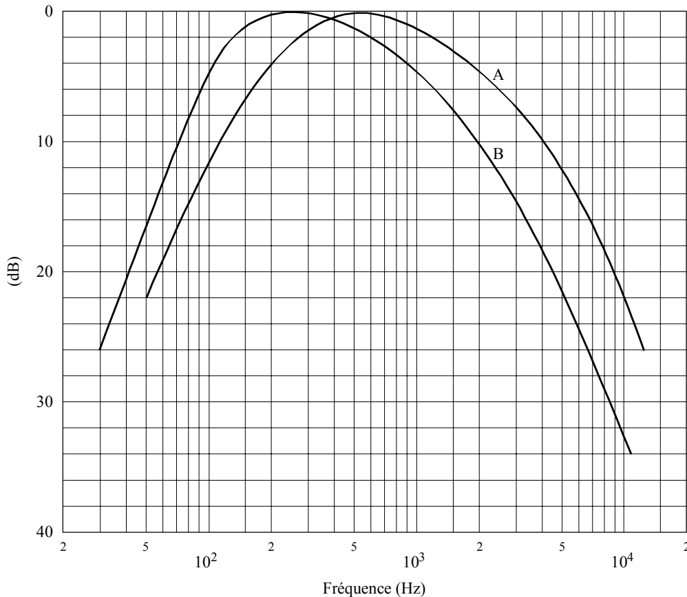
Courbes A: spectre du bruit normalisé (mesuré à l'aide d'un filtre «tiers d'octave») B: réponse en fréquence du filtre
