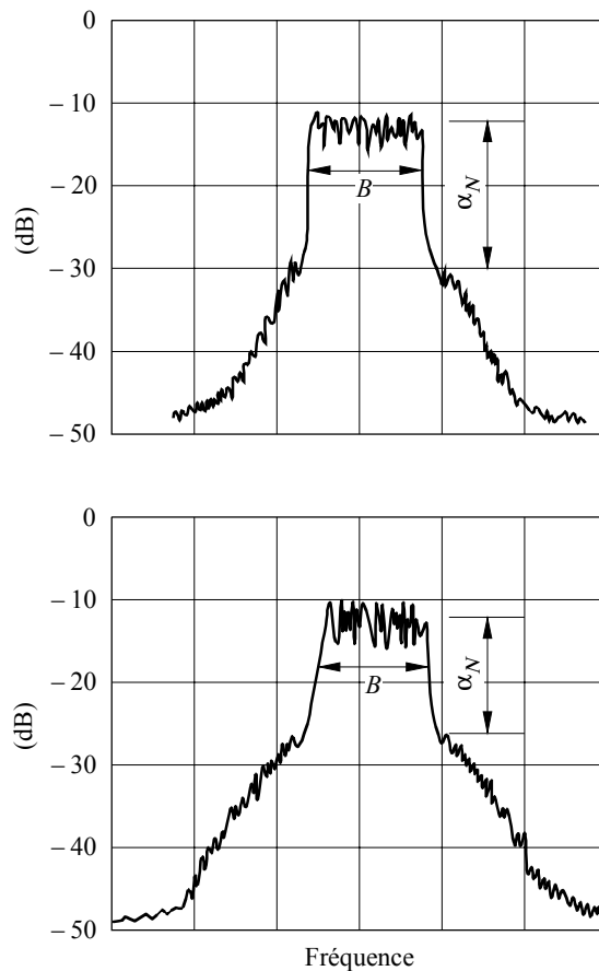
FIGURE 23 Enveloppe spectrale d'une émission de classe J3E modulée par du bruit blanc
