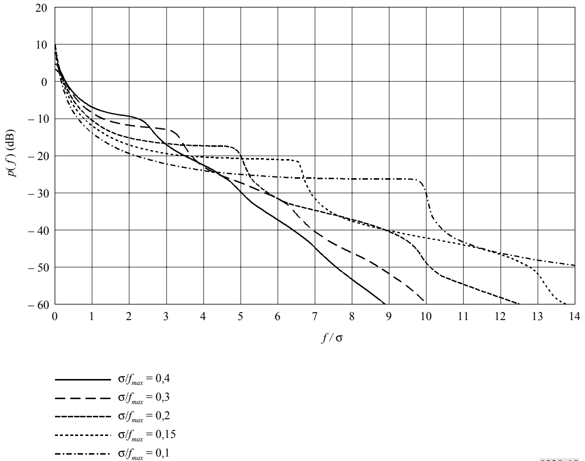
FIGURE 18 Distribution de la puissance du spectre pour \sigma/f_{max} < 0,5
