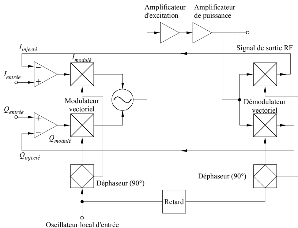
FIGURE 48 Technique à boucle cartésienne
