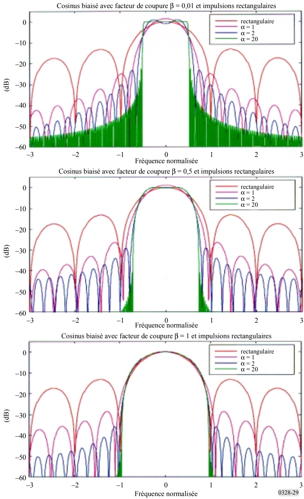
FIGURE 29 Spectres pour des facteurs de coupure = 0,01; 0,5 et 1
