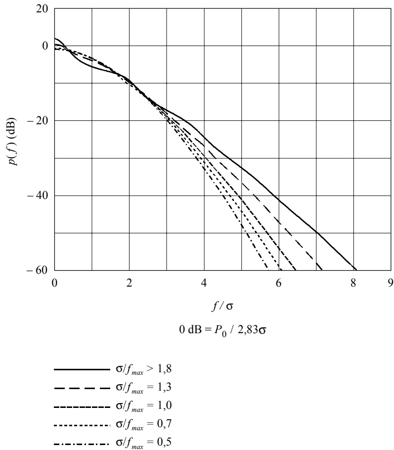
FIGURE 17 Distribution de la puissance du spectre pour \sigma/f_{max} \geq 0,5
