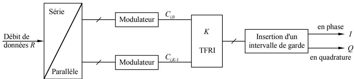
FIGURE 34 Emetteur MFO
