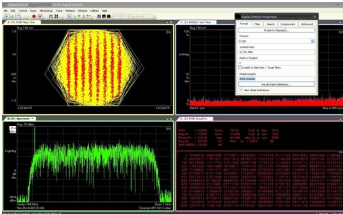
FIGURA 2 Presentación del VSA que ilustra una forma espectral característica
