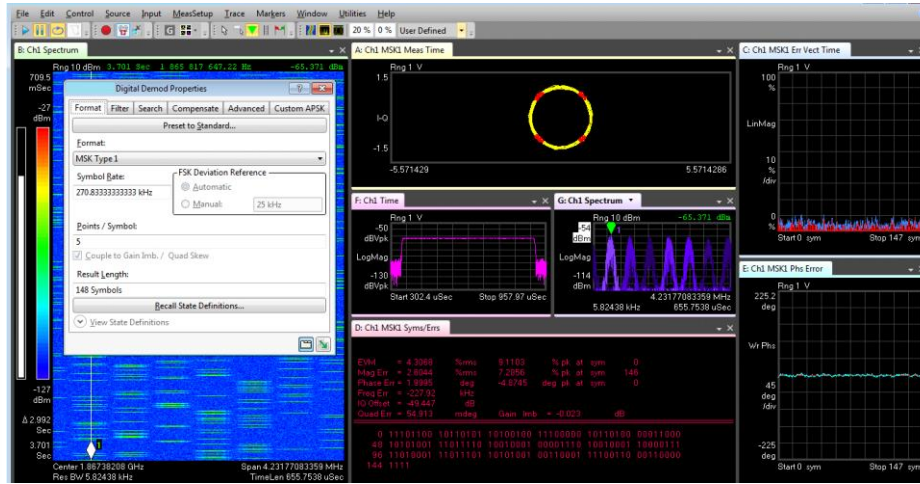
FIGURA 8 Resultados del análisis del enlace ascendente GSM
