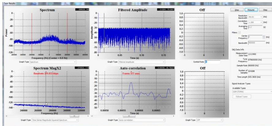
FIGURA 7 Resultados del análisis del enlace descendente GSM
