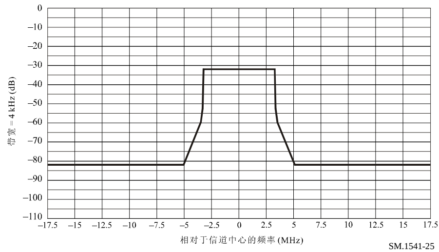
7 MHz ISDB-T的频谱限制掩模 ( P > 39 dBW)
