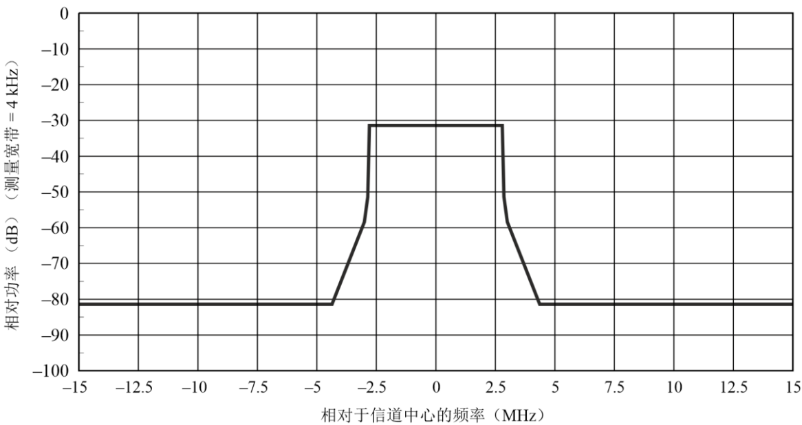
用于6 MHz信道配置系统D（DTMB）的频谱限制掩模
