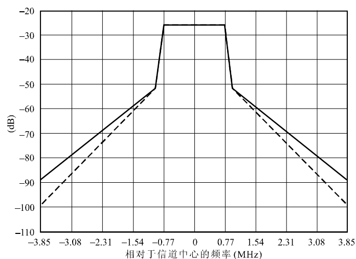
数字系统A的频谱限制掩模 ( 9 \text{ dBW} < P \leq 29 \text{ dBW} )
