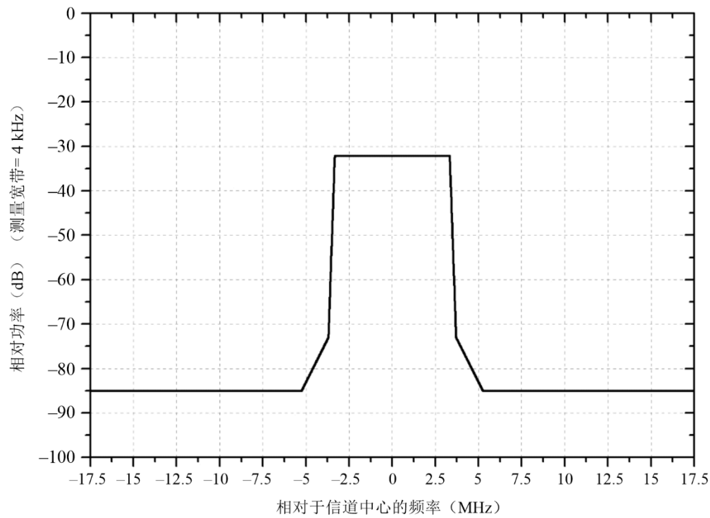
7 MHz DTMB的频谱限值掩膜
