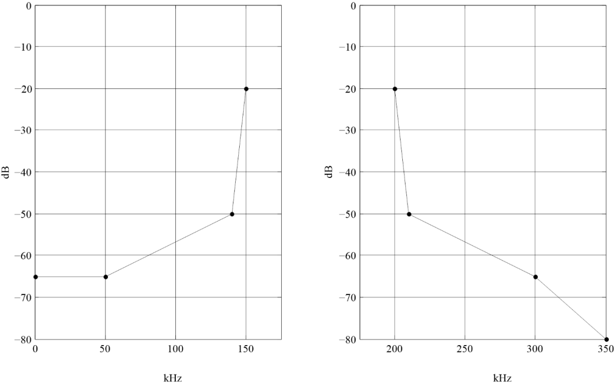
图34 频谱模式C的频谱掩模
