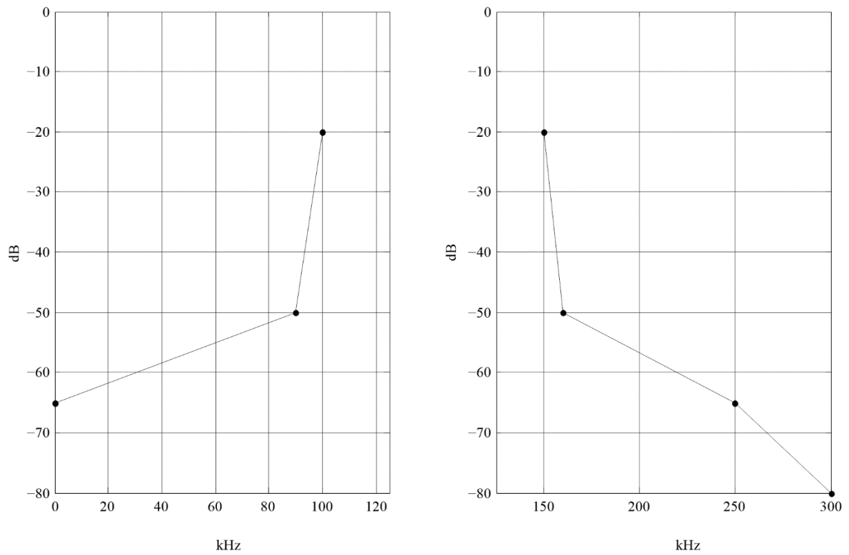
频谱模式E的频谱掩模
