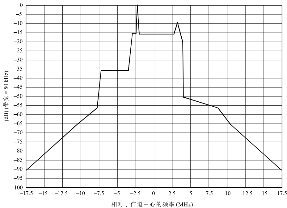
7 MHz模拟电视、0.75 MHz VSB负调制 ( P=39\text{ dBW} 至 50\text{ dBW} )
