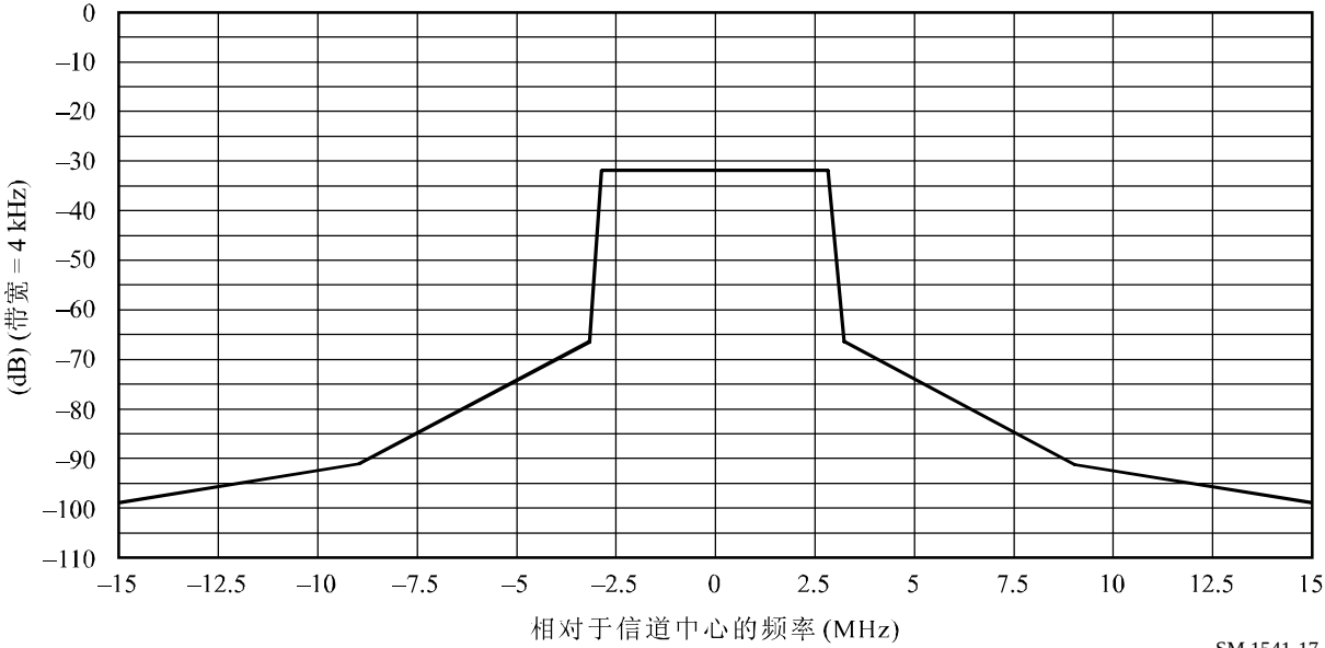
6 MHz DVB-T频谱限制掩模（ P=39\text{ dBW} 至 50\text{ dBW} ）
