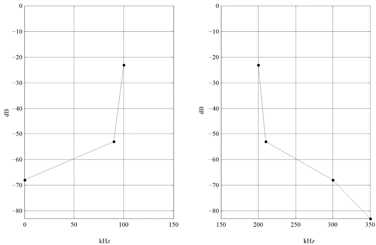
图37 频谱模式F的频谱掩模
