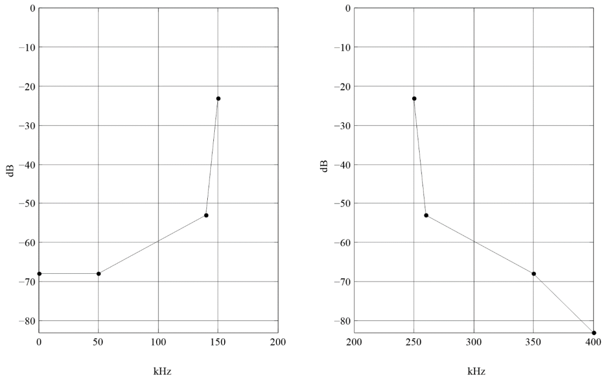
频谱模式D的频谱掩模
