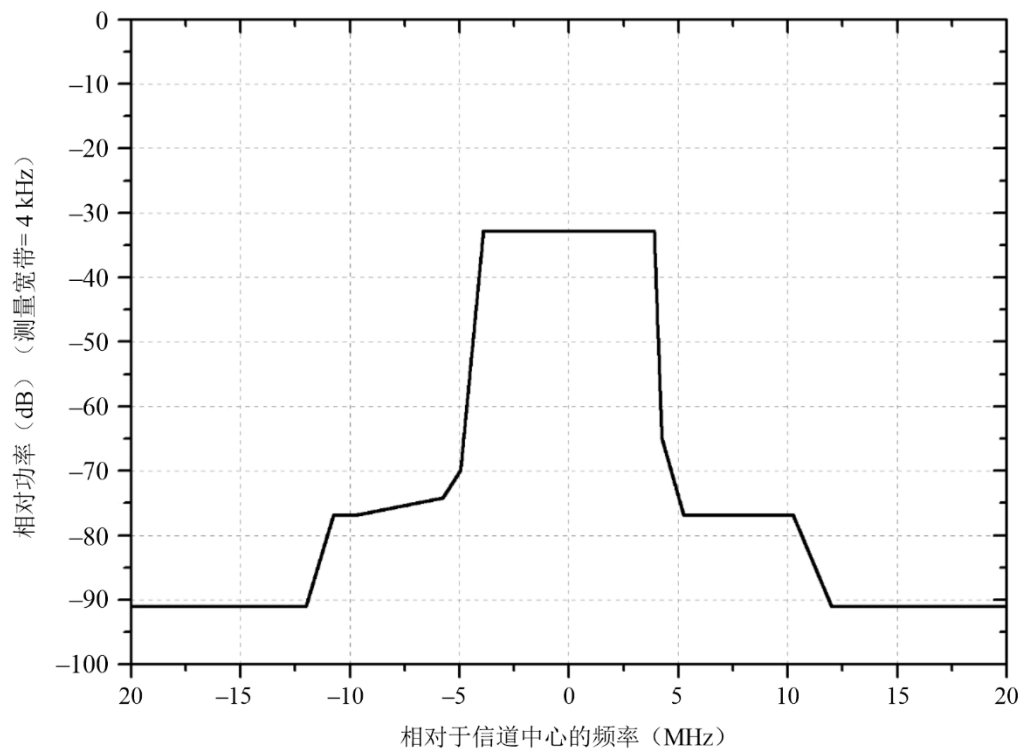
8 MHz DTMB的频谱限值掩膜
