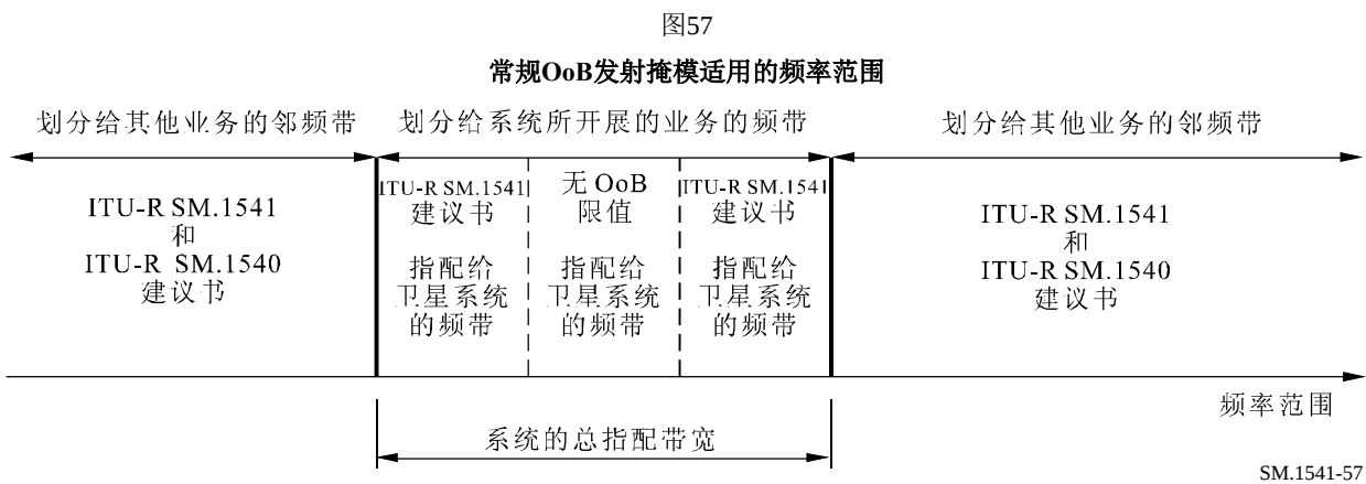
图57注 – 有关OoB域发射的本建议书适用范围为从总指配频段的端点直到杂散域的起始点。
