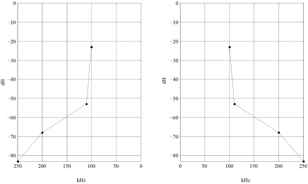
图33 频谱模式B的频谱掩模
