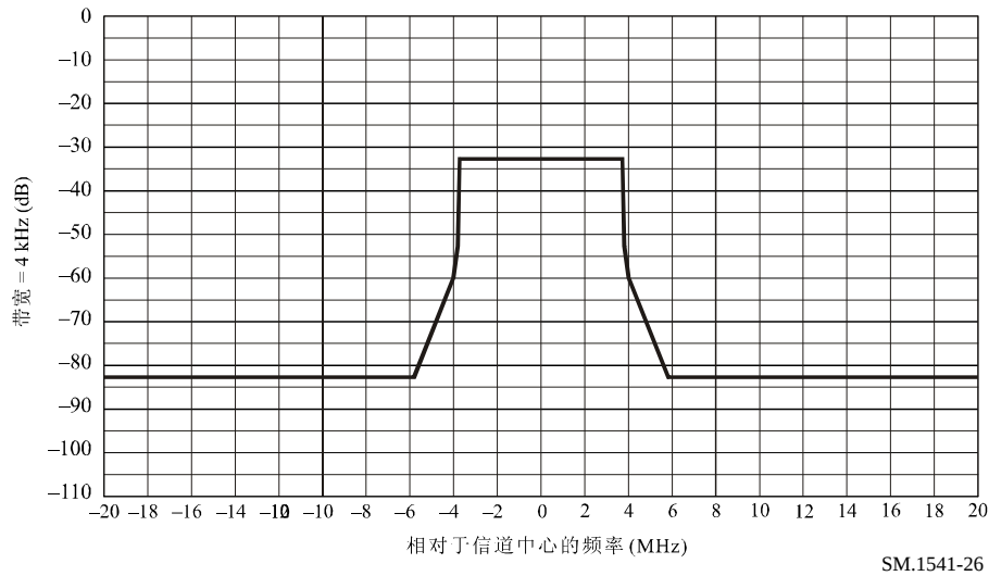
8 MHz ISDB-T的频谱限制掩模（ P>39\text{ dBW} ）
