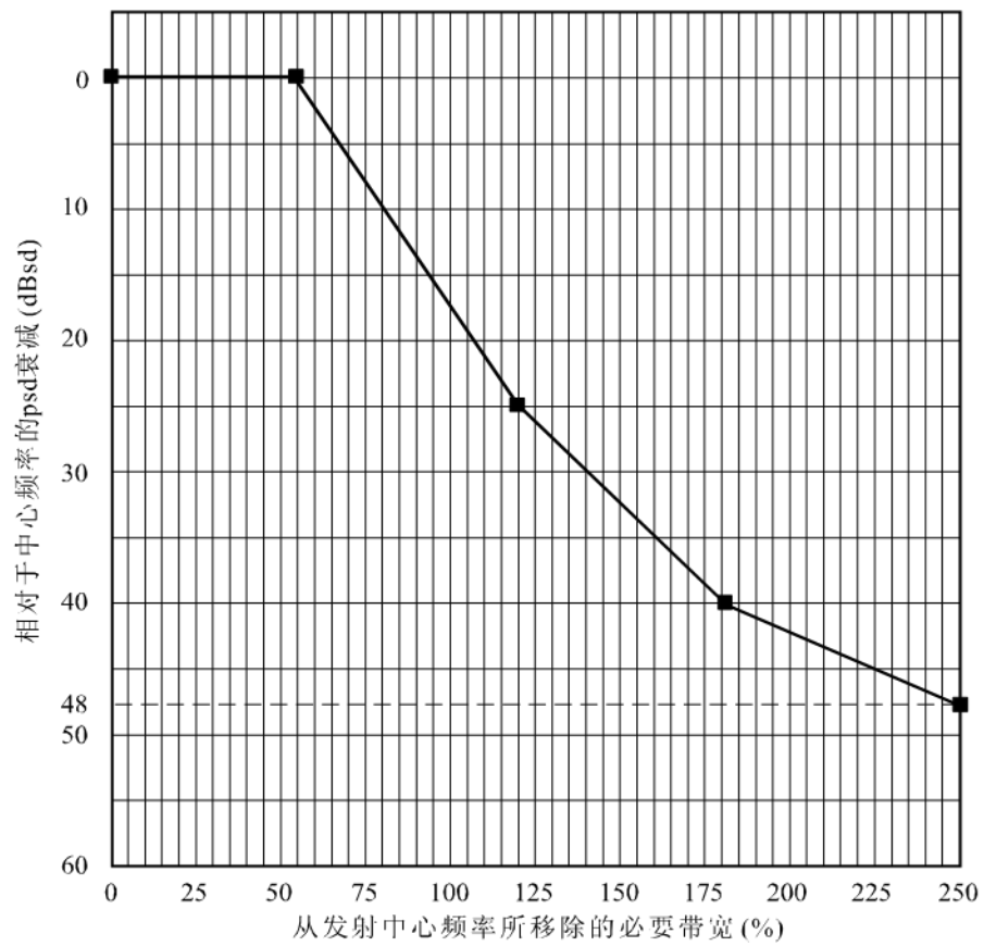
30 MHz以下固定数字业务的常规频谱掩模 (见表38)
