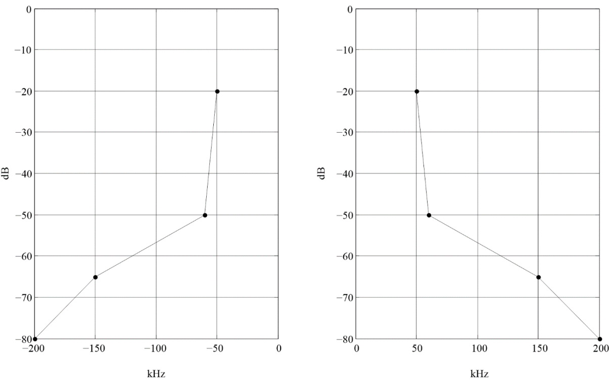
图32 频谱模式A的频谱掩模
