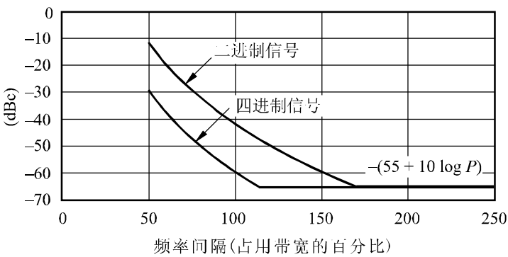
图49 航空遥测带外发射掩模的示例
