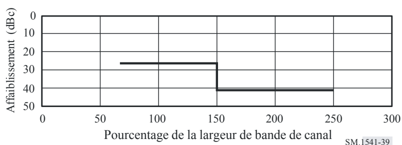
Gabarit des émissions hors bande pour les systèmes cellulaires analogiques à largeur de bande de canal de 30 kHz
