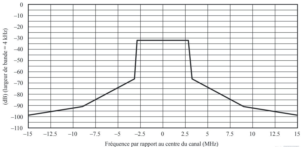
Gabarit de limite spectrale pour les systèmes DVB-T à 6 MHz (pour P compris entre 39 et 50 dBW)
