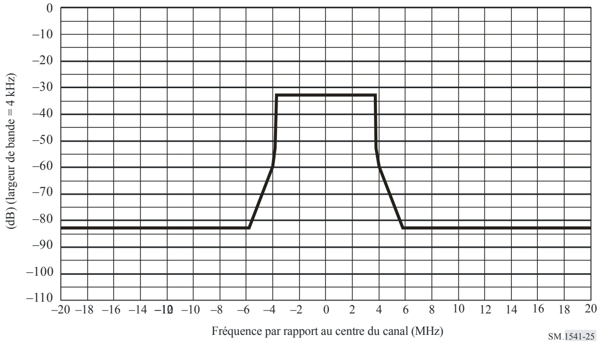
Gabarit de limite spectrale pour les systèmes ISDB-T à 8 MHz (pour P > 39 dBW)
