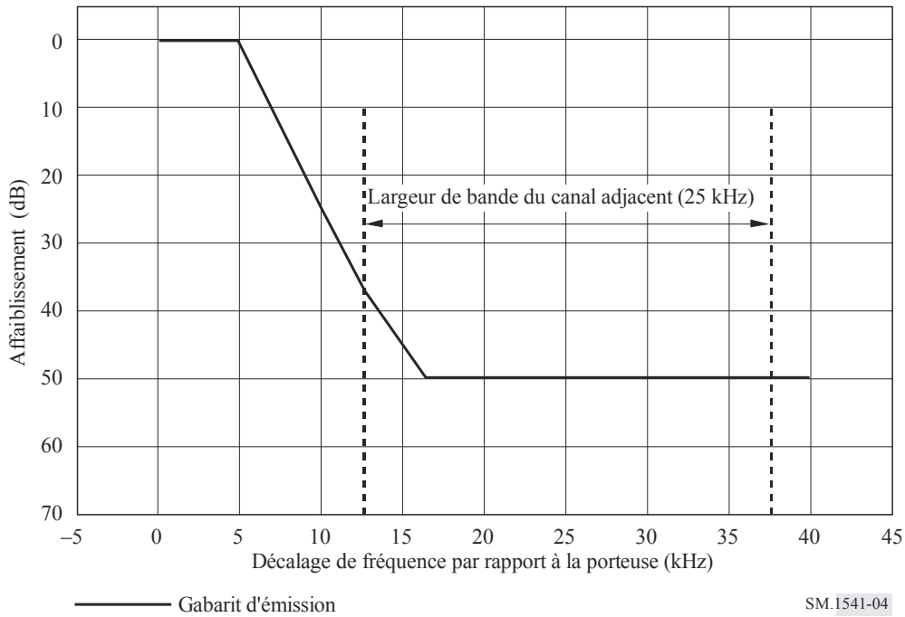
Gabarit d'émission G (sur la base d'une RBW de 300 Hz)
