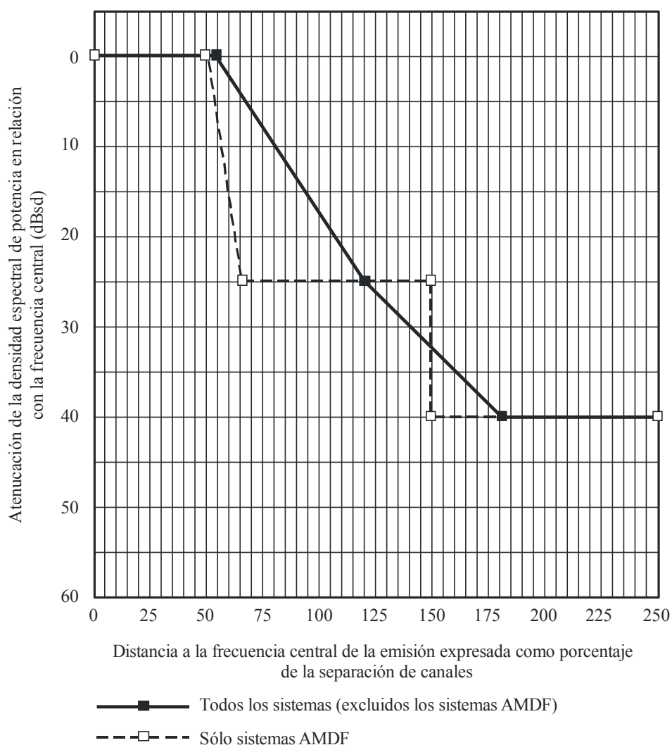
FIGURA 44 Máscaras espectrales genéricas para el servicio fijo digital por encima de 30 MHz (véase el Cuadro 28)
