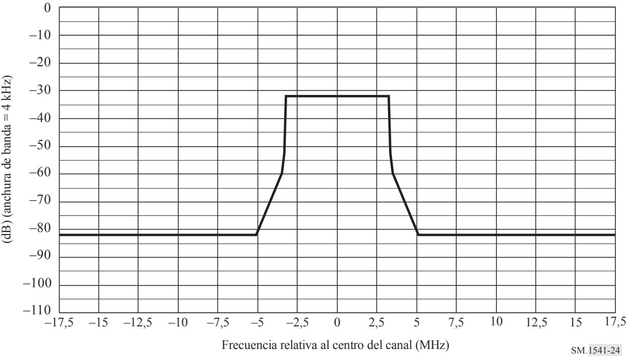
FIGURA 24 Máscara de límites espectrales para los sistemas ISDB-T de 7 MHz (para P > 39 dBW)
