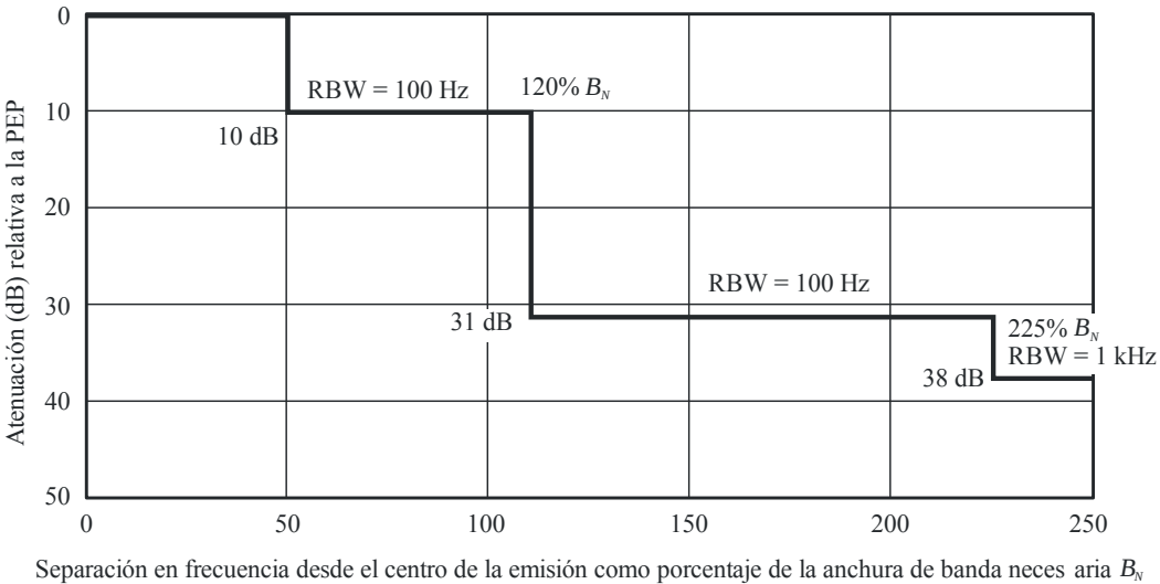
FIGURA 34 Estaciones que funcionan a frecuencias inferiores a 30 MHz en los casos normales o de banda estrecha de la Recomendación UIT-R SM.1539
