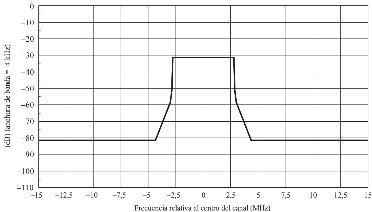
FIGURA 18 Máscara de límites espectrales para sistemas ISDB-T de 6 MHz (para P > 39 dBW)
