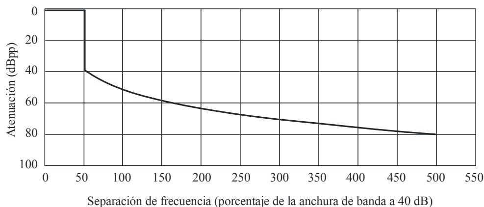
Objetivo de diseño para futuros sistemas de radar
