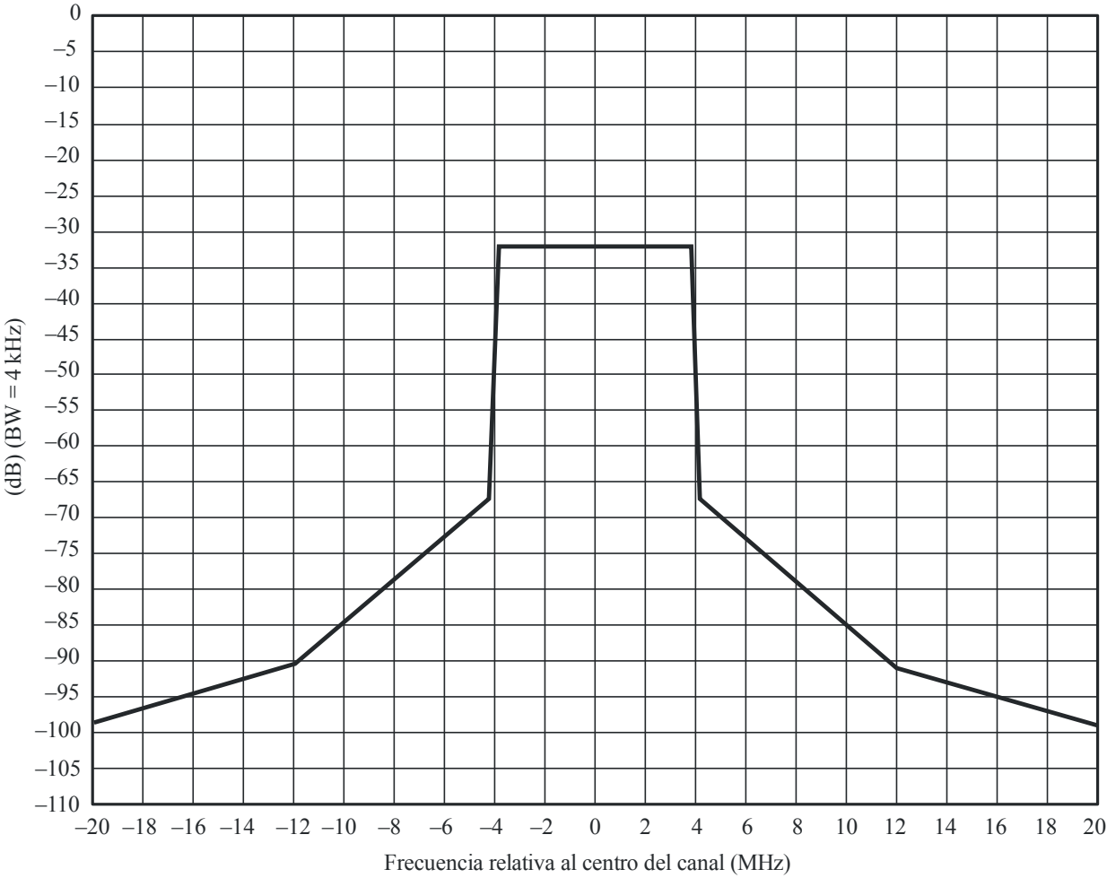
FIGURA 23 Máscara del límite espectral para los sistemas DVB-T de 8 MHz (para P = 39 a 50 dBW)
