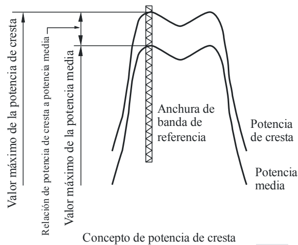
FIGURA 2 Referencia de 0 dBpp, valor máximo de la potencia de cresta
