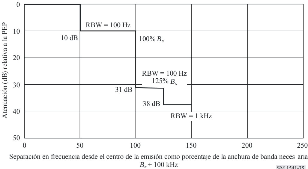
FIGURA 35 Estaciones que funcionan a frecuencias inferiores a 30 MHz en el caso de banda ancha de la Recomendación UIT-R SM.1539
