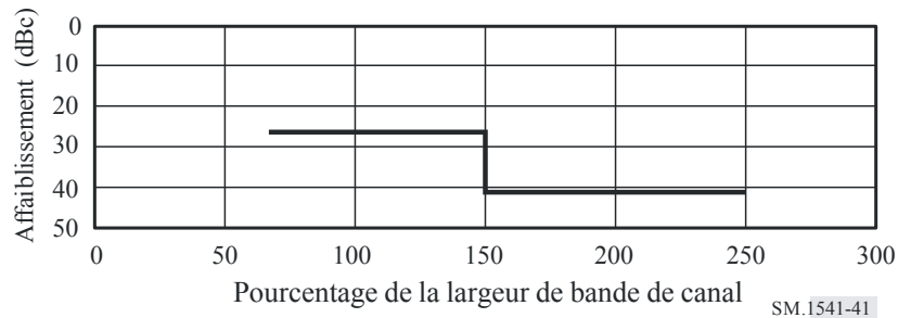
Gabarit des émissions hors bande pour les systèmes cellulaires analogiques à largeur de bande de canal de 30 kHz
