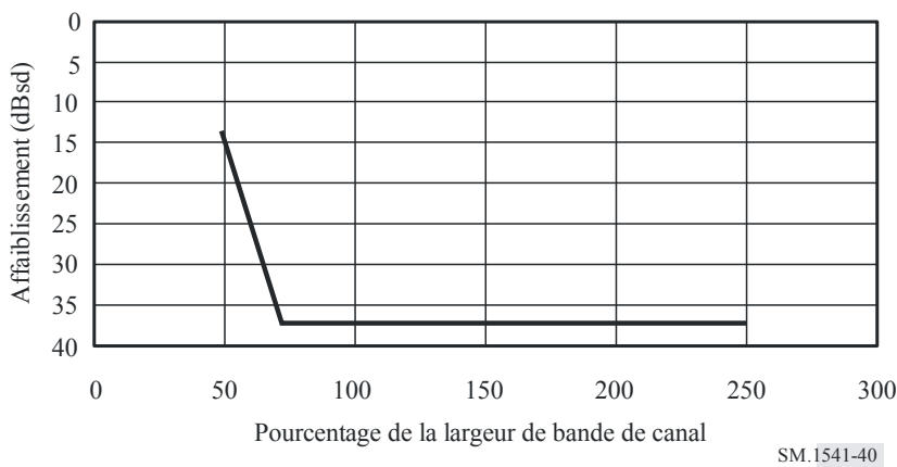
Gabarit des émissions hors bande pour les systèmes mobiles terrestres à largeur de bande de canal de 6,5 kHz
