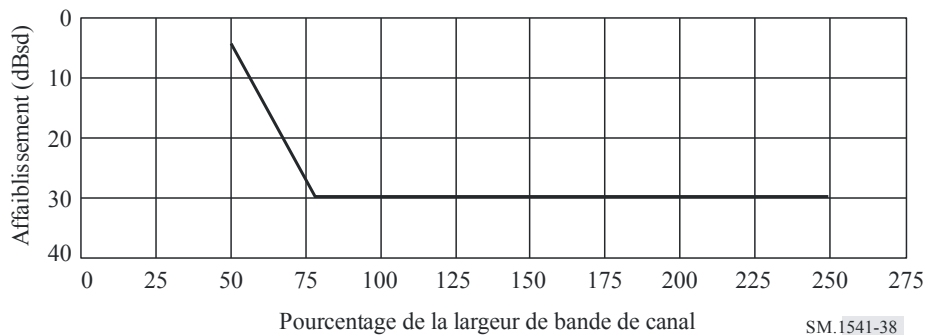
Gabarit des émissions hors bande pour les systèmes mobiles terrestres à largeur de bande de canal de 12,5 kHz
