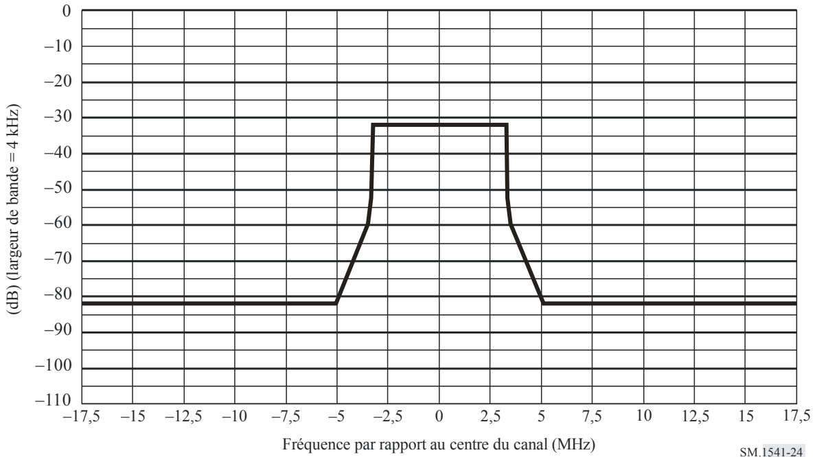
Gabarit de limite spectrale pour les systèmes ISDB-T à 7 MHz (pour P > 39 dBW)
