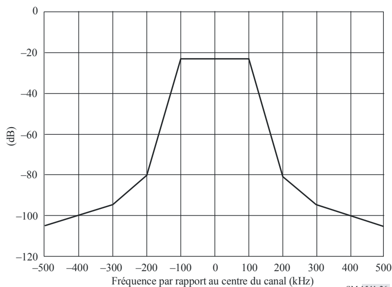
Gabarit de limite spectrale pour les émetteurs de radiodiffusion sonore à modulation de fréquence en ondes métriques (proposition initiale) (Canaux de 200 kHz)
