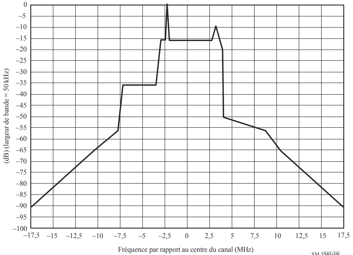
Gabarit de limite spectrale pour la télévision analogique à 7 MHz, modulation négative, BLR de 0,75 MHz (pour P = 39 à 50 dBW)
