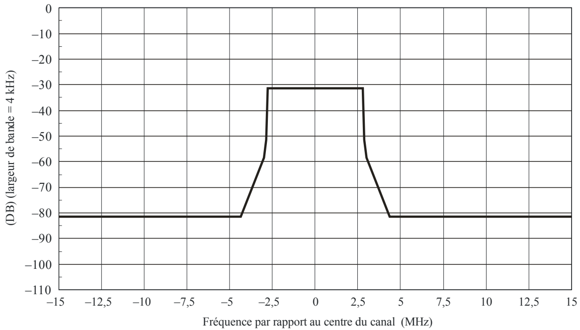
Gabarit de limite spectrale pour les systèmes ISDB-T à 6 MHz (pour P < 39 dBW)
