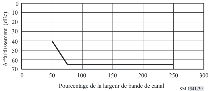
Gabarit des émissions hors bande pour les systèmes à BLU avec compression-extension d'amplitude et à largeur de bande de canal de 5 kHz
