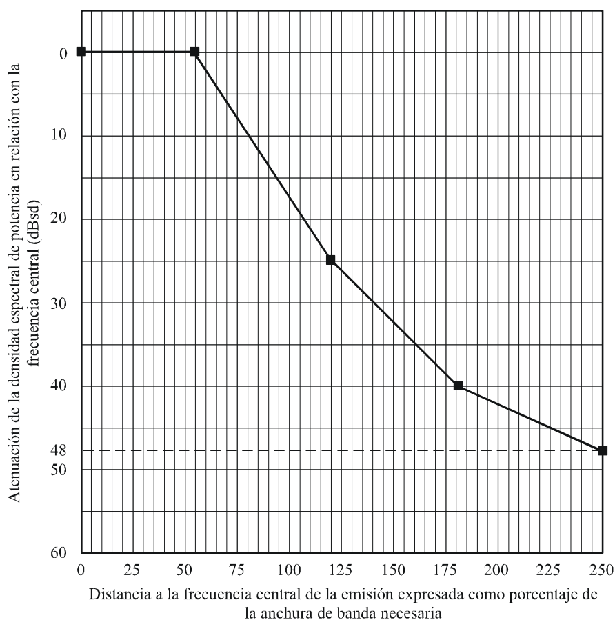
FIGURA 46 Máscaras espectrales genéricas del servicio fijo digital por debajo de 30 MHz (Véase el Cuadro 29)
