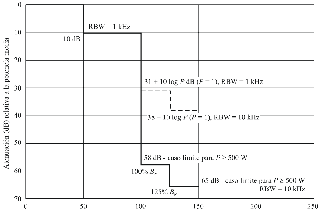
FIGURA 38 Estaciones que funcionan por encima de 30 MHz en el caso de banda ancha de la Recomendación UIT-R SM.1539
