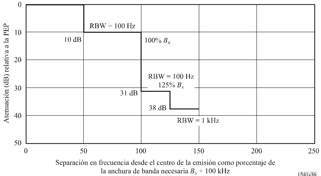
FIGURA 36 Estaciones que funcionan a frecuencias inferiores a 30 MHz en el caso de banda ancha de la Recomendación UIT-R SM.1539
