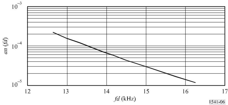
FIGURA 6 Distribución de la potencia de emisión en el lado cercano de la banda adyacente
