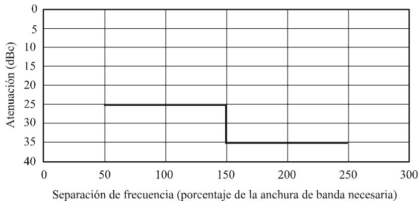
FIGURA 44 Máscara fuera de banda para servicios móviles aeronáuticos y móviles marítimos
