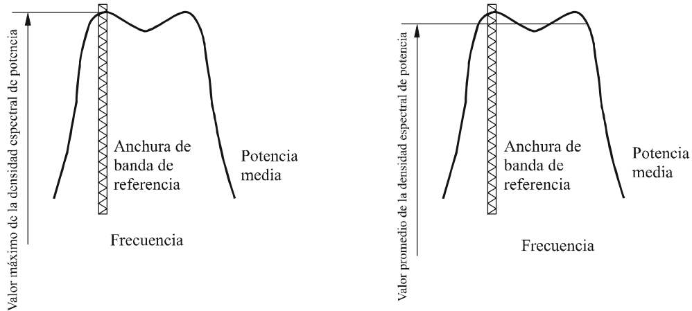
a) Concepto de densidad espectral de potencia máxima b) Concepto de densidad espectral de potencia promedio
