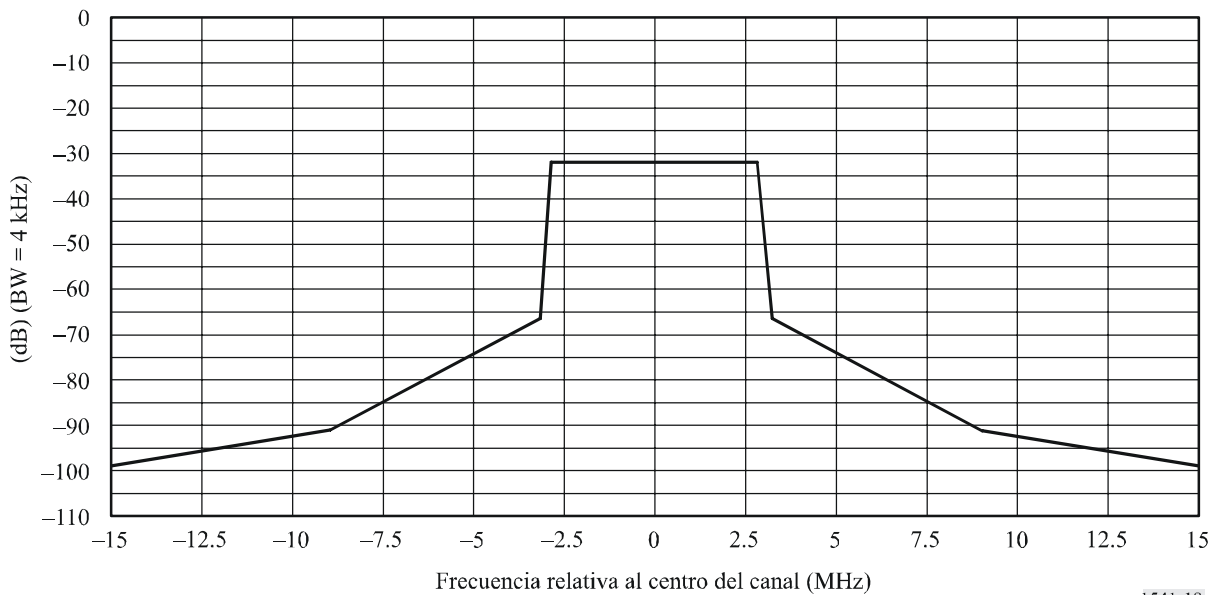
Contorno del límite espectral para la DVB-T de 6 MHz ( P = 39 a 50 dBW)
