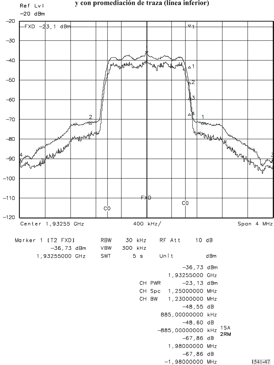
FIGURA 47 Espectro del enlace ascendente de acceso múltiple por división de código (IS95) medido con la función de medición de potencia media verdadera (línea superior) y con promediación de traza (línea inferior)
