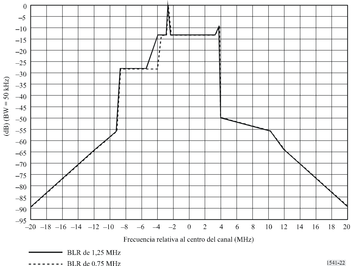
Máscara del límite espectral para la televisión analógica de 8 MHz, modulación positiva (para P = 39 a 50 dBW)
