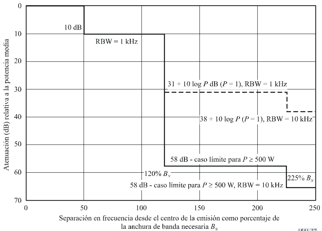
FIGURA 37 Estaciones que funcionan a frecuencias superiores a 30 MHz en los casos normales o de banda estrecha de la Recomendación UIT-R SM.1539
