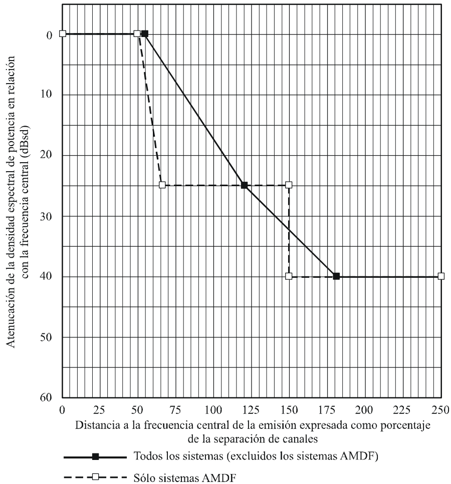
FIGURA 45 Máscaras espectrales genéricas para el servicio fijo digital por encima de 30 MHz (véase el Cuadro 28)
