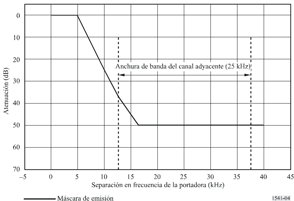
FIGURA 4 Máscara de emisión G (para una RBW de 300 Hz)
