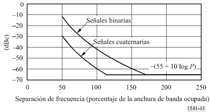
FIGURA 43 Ejemplos de máscaras fuera de banda para telemetría aeronáutica (5 Mbit/s a 10W)
