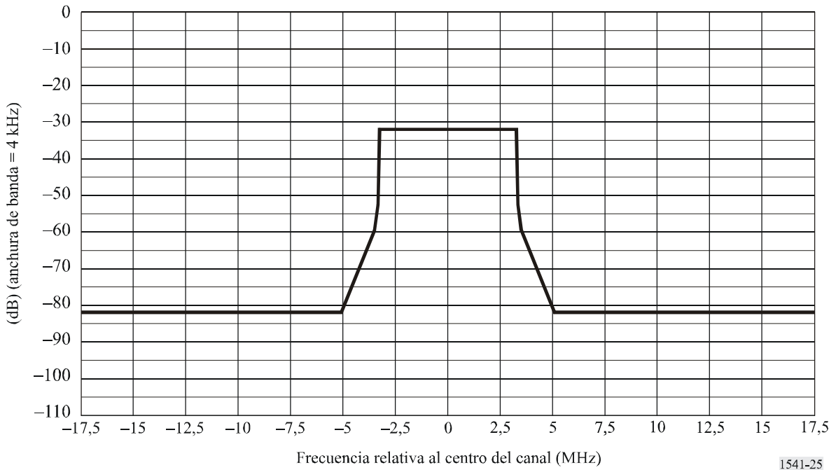
Máscara de límites espectrales para los sistemas ISDB-T de 7 MHz (para P > 39 dBW)
