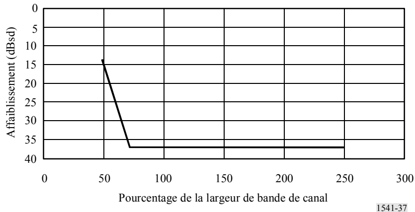
FIGURE 37 Gabarit des émissions hors bande pour les systèmes mobiles terrestres à largeur de bande de canal de 6,5 kHz
