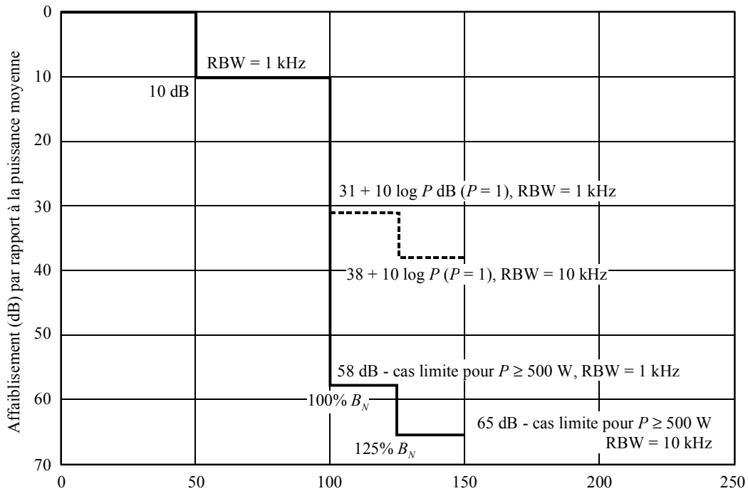
FIGURE 34 Stations fonctionnant au-dessus de 30 MHz dans le cas à large bande de la Recommandation UIT-R SM.1539
