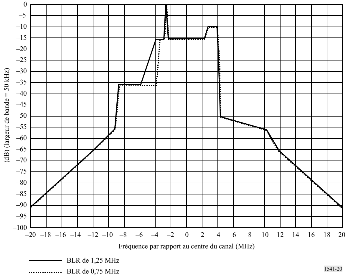
FIGURE 20 Gabarit de limite spectrale pour la télévision analogique à 8 MHz, modulation négative (pour P = 39 à 50 dBW)
