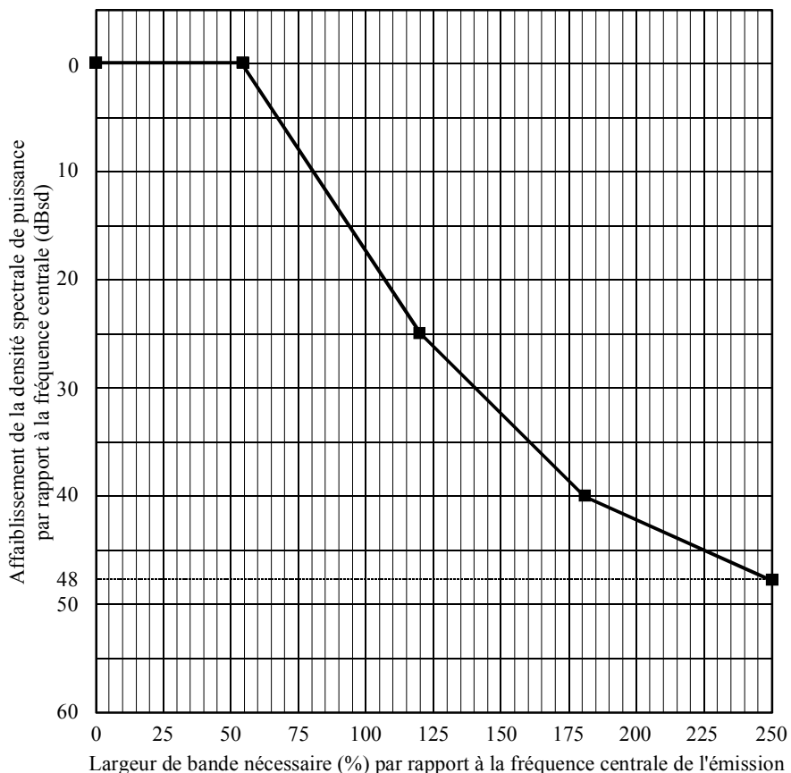
Gabarits spectraux génériques pour le service fixe numérique fonctionnant au-dessous de 30 MHz
