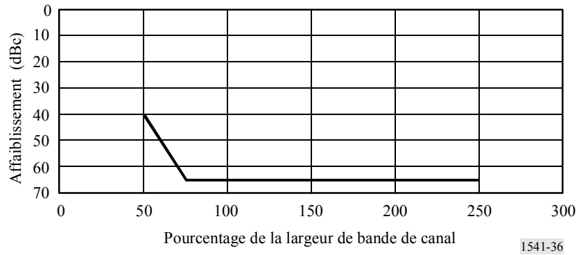
FIGURE 36 Gabarit des émissions hors bande pour les systèmes à BLU avec compression-extension d'amplitude et à largeur de bande de canal de 5 kHz
