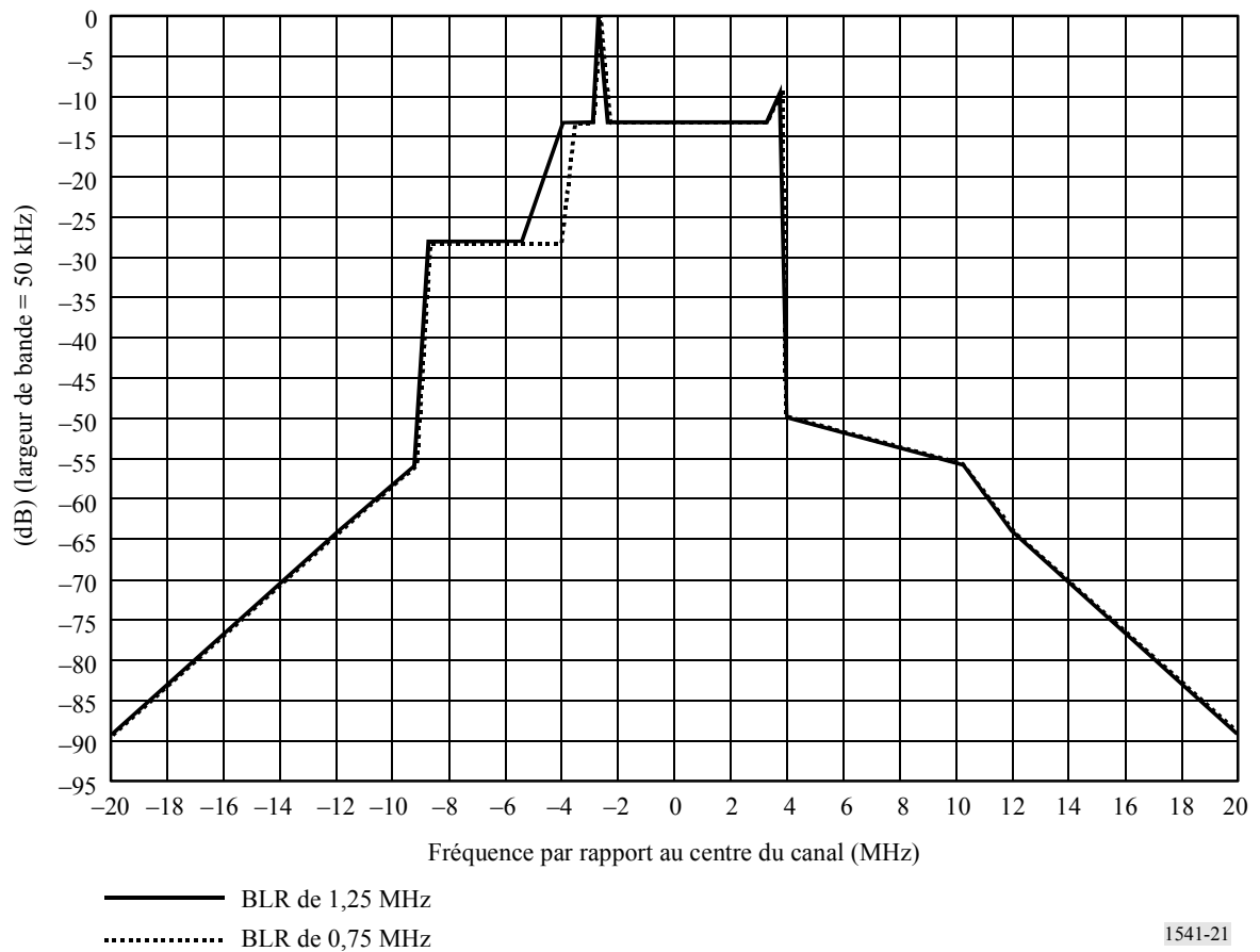
FIGURE 21 Gabarit de limite spectrale pour la télévision analogique à 8 MHz, modulation positive (pour P = 39 à 50 dBW)
