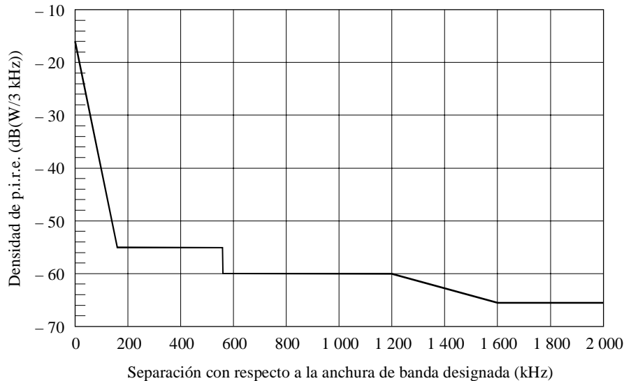
FIGURA 2 Norma del ETSI sobre emisiones no deseadas para terminales S-PCN
