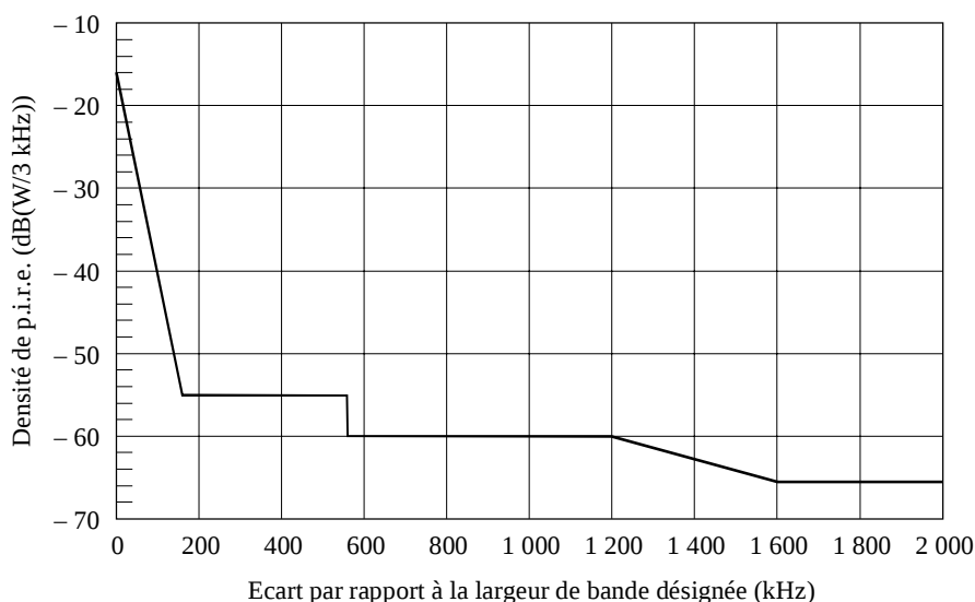
FIGURE 2 Gabarit normalisé par l'ETSI applicable aux rayonnements non désirés pour les stations S-PCN
