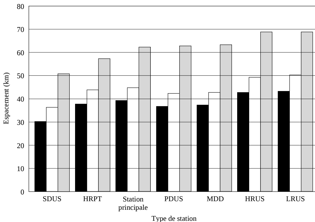
FIGURE 7 Plage d'espacements pour les stations du SMS utilisées dans des systèmes à satellites OSG
