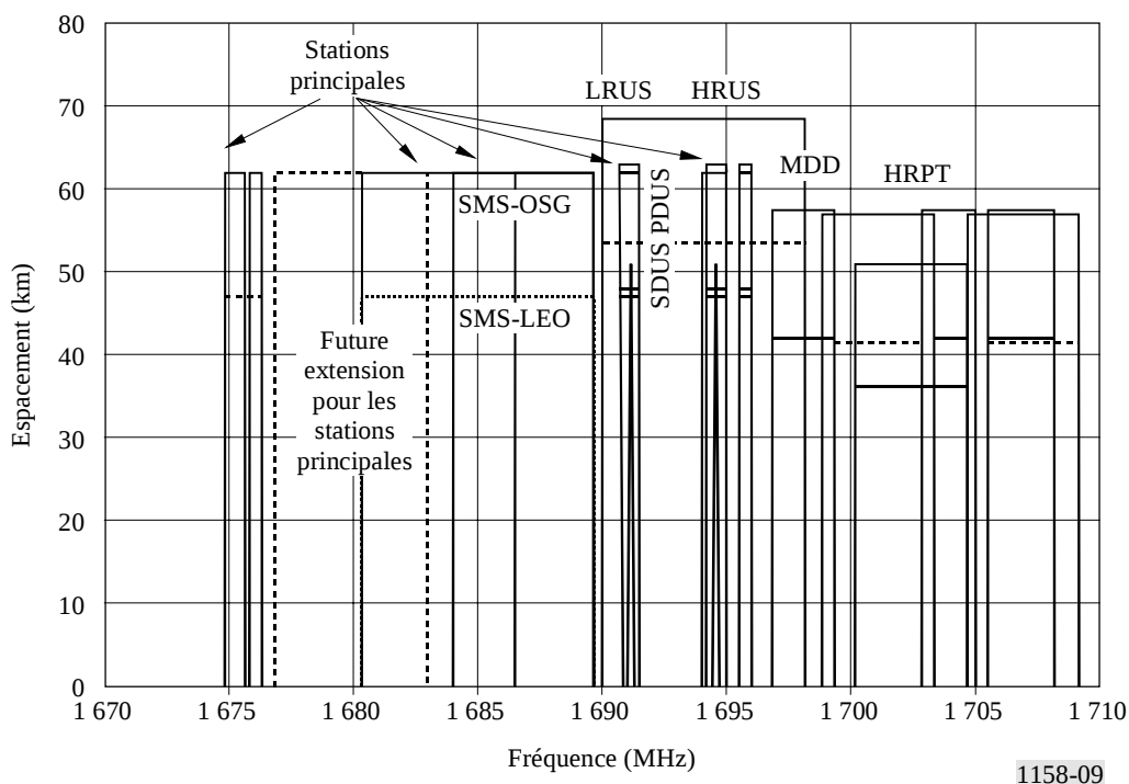
FIGURE 9 Largeurs de bande occupées par le service METSAT
