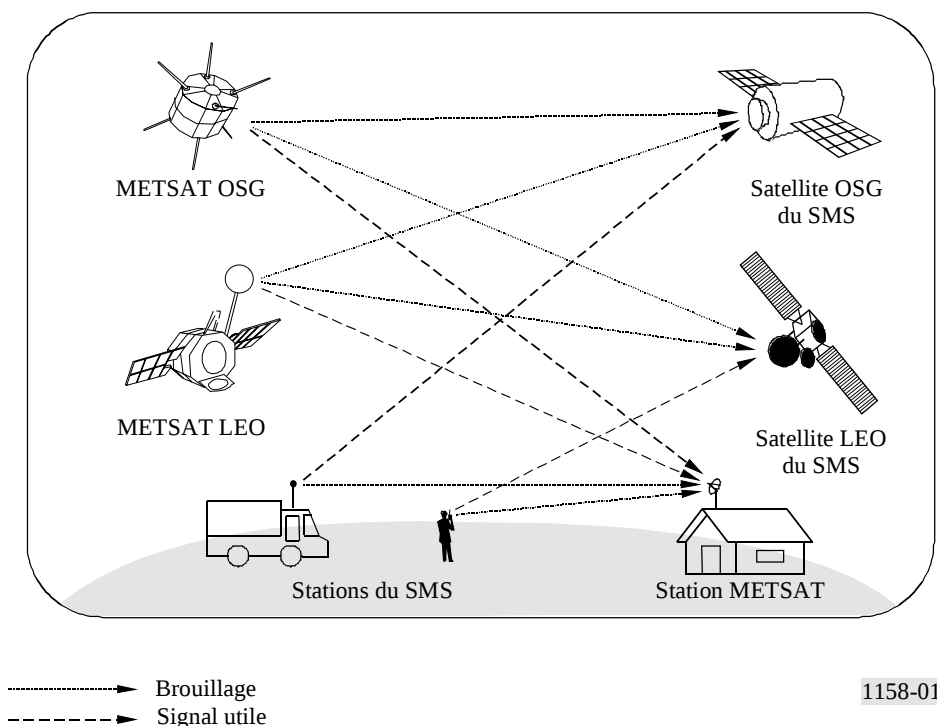
FIGURE 1 Configurations de brouillage examinées
