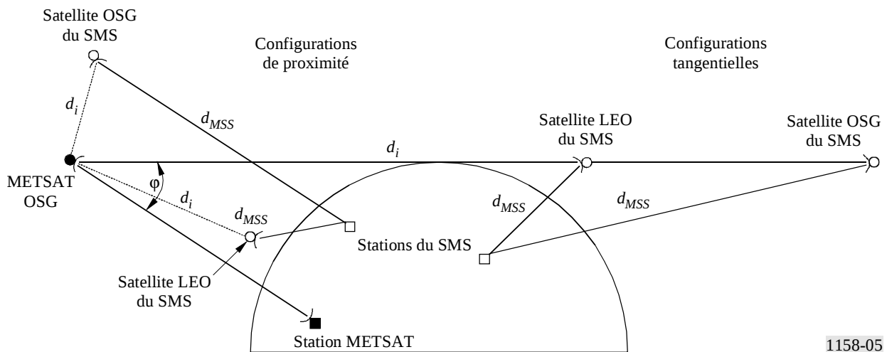
FIGURE 5 Configurations de brouillage entre un METSAT OSG et un MOBSAT
