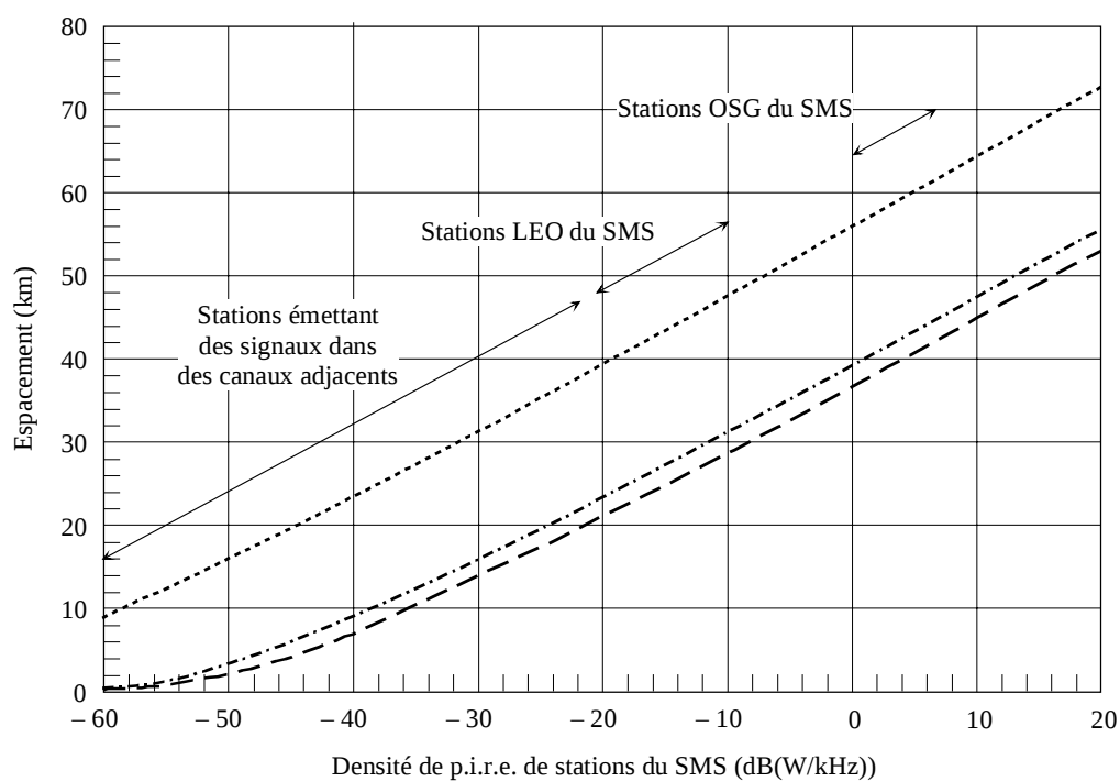
FIGURE 3 E spacements totaux pour des PDUS
