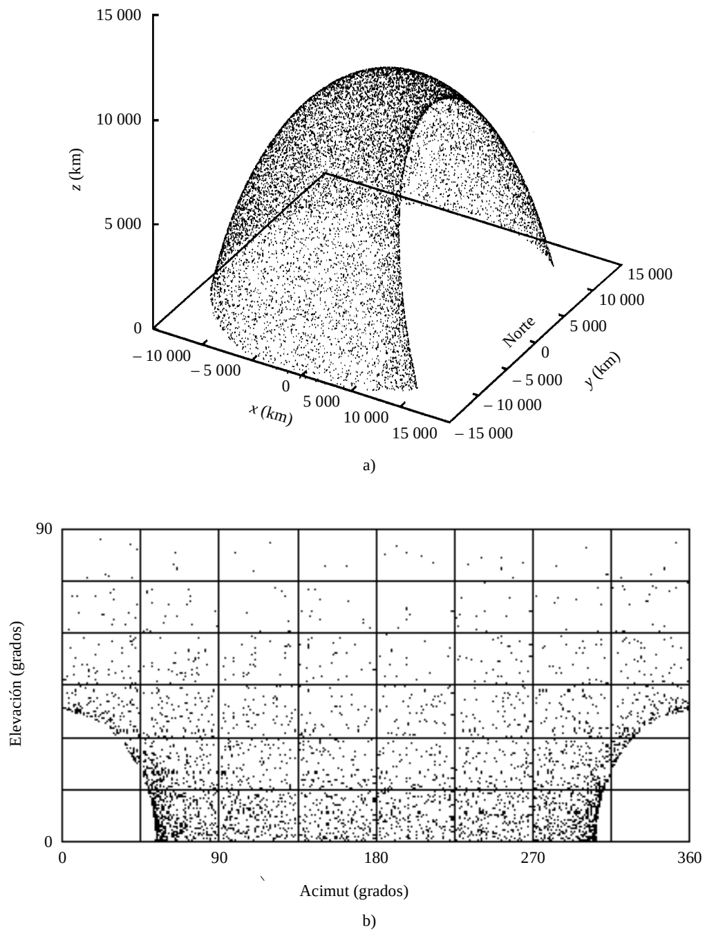
FIGURA 6 Dos coberturas celestes típicas para satélites no OSG
