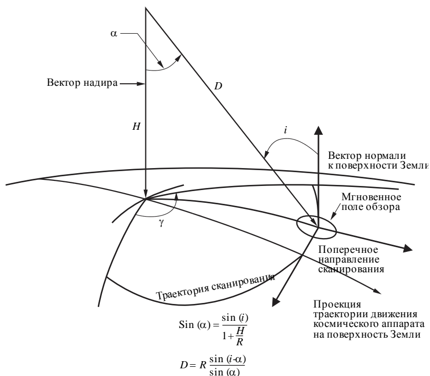
Типичная схема сканирования в рефлектометрах с коническим сканированием
