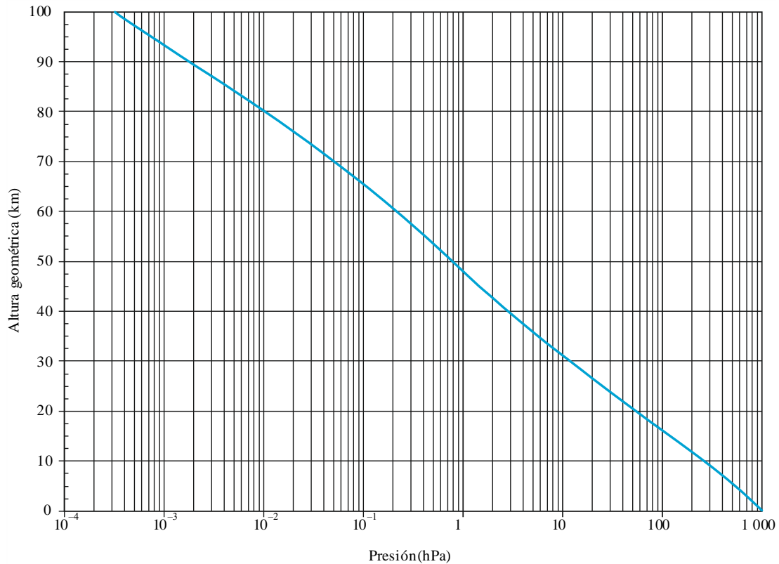
FIGURA 2 Presión en función de la altura geométrica
