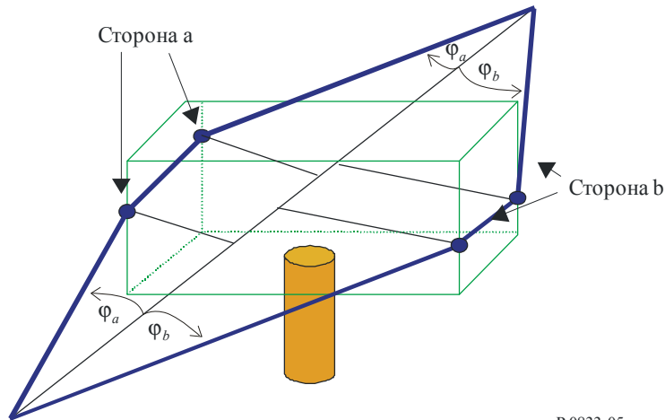
РИСУНОК 5 Составляющие, дифрагируемые вокруг растительного массива
