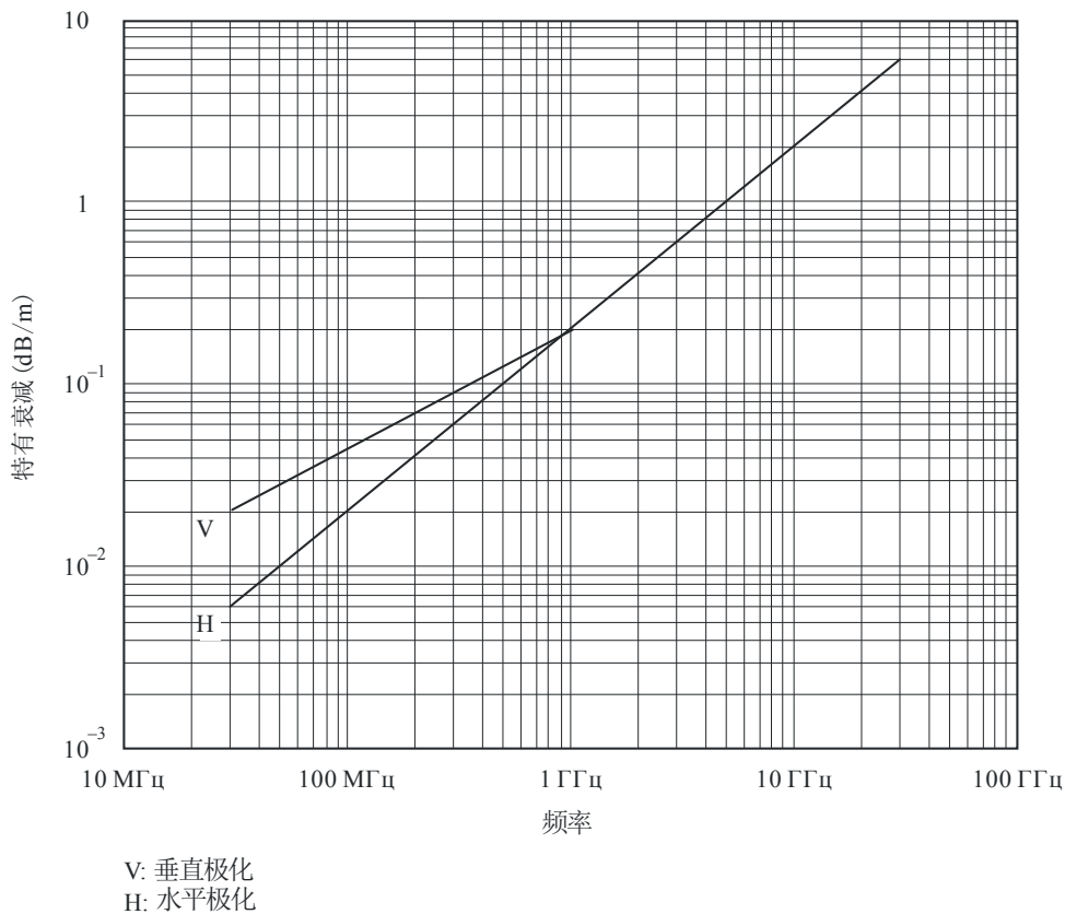
图2 林地造成的特有衰减
