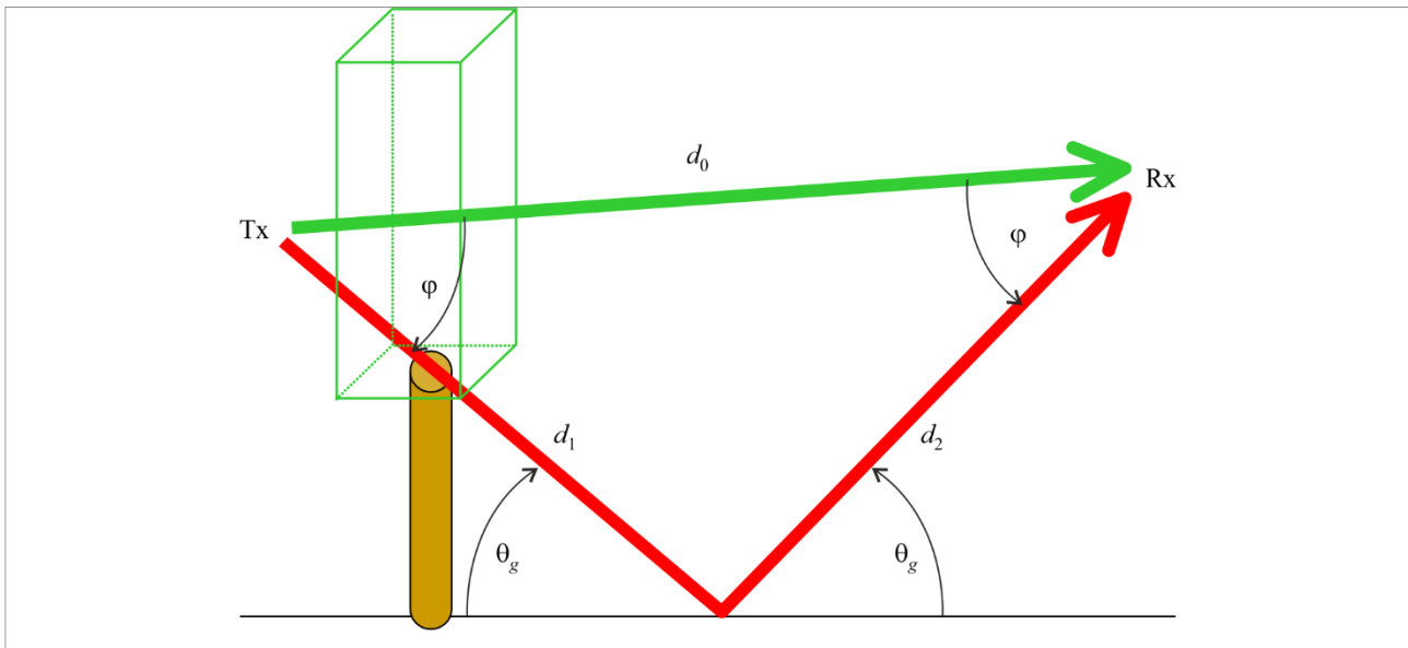
FIGURE 8 Composante réfléchi sur le sol
