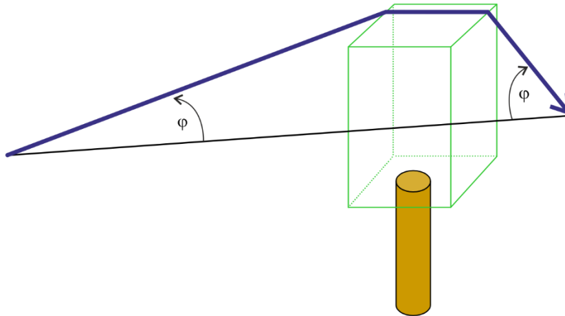
FIGURE 6 Composante de diffusion par diffraction sur la couverture végétale
