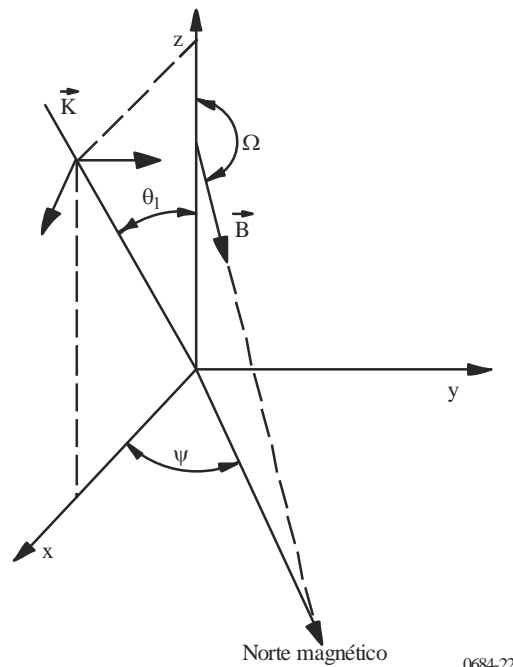
FIGURA 16 Geometría de propagación de las ondas
