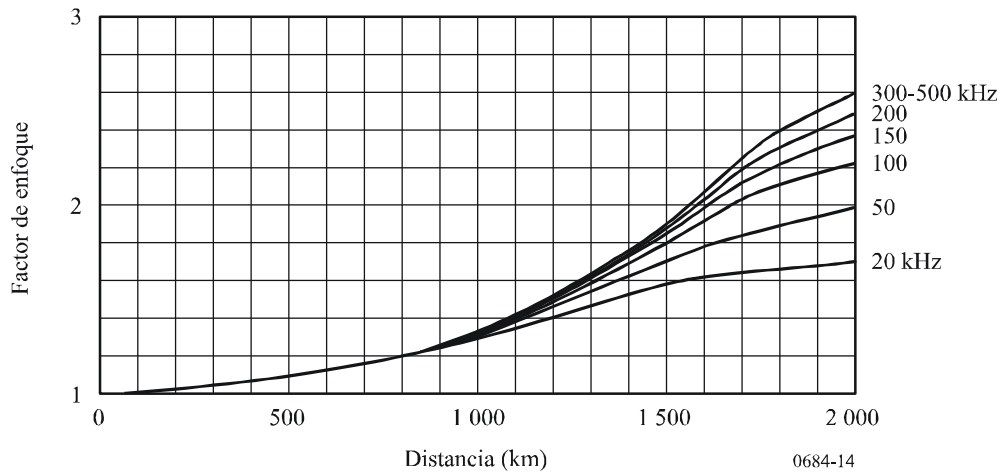
FIGURA 14 Factor de enfoque ionosférico
