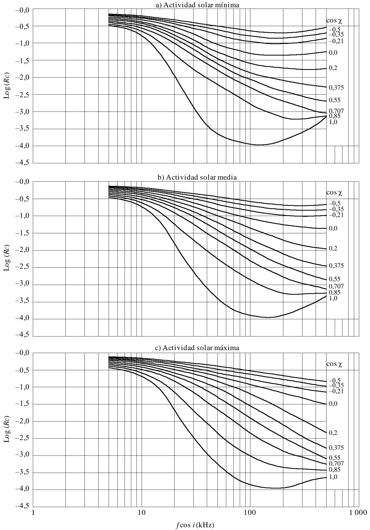
FIGURA 15 Coeficiente de reflexión ionosférica
