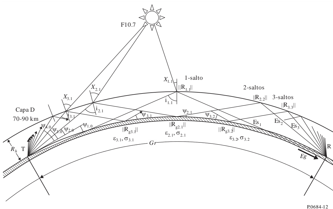
FIGURA 12 Factores de propagación y geometría del trayecto
