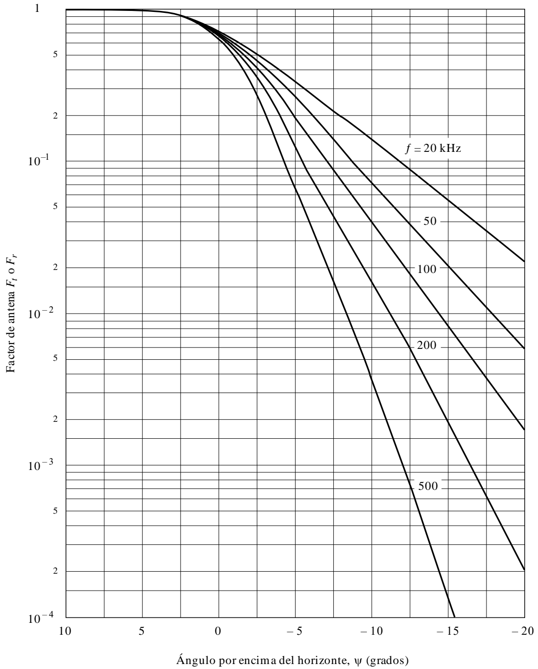
FIGURA 7 Factor de antena – Mar
