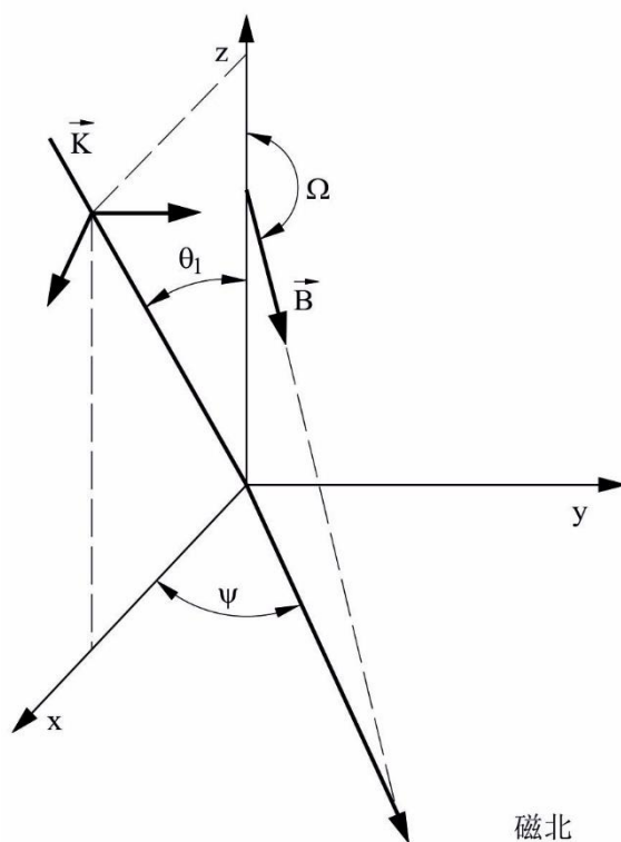
图16 波传播的几何图
