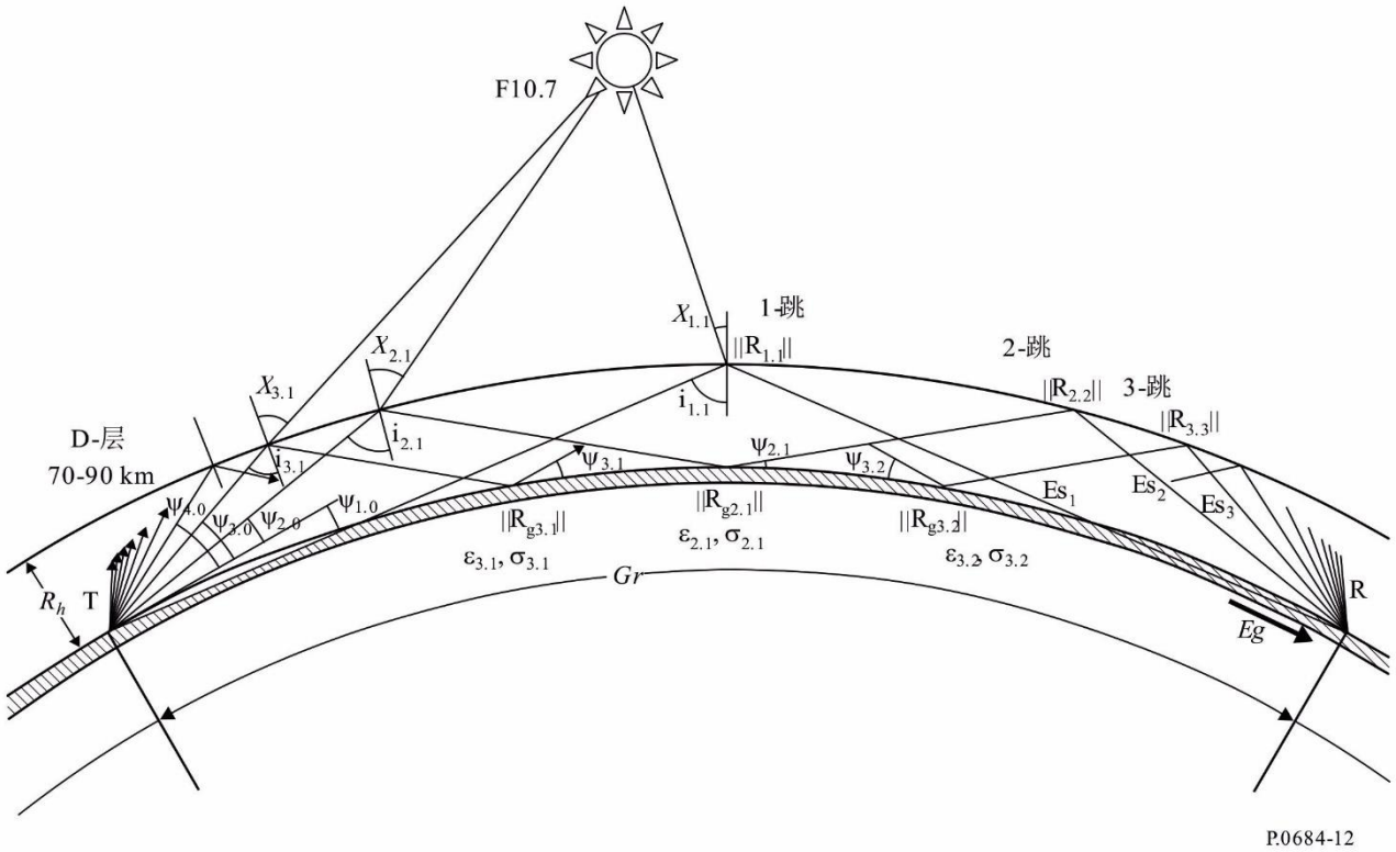
图12 传播因子和路径几何图
