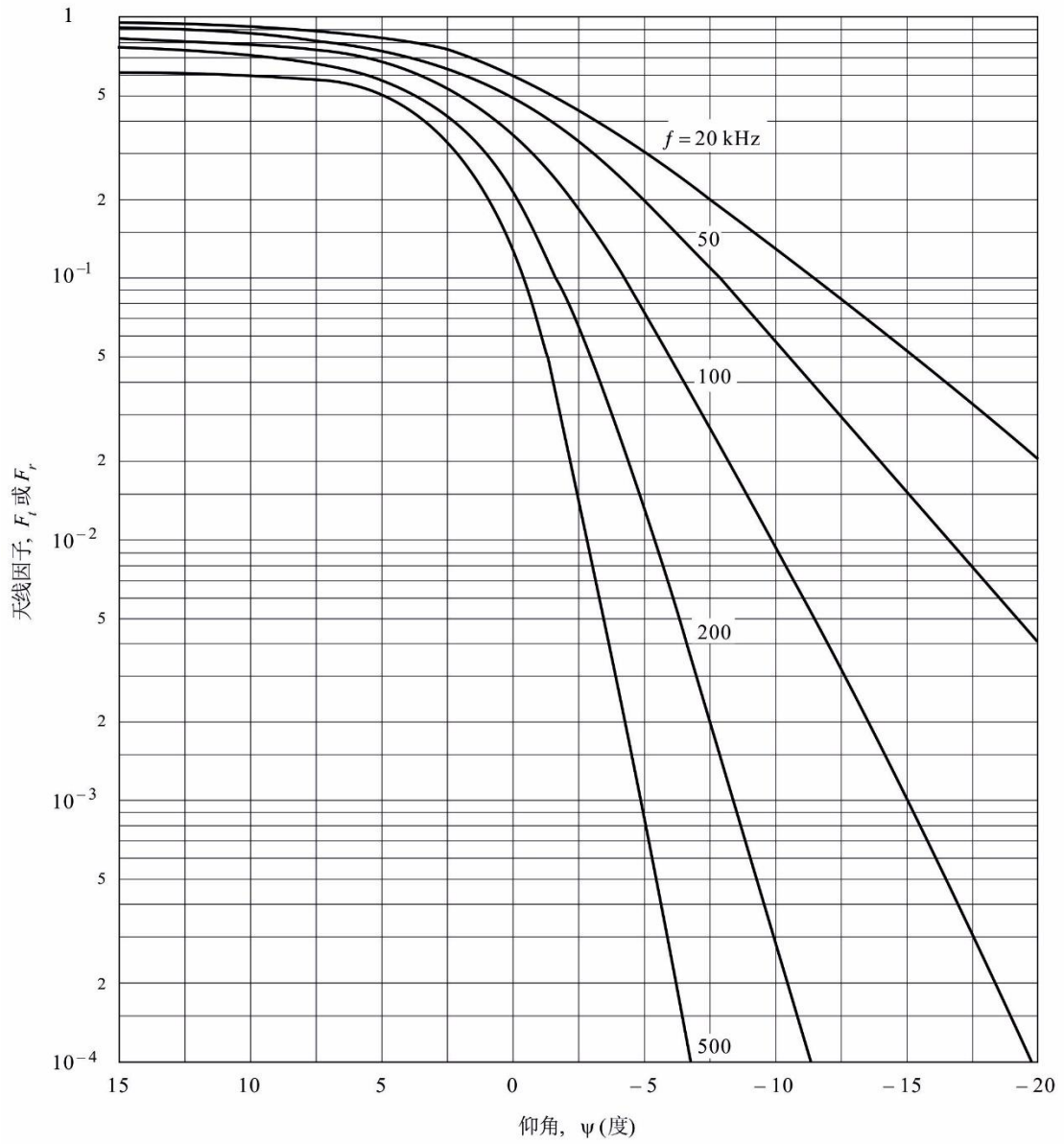
图8 天线因子 - 陆地条件
