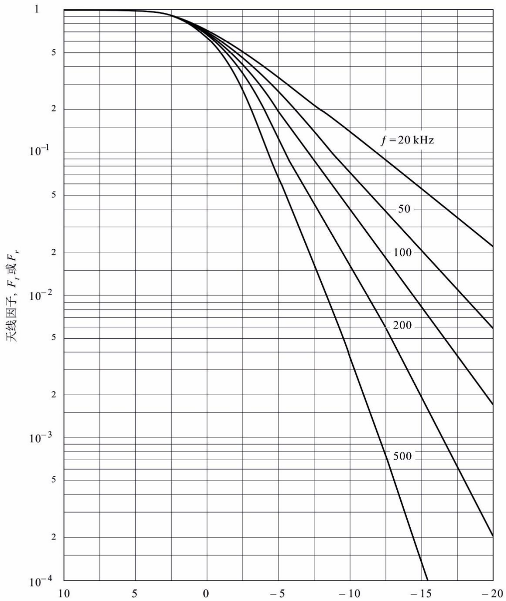
图7 天线因子 - 海水条件
