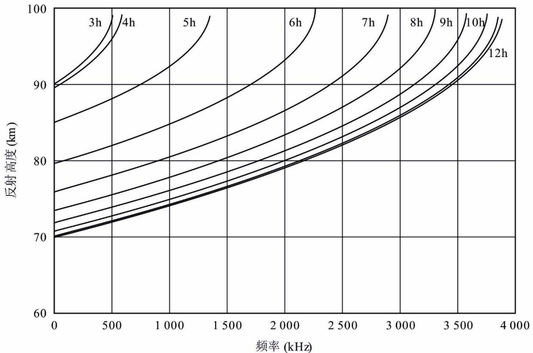
反射层随当地时间的变化情况示例
