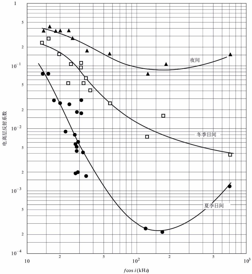
图10 电离层反射系数 - 太阳极小期条件
