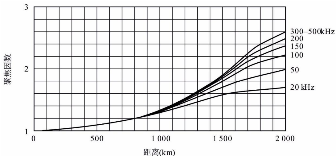
图14 电离层聚焦因数
