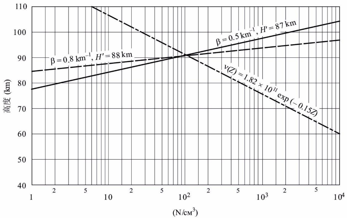
夜间电子密度分布和碰撞频率分布
