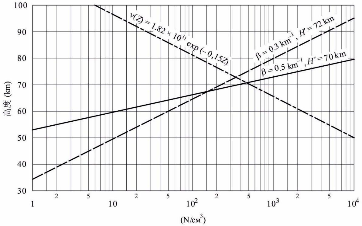
日间电子密度分布和碰撞频率分布
