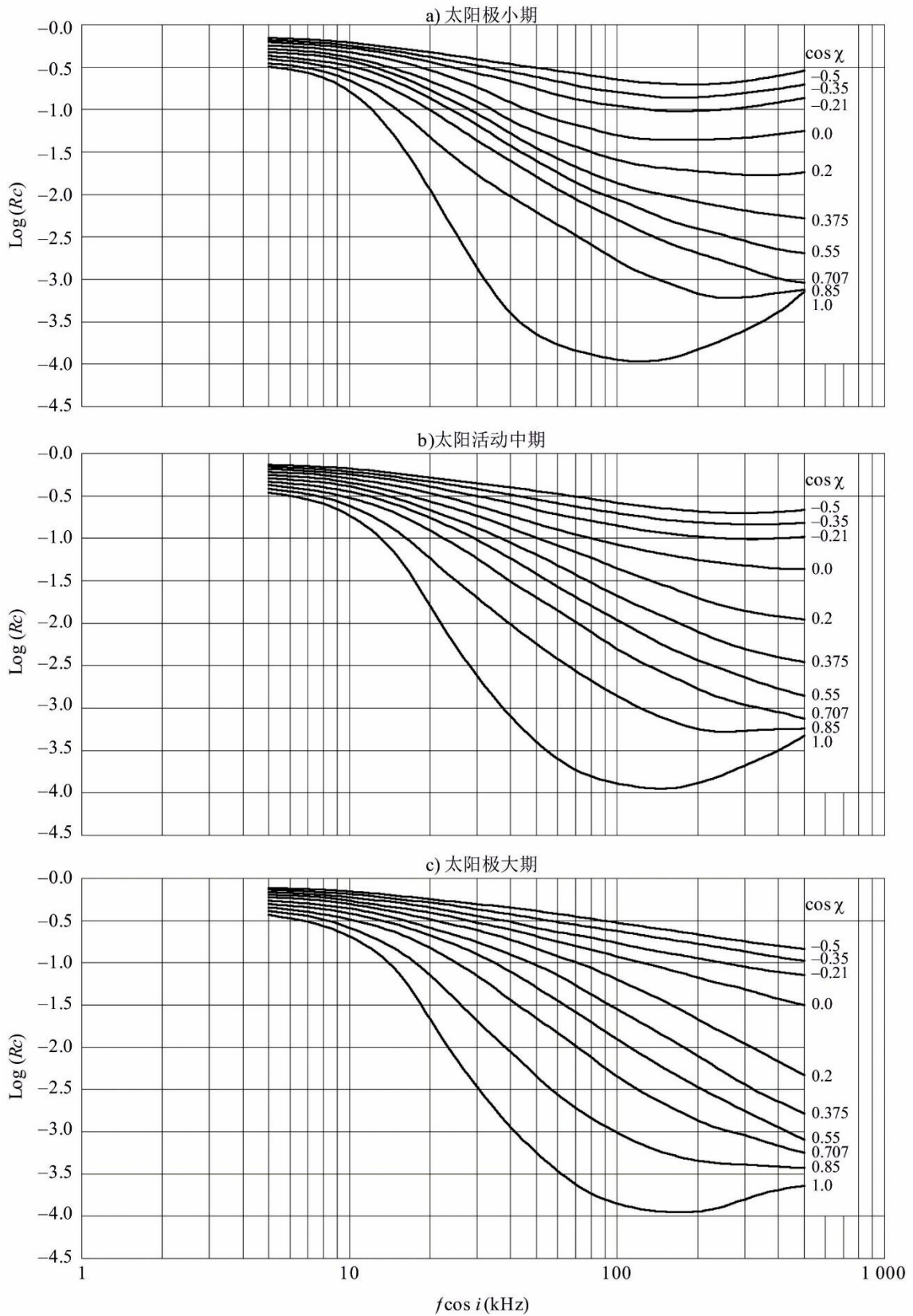
图15 电离层反射系数
