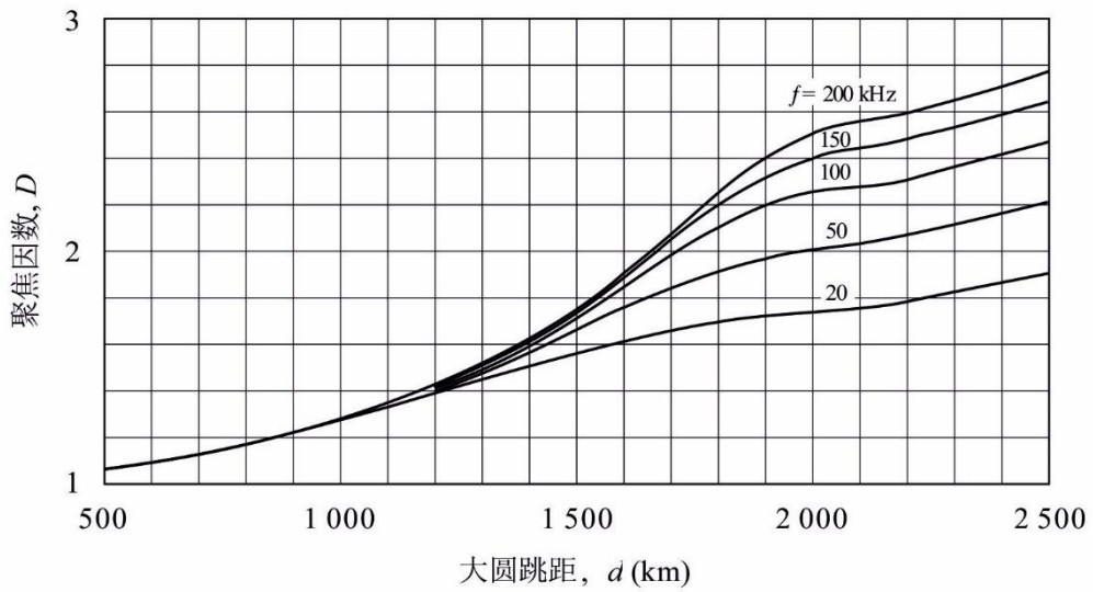
图6 电离层聚焦因数 - 夜间条件
