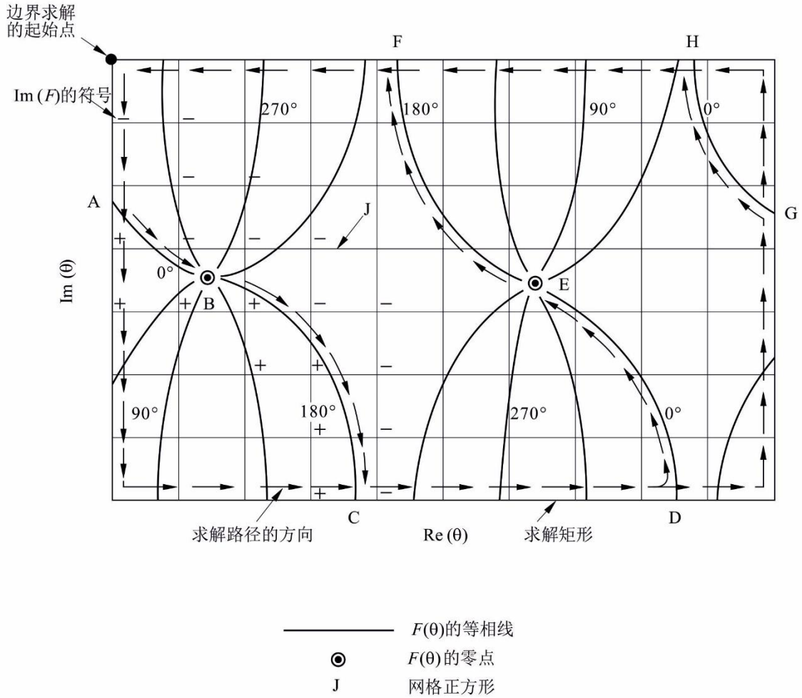
图18 函数法 F(q) 的模式求解
