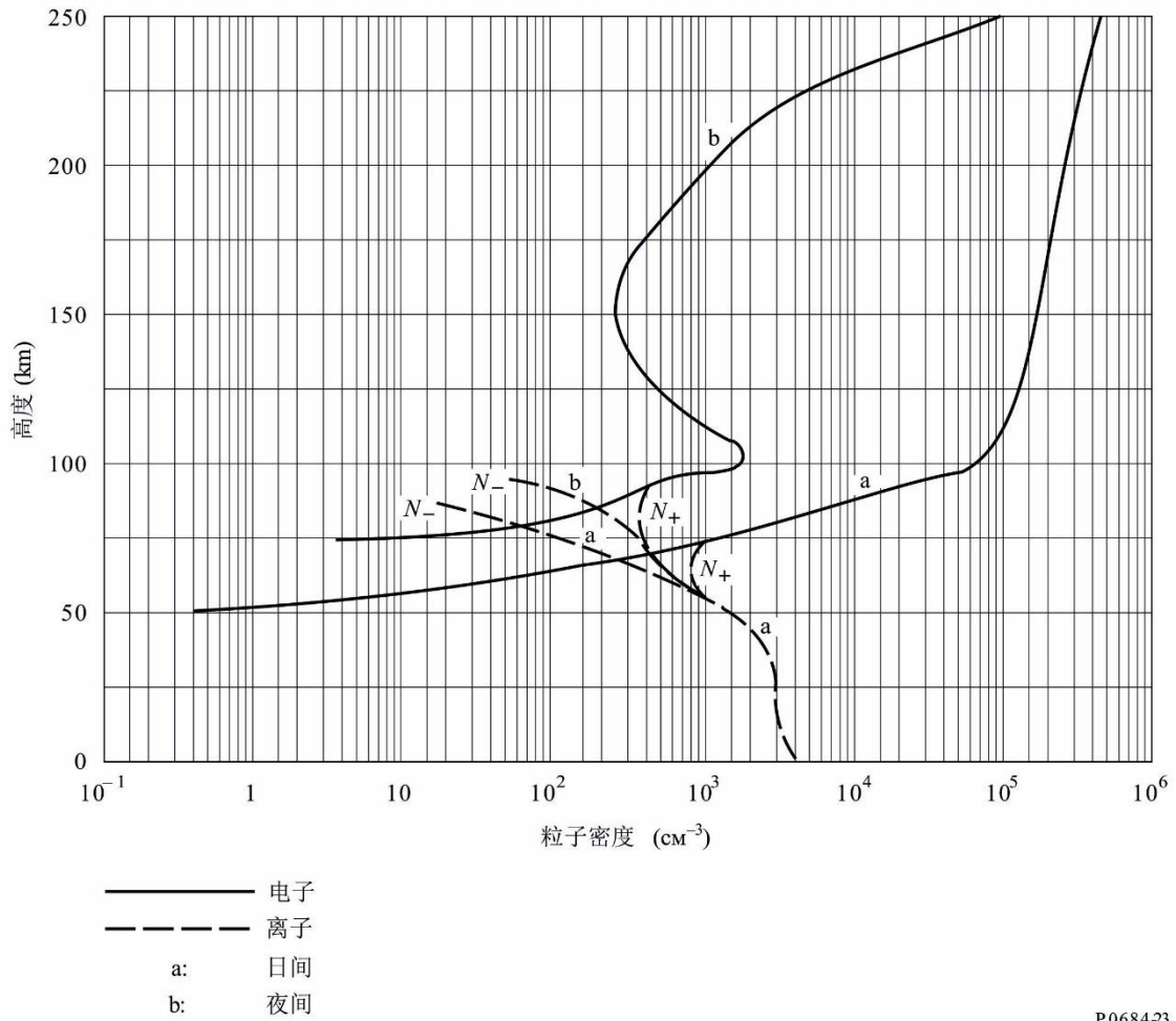
日间和夜间周围成分分布
