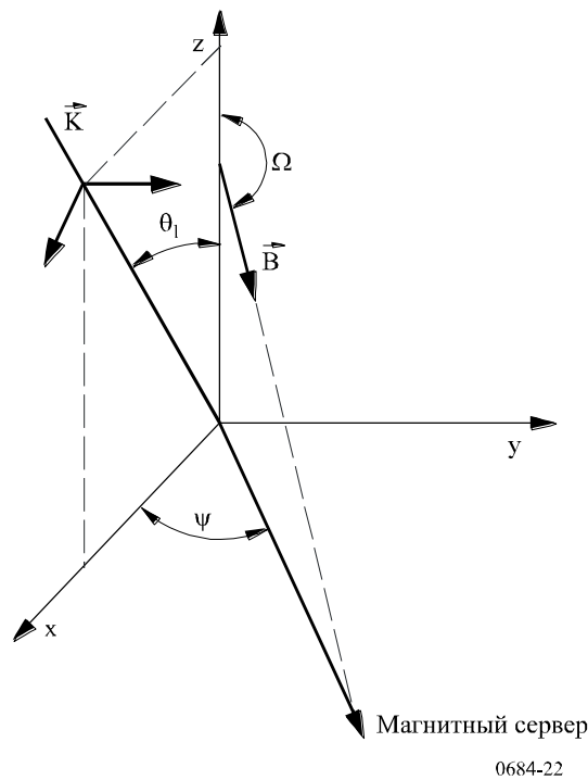
РИСУНОК 22 Геометрия распространения волны
