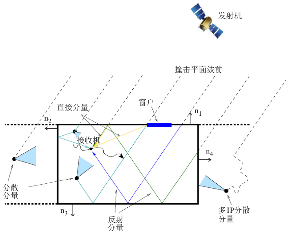
从卫星到室内信道模型中模拟单个组件的概述
