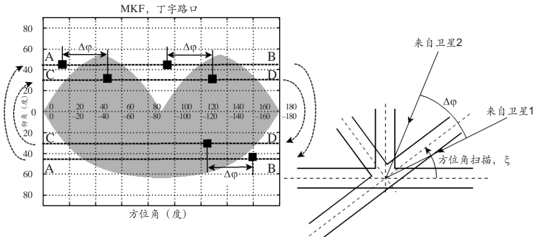
图26 相对于丁字路口的双GSO卫星星座 总系统可用度计算
