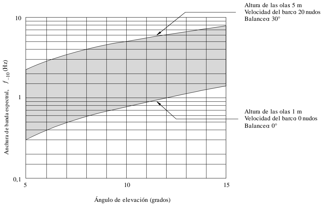
FIGURE 4 Anchura de banda espectral -10 dB del desvanecimiento por trayecto múltiple a 1,5 GHz, debido a la reflexión en el mar en función del ángulo de elevación
