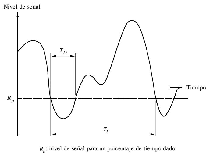
FIGURA 5 Duración de los desvanecimientos e intervalo de ocurrencia de los desvanecimientos
