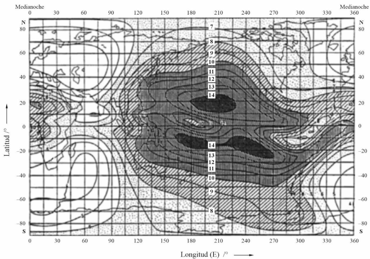
FIGURA 7 Refracción ionosférica
