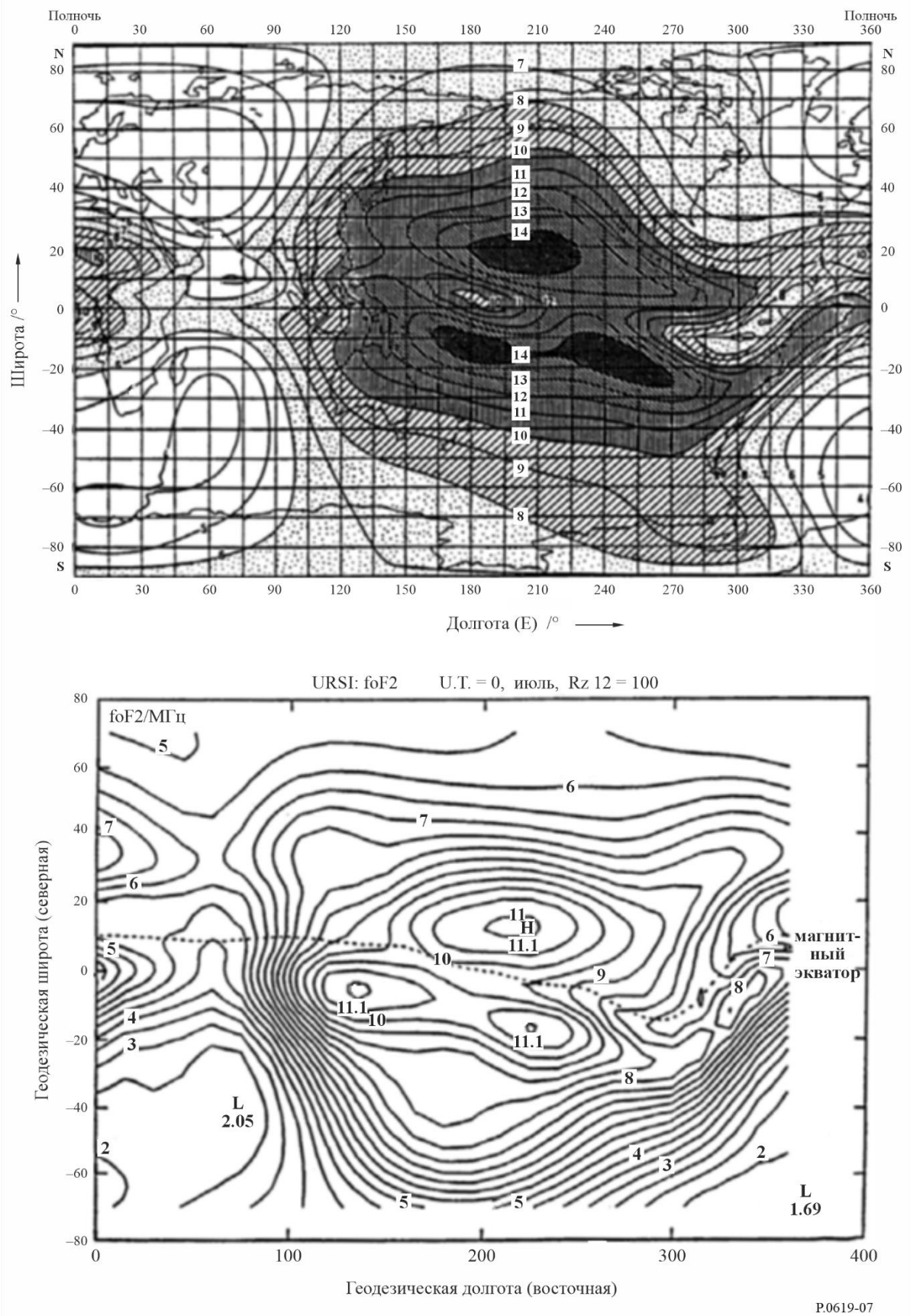
РИСУНОК 7 Ионосферная рефракция
