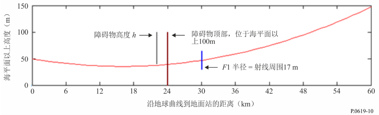
图10 与地对空射线有关的衍射参数几何
