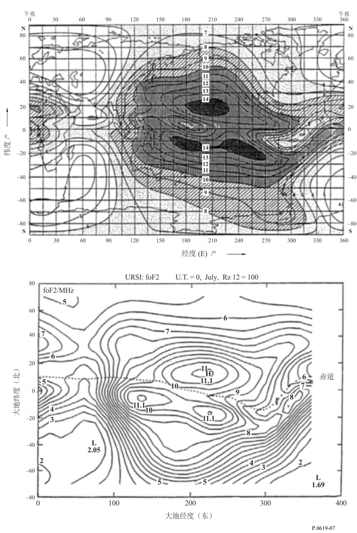
图7 电离层折射
