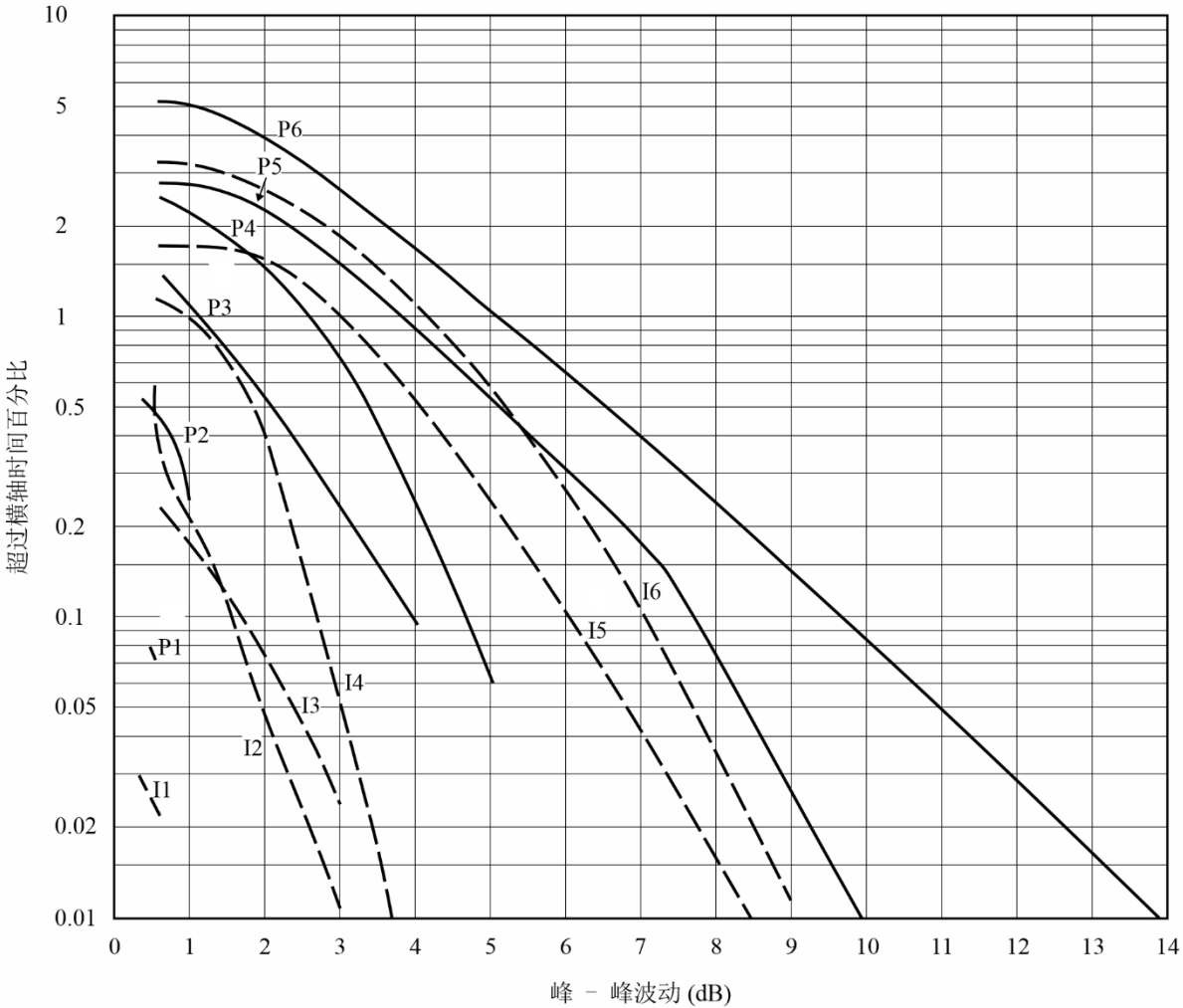
图14 中国香港地球站（曲线I1， P1， I3-I6， P3-P6） 和中国台北地球站（曲线P2和I2）观测到的峰 - 峰波动值年统计表
