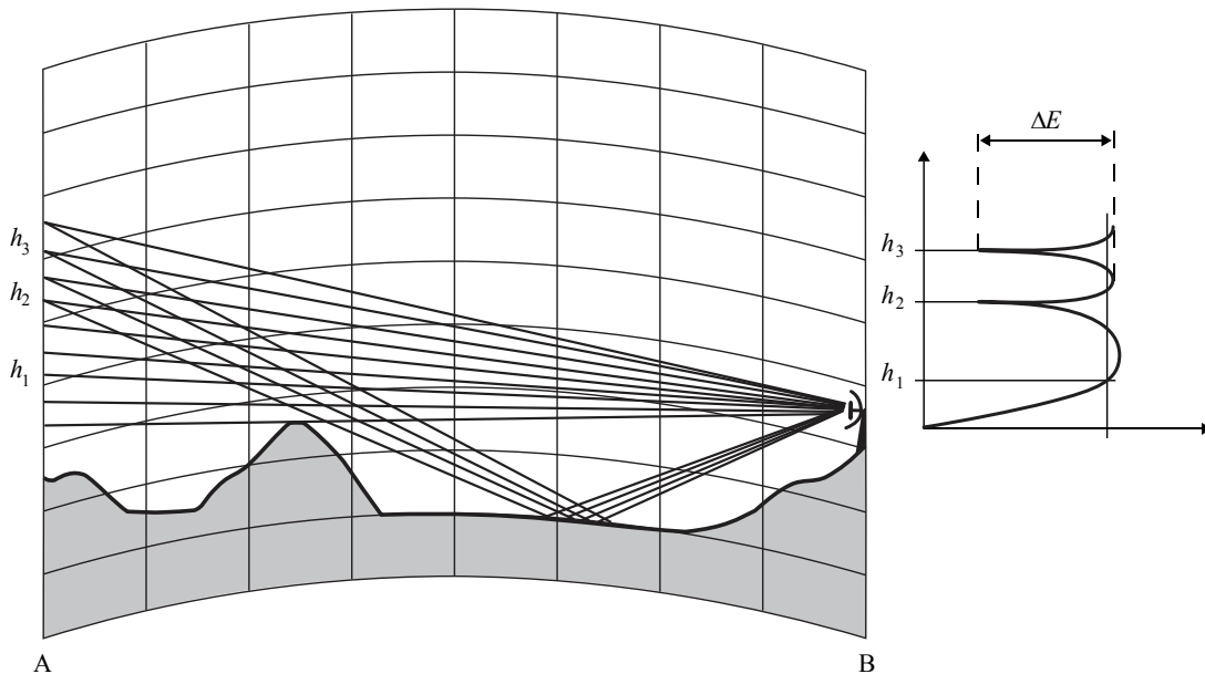
图10 从高度增益图测量 \Delta E (dB)
