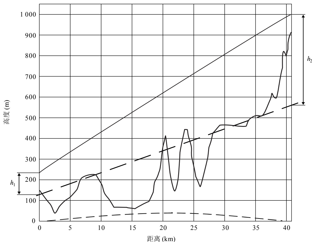
图9 反射地形采用的路径
