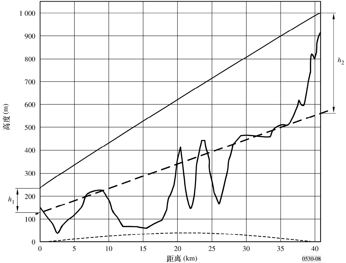
反射地形采用的路径
