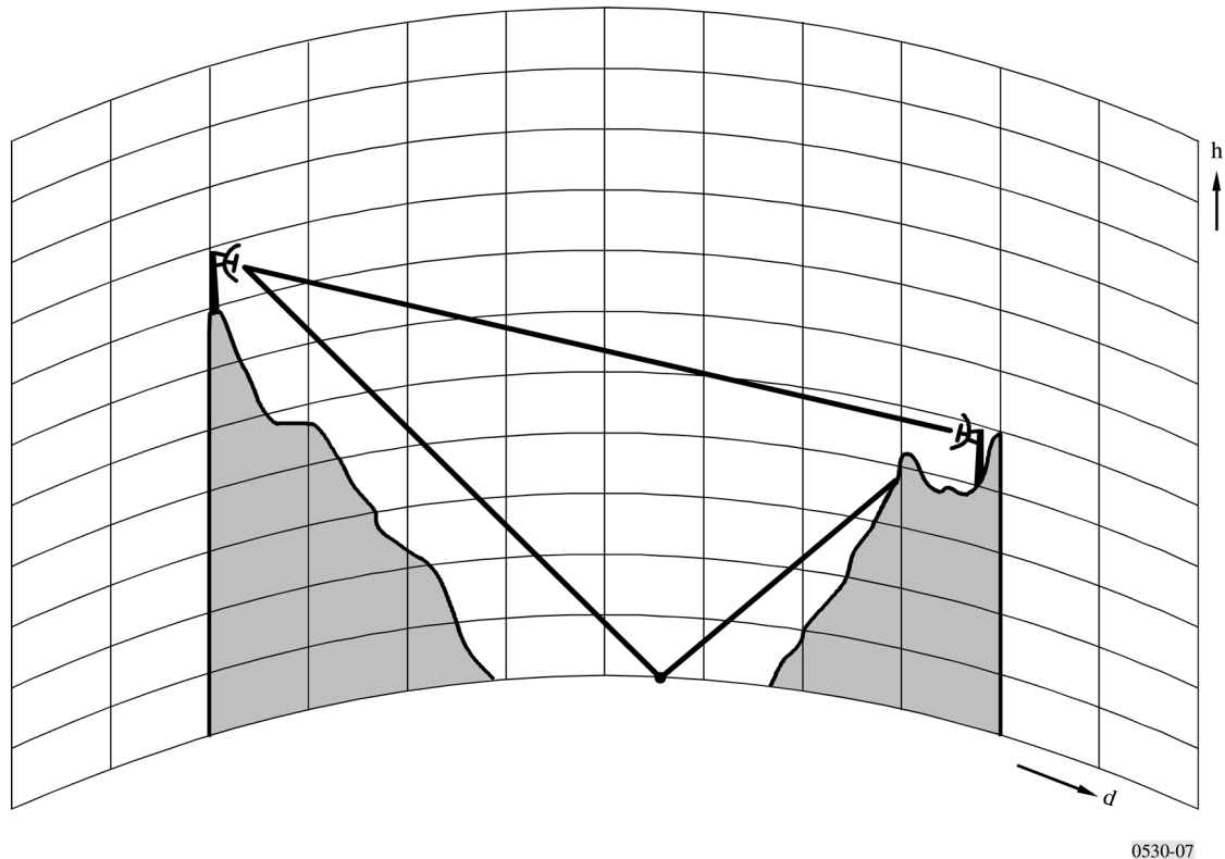
避免天线镜面反射的例子
