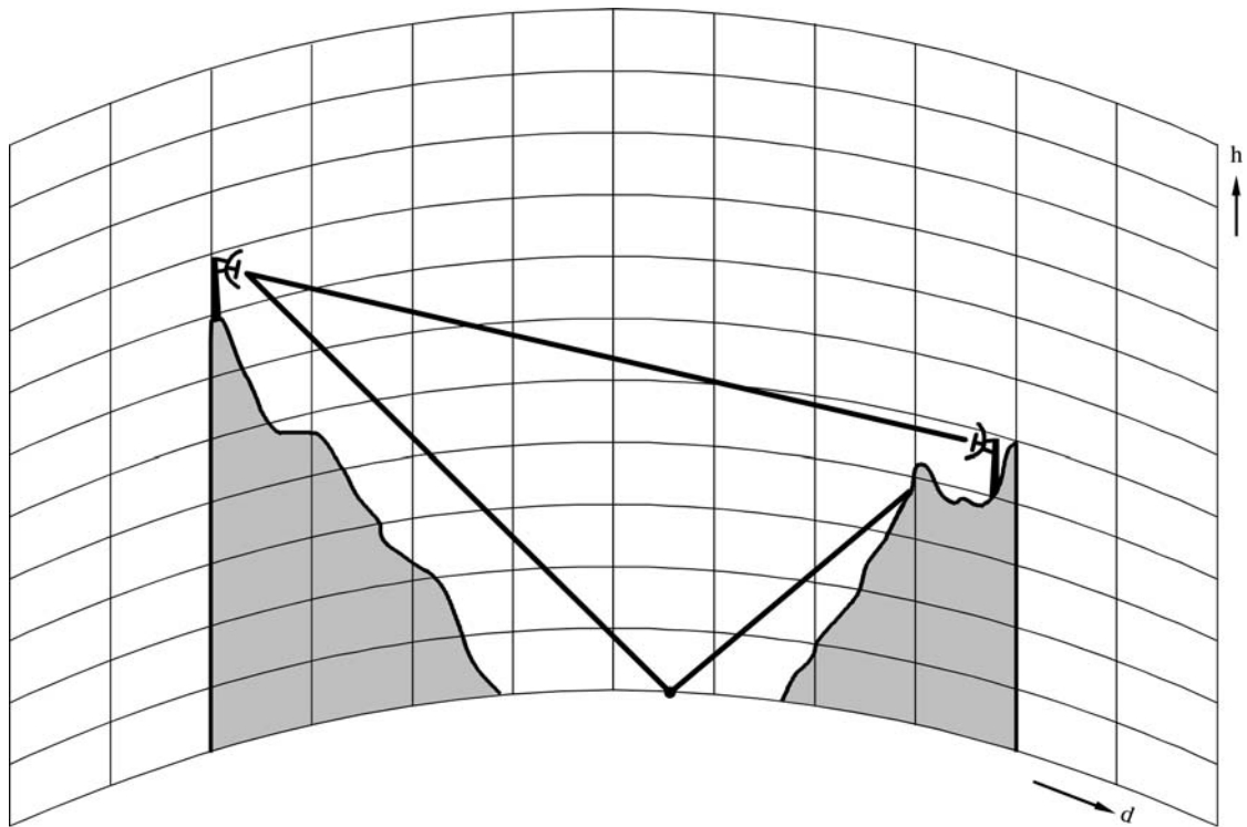
避免天线镜面反射的例子
