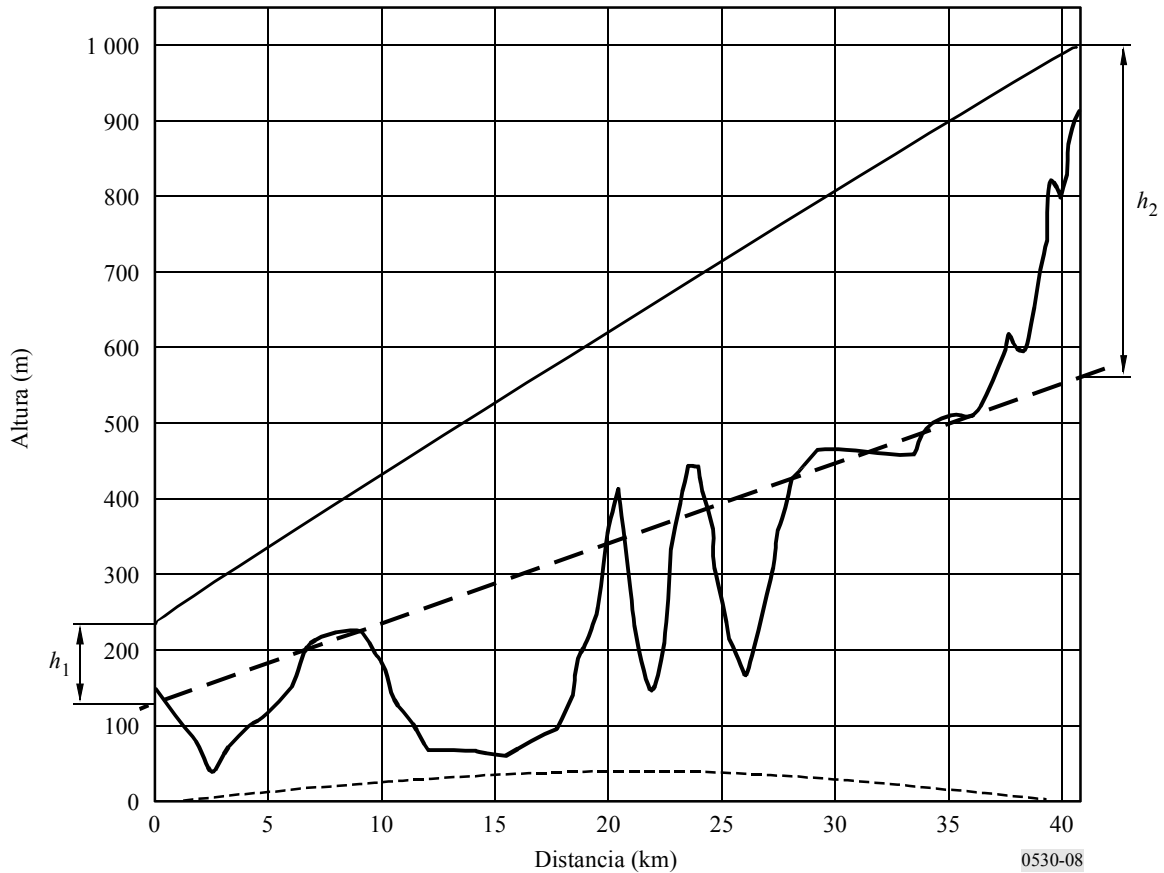
FIGURA 8 Trayecto con terreno reflectivo
