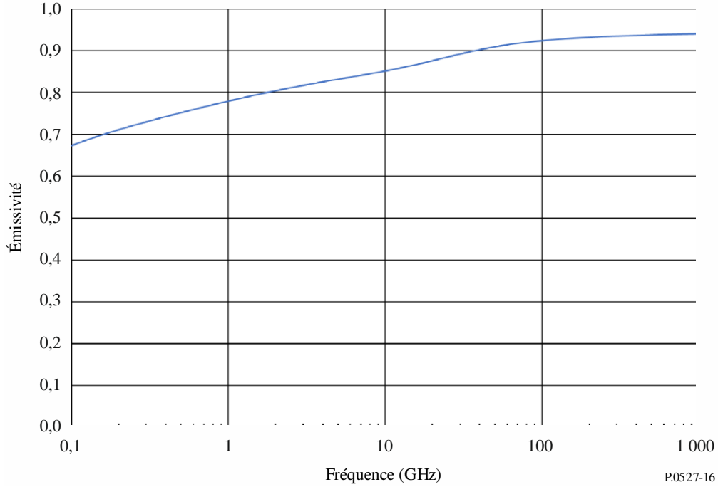
FIGURE 16 Émissivité de la végétation ( M_g = 0,26, T = 22\text{ °C} )
