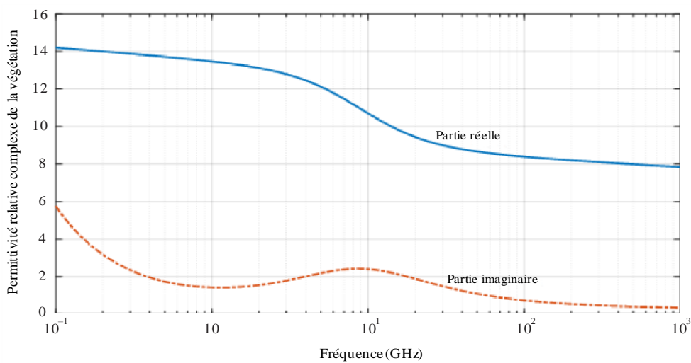
FIGURE 12 Permittivité relative complexe de la végétation en fonction de la fréquence ( M_g = 0,68, T = -7^\circ \text{C} )
