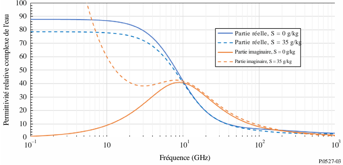
FIGURE 3 Permittivité relative complexe de l'eau pure et de l'eau salée en fonction de la fréquence ( T = 0^{\circ} \text{C} )
