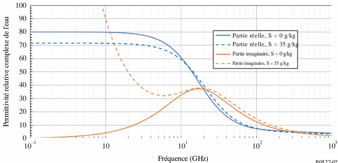
FIGURE 2 Permittivité relative complexe de l'eau pure et de l'eau salée en fonction de la fréquence ( T = 20^\circ \text{C} )
