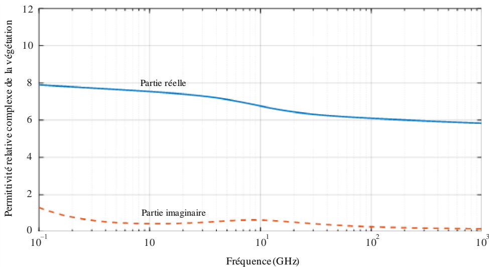
FIGURE 13 Permittivité relative complexe de la végétation en fonction de la fréquence ( M_g = 0,68, T = -10^\circ \text{C} )
