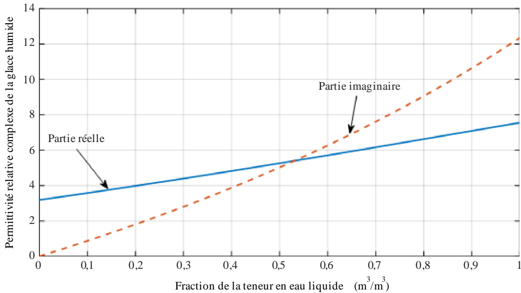
FIGURE 5 Permittivité relative complexe de la glace humide en fonction de la teneur en eau liquide ( f = 60 \text{ GHz} et T = 0^\circ \text{ C} )
