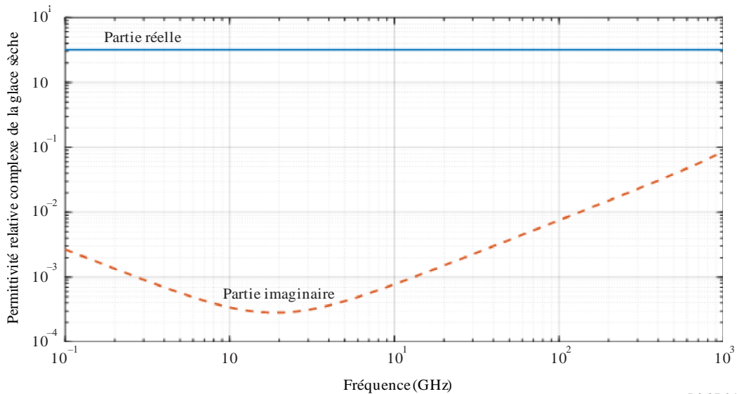
FIGURE 4 Permittivité relative complexe de la glace sèche en fonction de la fréquence ( T = -10^\circ \text{C} )
