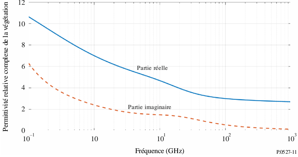
FIGURE 11 Permittivité relative complexe de la végétation en fonction de la fréquence ( M_g = 0,26, T = 22^\circ \text{C} )
