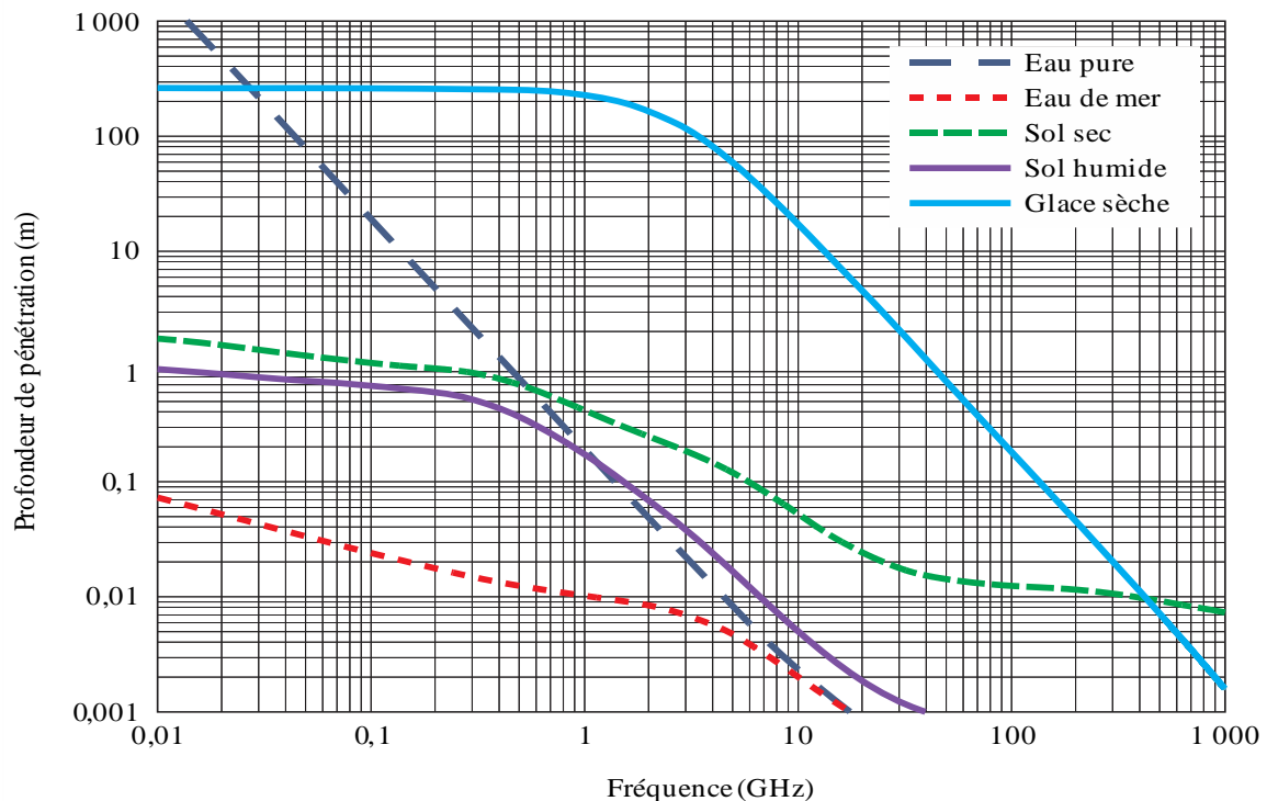
Profondeur de pénétration de différents types de sol en fonction de la fréquence
