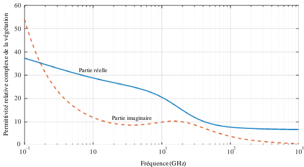
FIGURE 10 Permittivité relative complexe de la végétation ( M_g = 0,68 , T = 22^\circ \text{C} )
