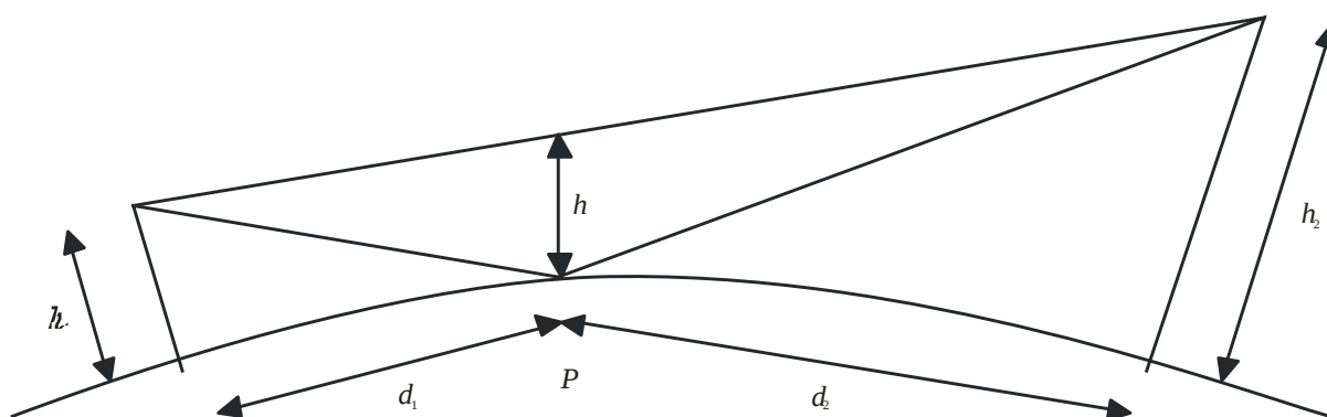
FIGURA 7 Trayecto libre de obstáculos
