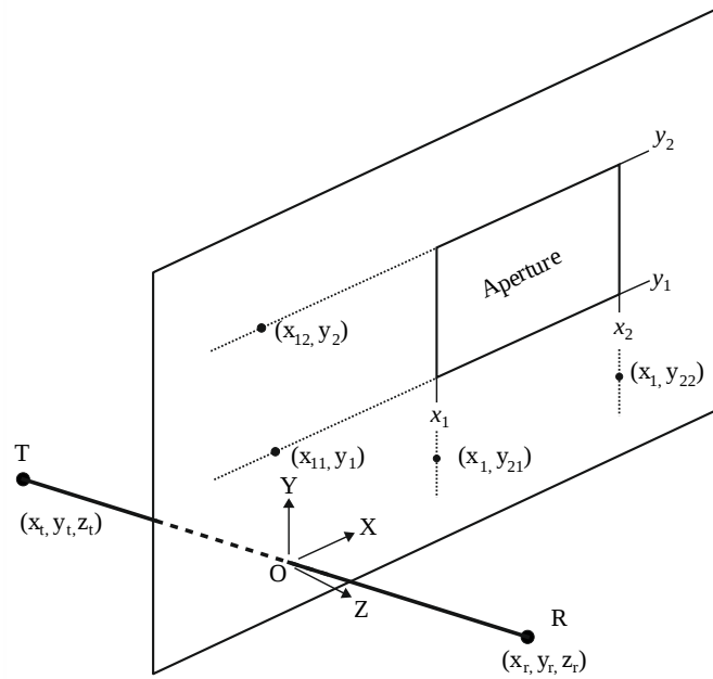
FIGURA 15 Geometría para una abertura rectangular única
