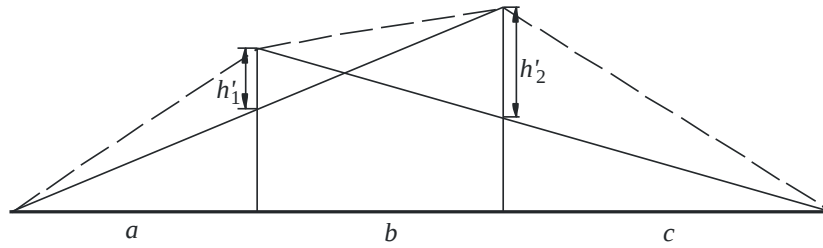
FIGURA 11 Método para dos aristas aisladas
