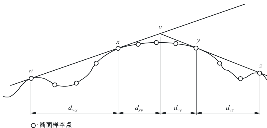
多点障碍物的几何图
