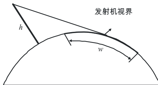
半阴影宽度的确定
