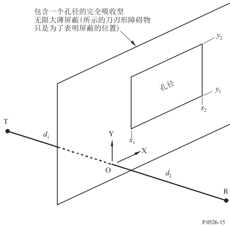
图 15 单个矩形孔径的几何图
