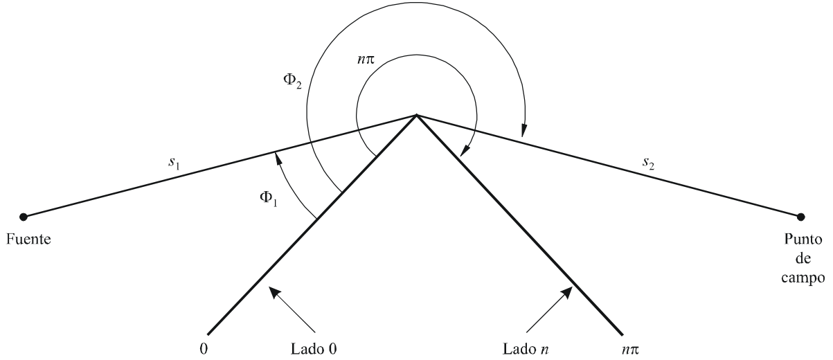
FIGURA 17 Geometría para aplicar la UTD de la difracción por cuña
