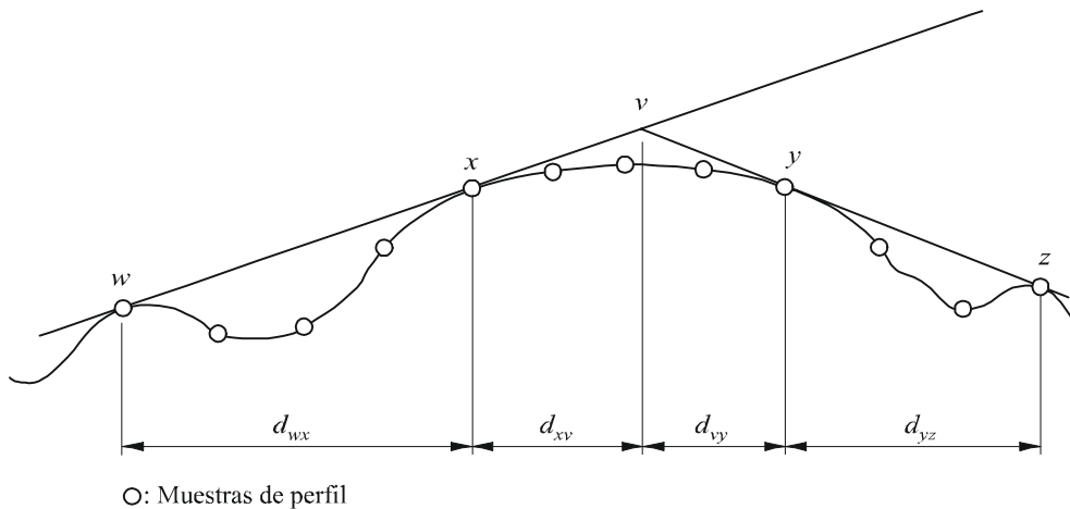
FIGURA 14 Geometría de un obstáculo multipunto
