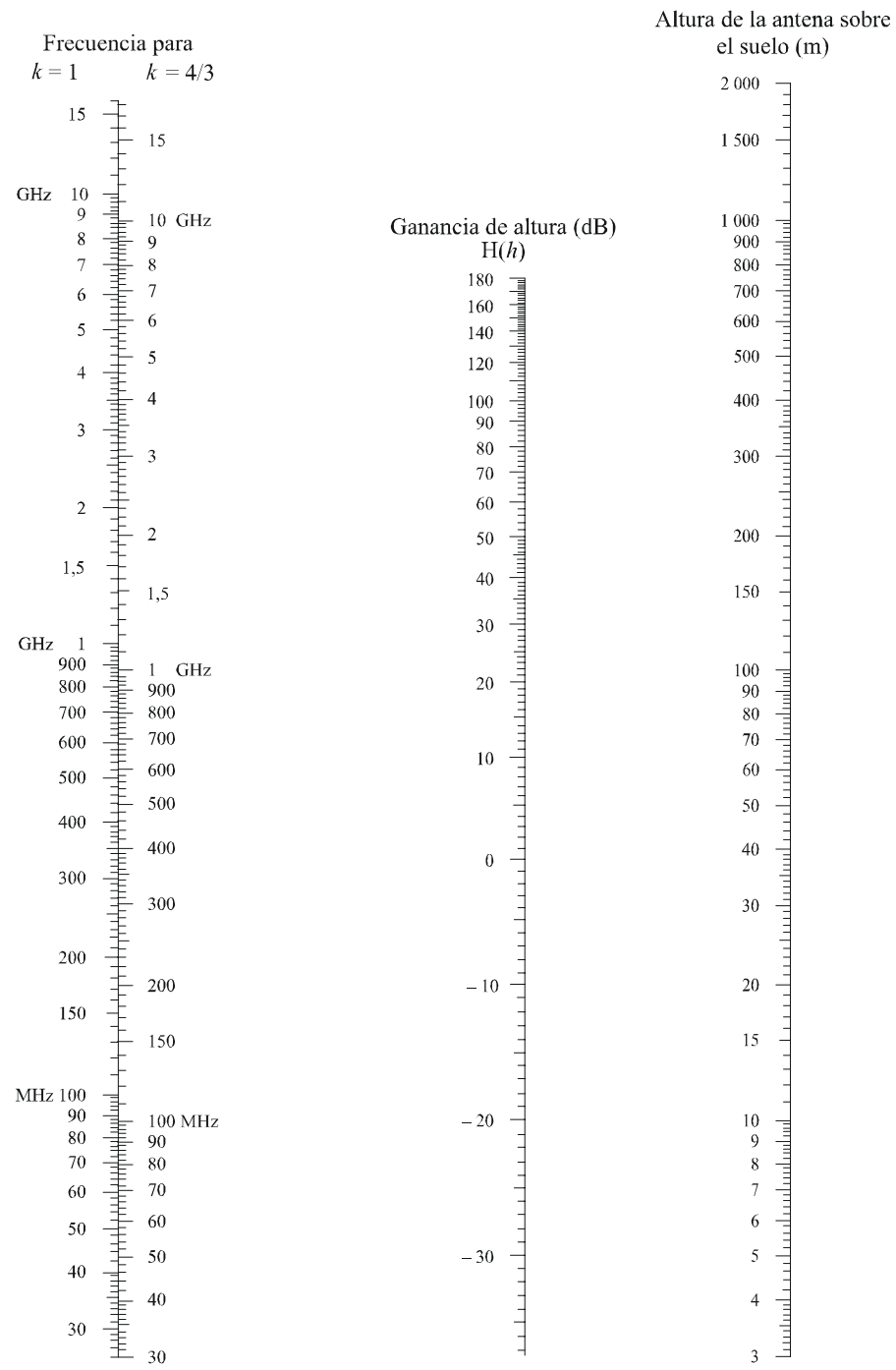
FIGURA 4 Difracción en una Tierra esférica – Ganancia de altura
