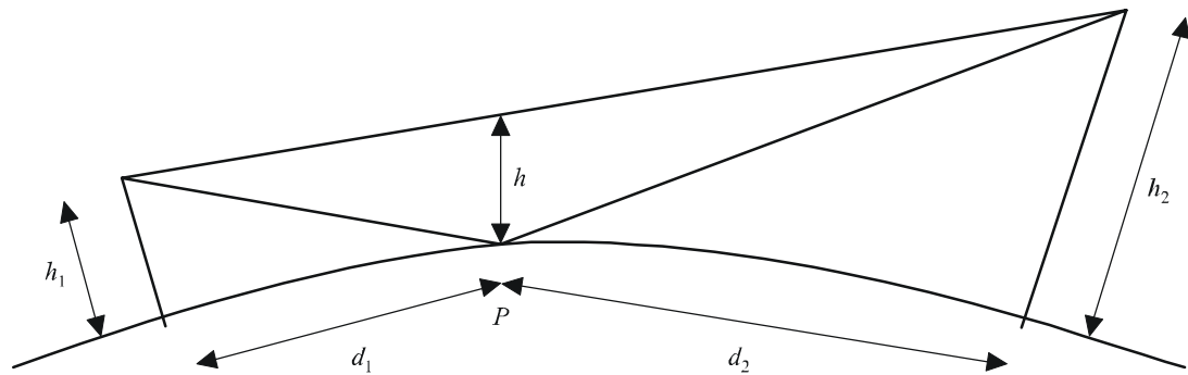
FIGURA 7 Trayecto libre de obstáculos
