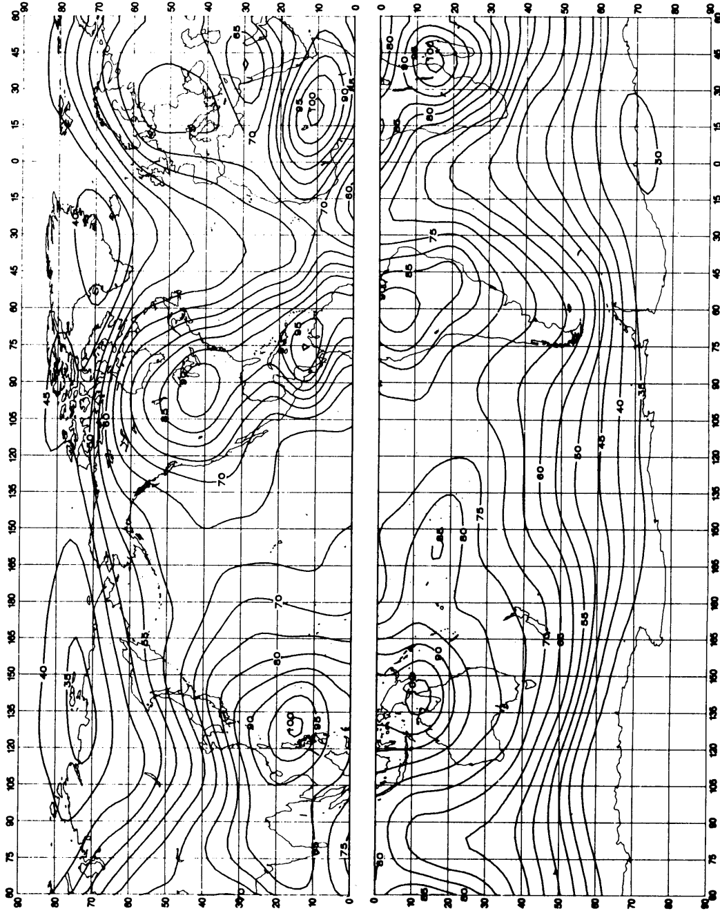
FIGURE 32a -- Valeurs attendues du bruit atmosphérique radioélectrique, F_{am} , en dB au-dessus de kT_{0b} à 1 MHz (Eté; 2000-2400 heure locale)
