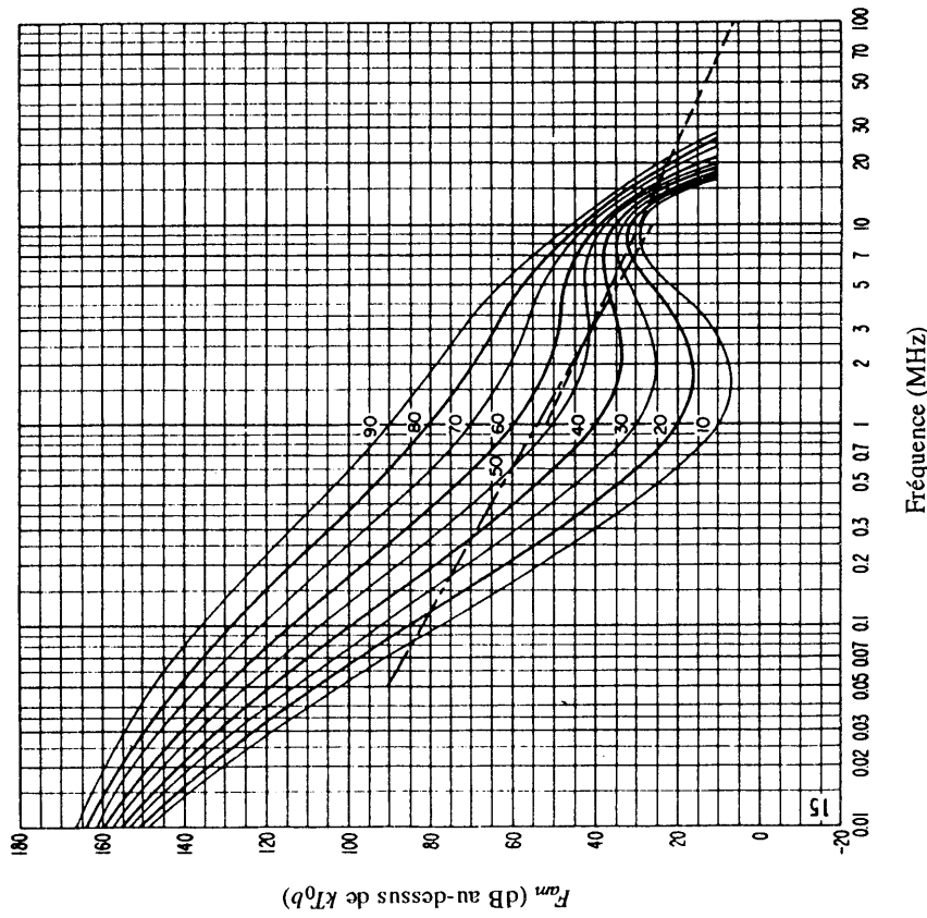
FIGURE 28b – Variation du bruit radioélectrique en fonction de la fréquence (Eti; 0400-0800 heure locale)
