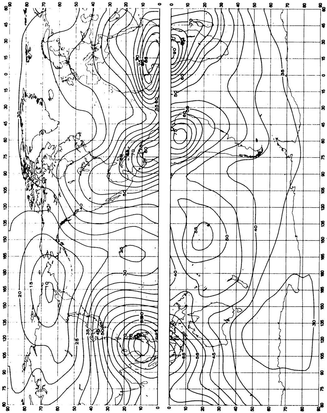
FIGURE 36a – Valeurs attendues du bruit atmospherique radioelectrique, F_{am} , en dB au-dessus de kT_0b à 1 MHz (Automne; 1200-1600 heure locale)
