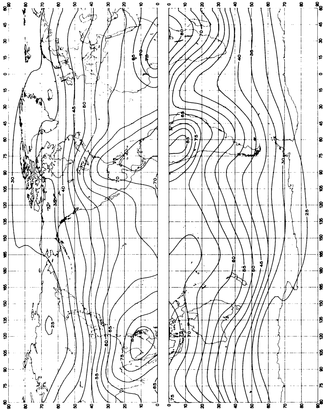
FIGURE 22a – Valeurs attendues du bruit atmosphérique radioélectrique, F_{0.1M} , en dB au-dessus de kT_0b à 1 MHz (Printemps; 0400-0800 heure locale)
