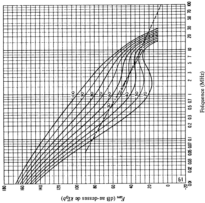
FIGURE 32b — Variation du bruit radioélectrique en fonction de la fréquence (Eie; 2000-2400 heure locale)
