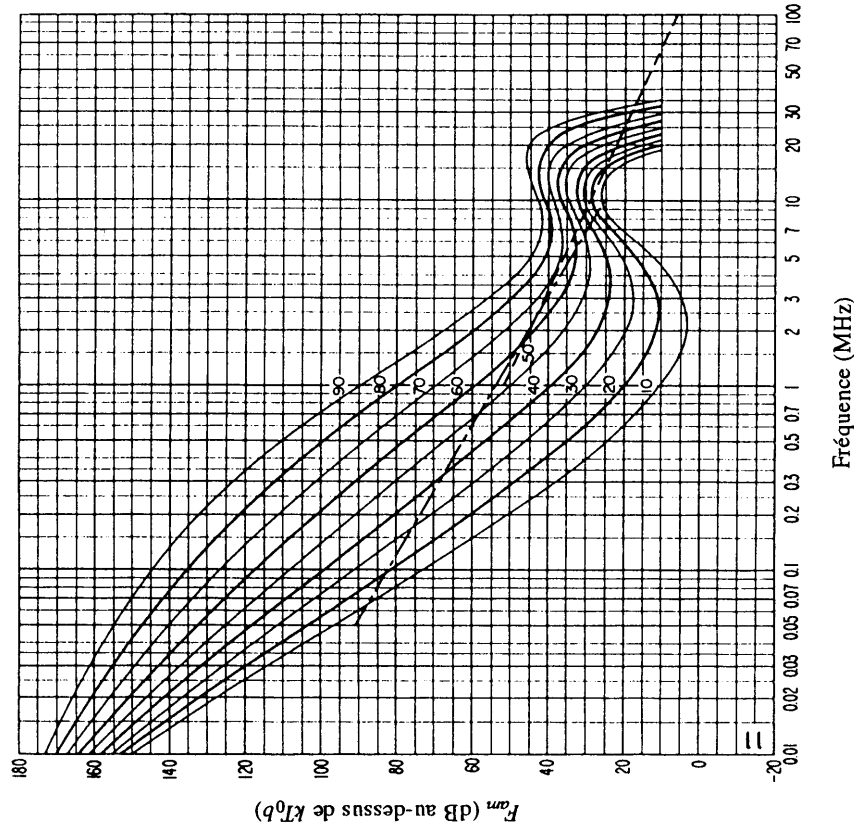
FIGURE 24c – Données sur la variabilité et le caractère du bruit (Printemps; 1200-1600 heure locale)
