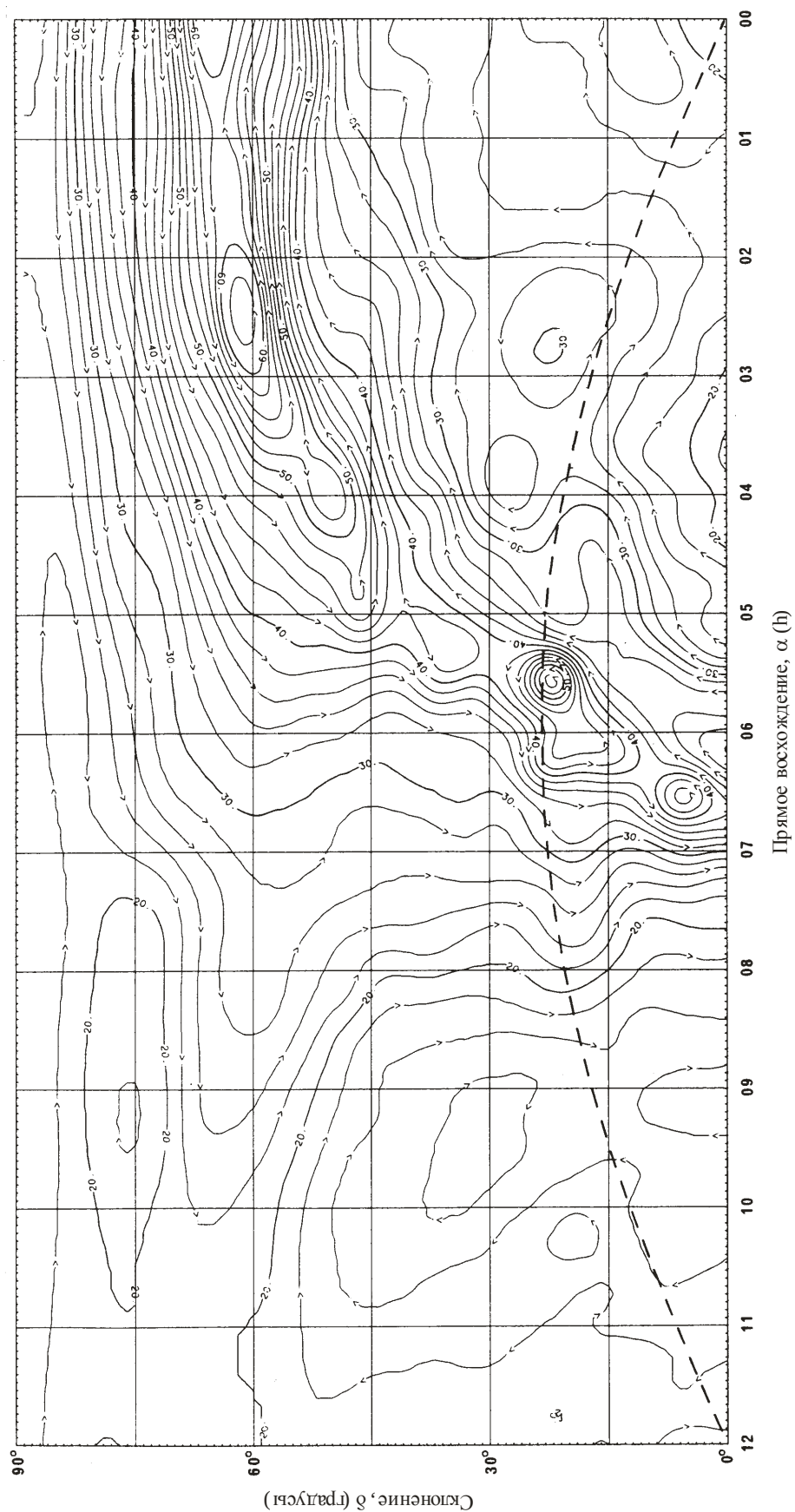
РИСУНОК 13а Температура неба на частоте 408 МГц
