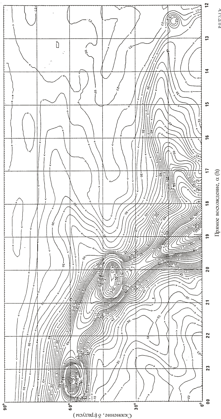
РИСУНОК 13с Температура неба на частоте 408 МГц
