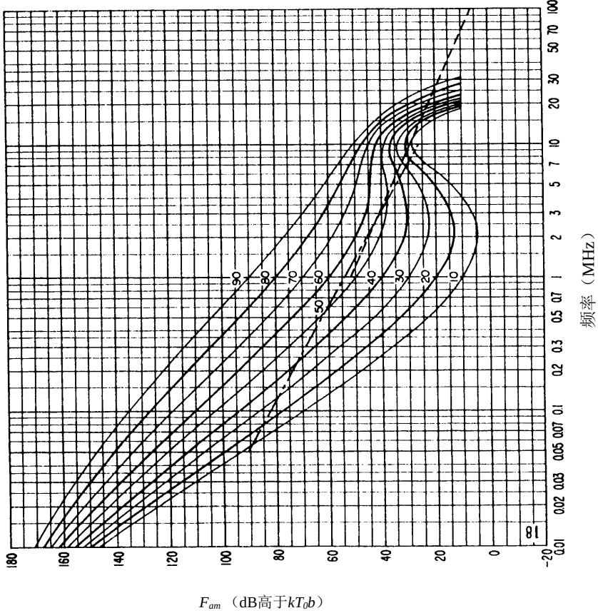
图 31b—无线电噪声随频率的变化 (夏季; 1600-2000LT)
