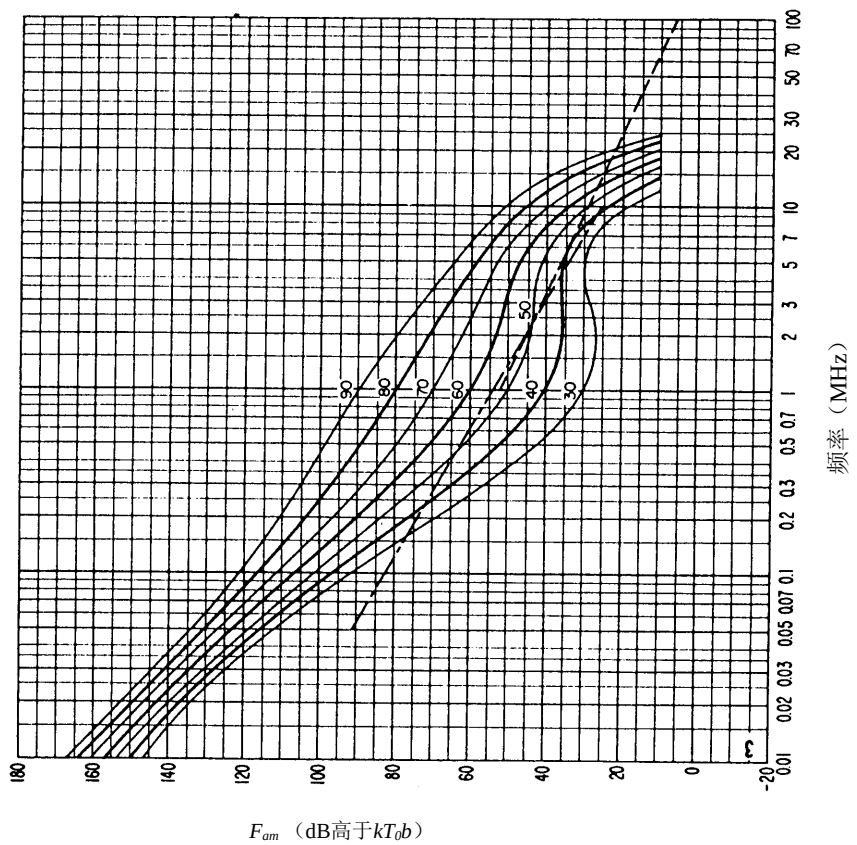
图 16b—无线噪声功率谱密度的变化 (冬季; 0400-0800LT)
