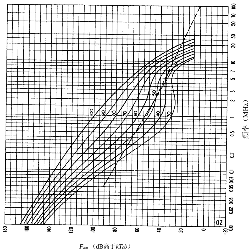
图 33b-无线电噪声声随频率的变化 (秋季; 0000-0400LT)
