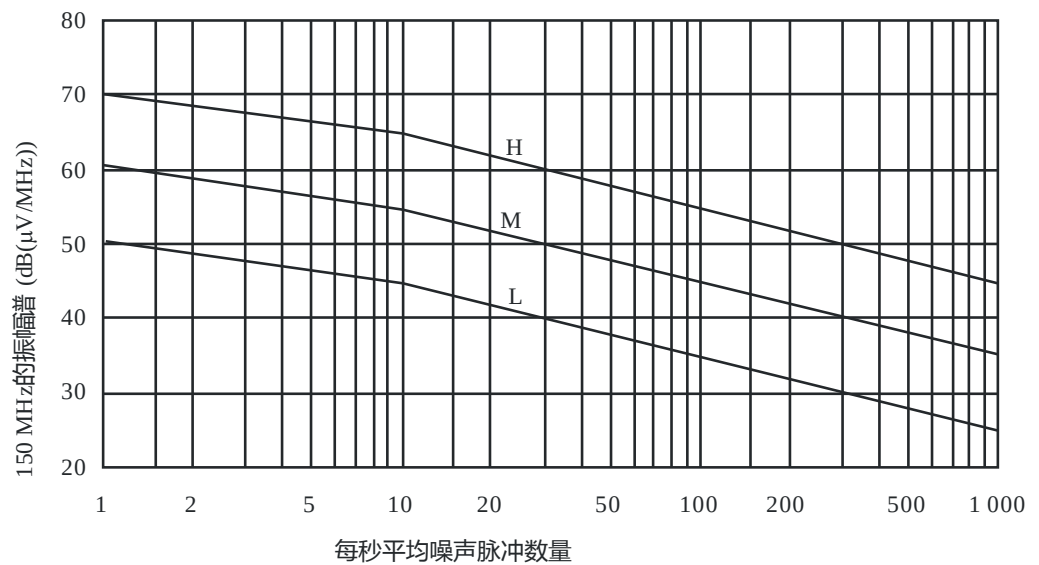
基站噪声振幅分布(150 MHz)
