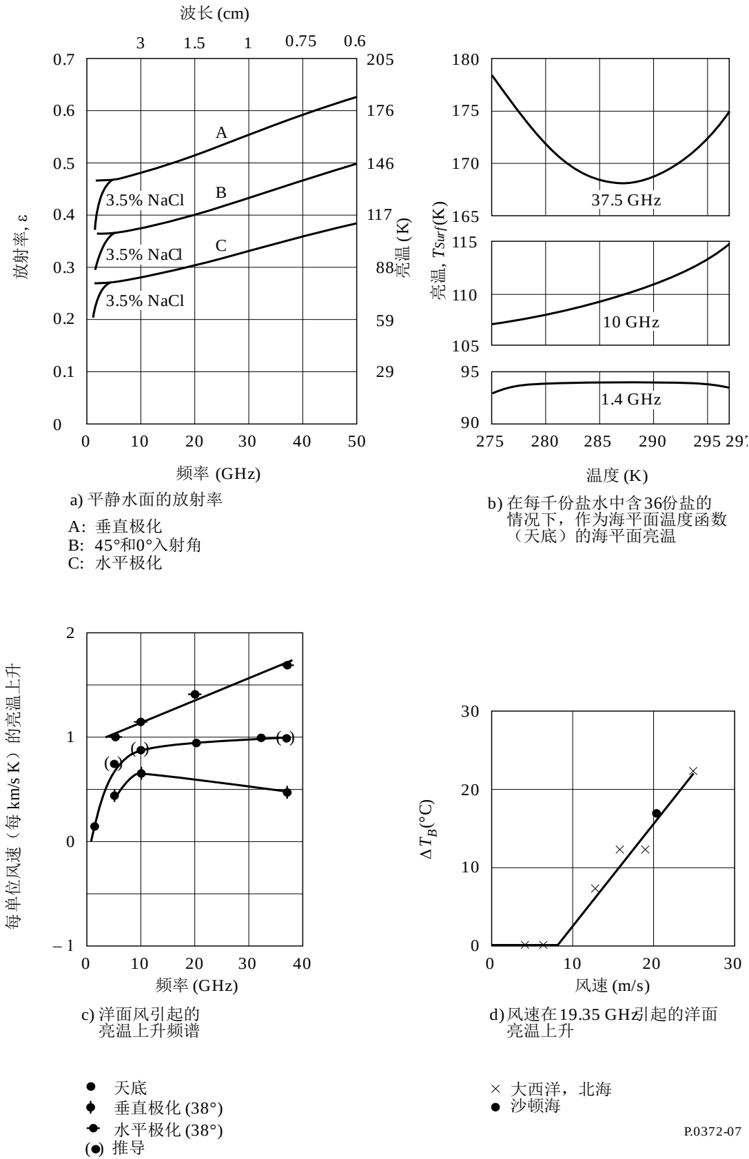
图 7 海平面放射率和亮温的变化
