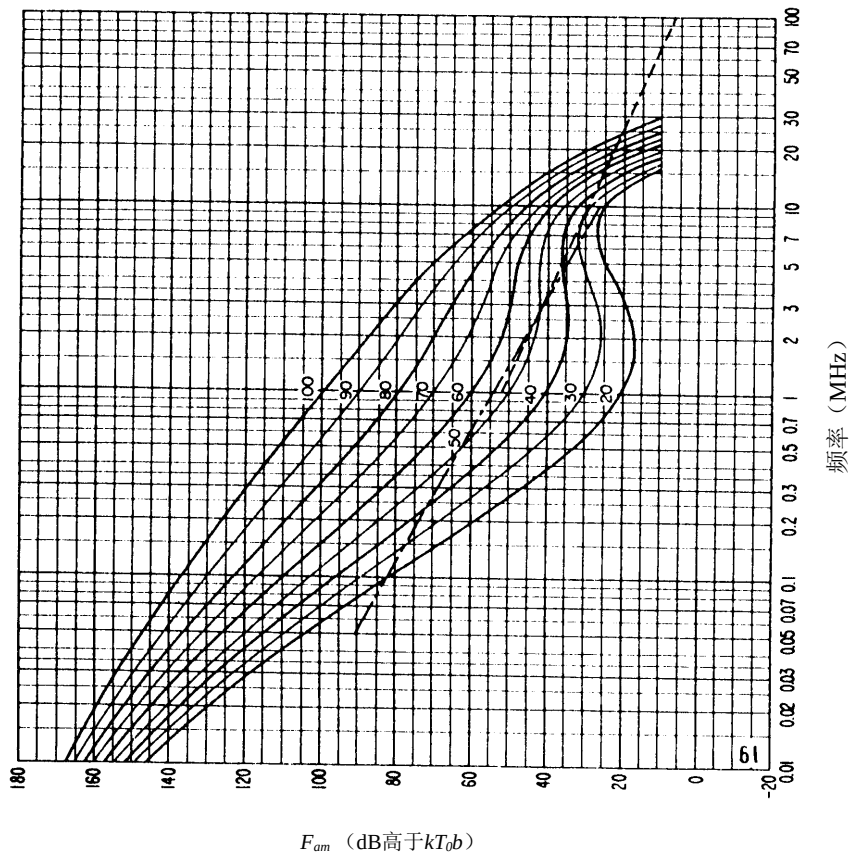
图 32b—无线电噪声随频率的变化 (夏季; 2000-2400LT)
