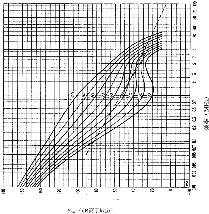
图 15b-无线电噪声随频率的变化
