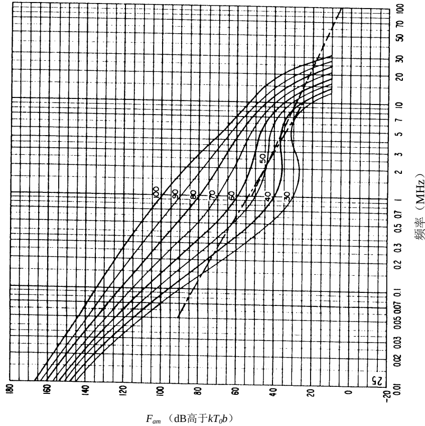
图 38b-无线电噪声随频率的变化 (秋季; 2000-2400LT)
