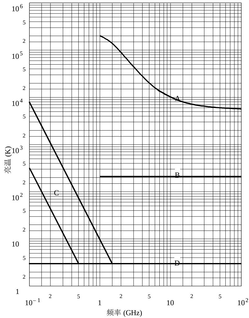
图12 地外噪声源
