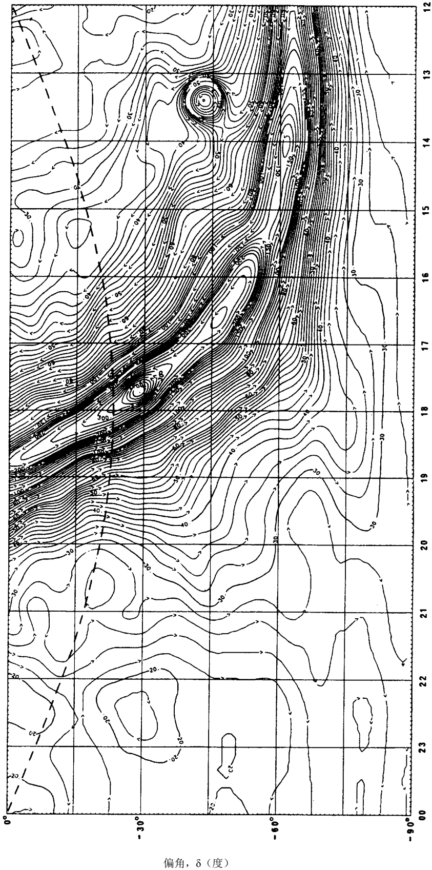
图13d 408 MHz的无线电天空温度
