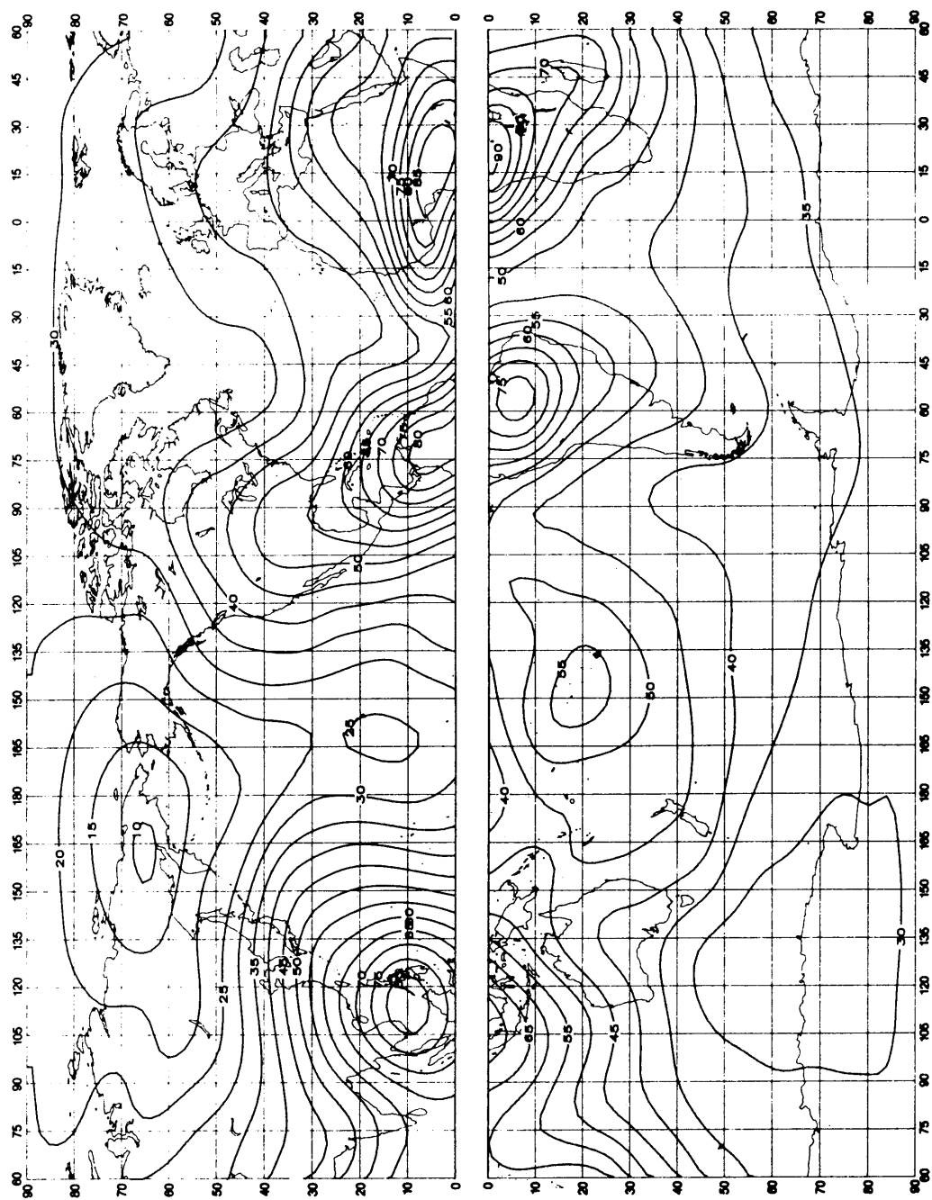
图36a-大气无线电噪声的预计值, F_{am} (1 MHz的dB高于 kT_0b ) (秋季; 1200-1600LT)
