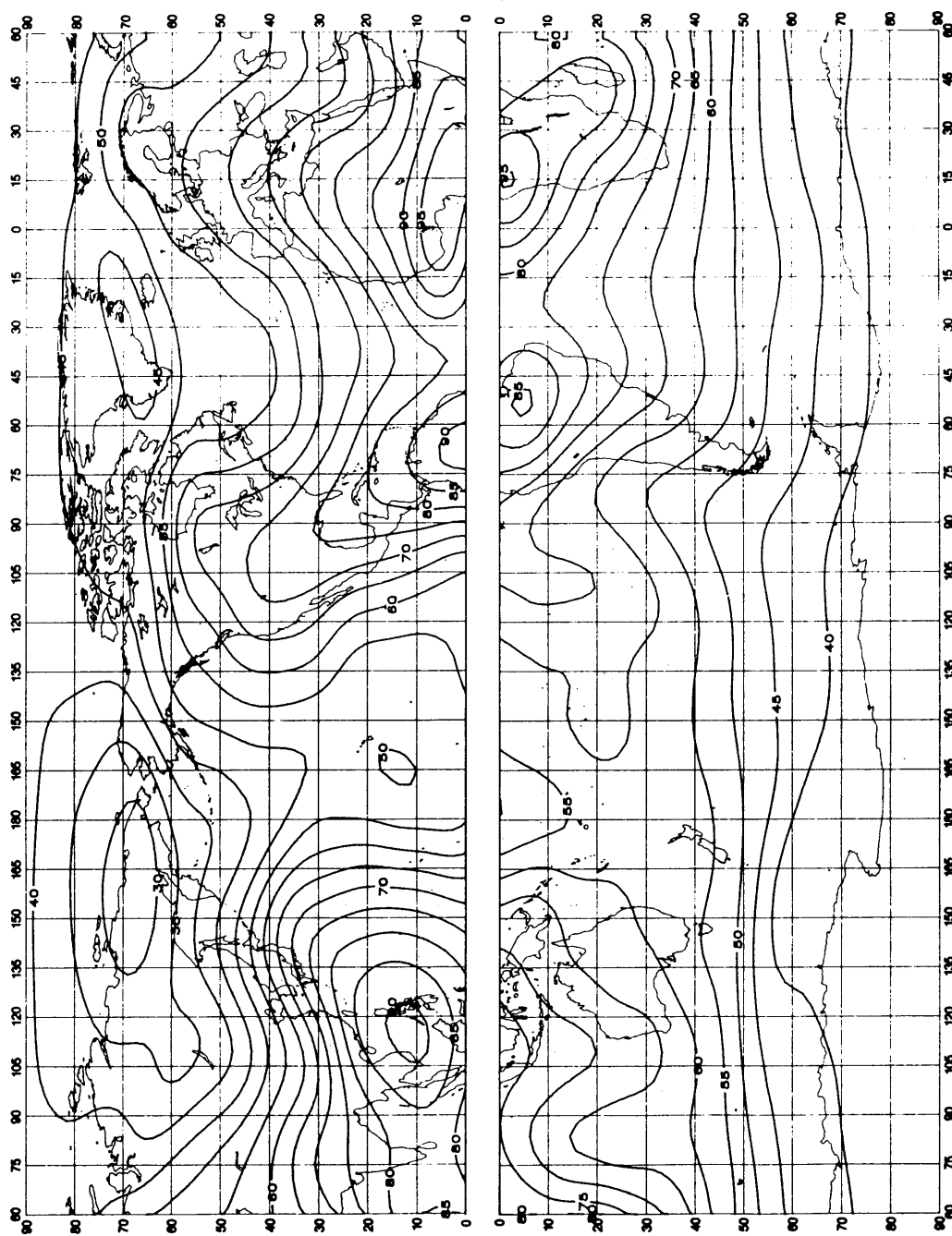
图37a-大气无线噪声的预计值, F_m (1 MHz的dB高于 kT_0b ) (秋季; 1600-2000LT)
