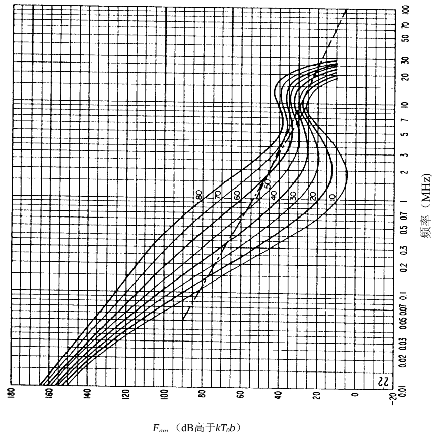
图 35b-无线电噪声随频率的变化 (秋季; 0800-1200LT)
