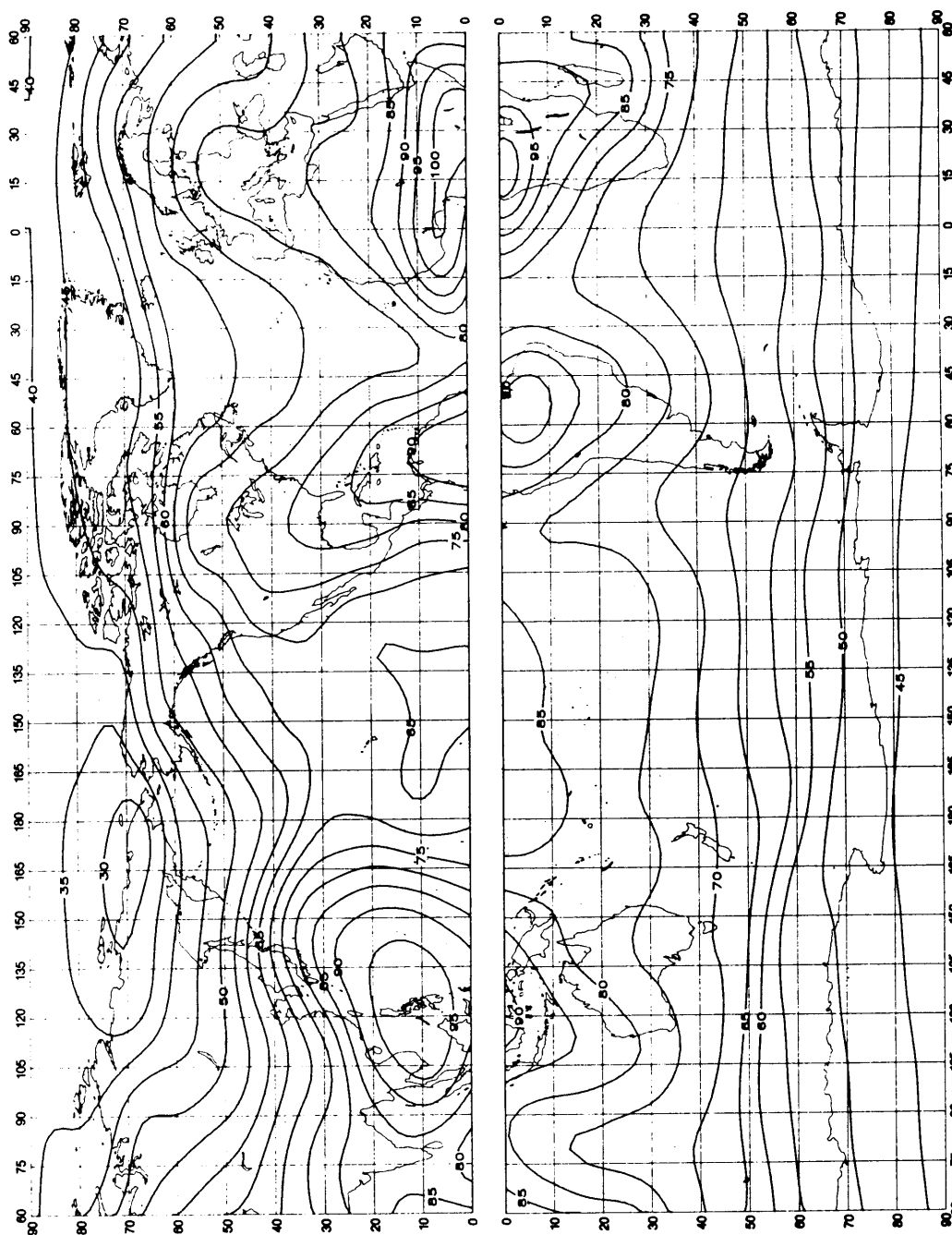
图38a-大气无线电噪声的预计值, F_{am} (1 MHz的dB高于 kT_{0b} ) (秋季; 2000-2400LT)
