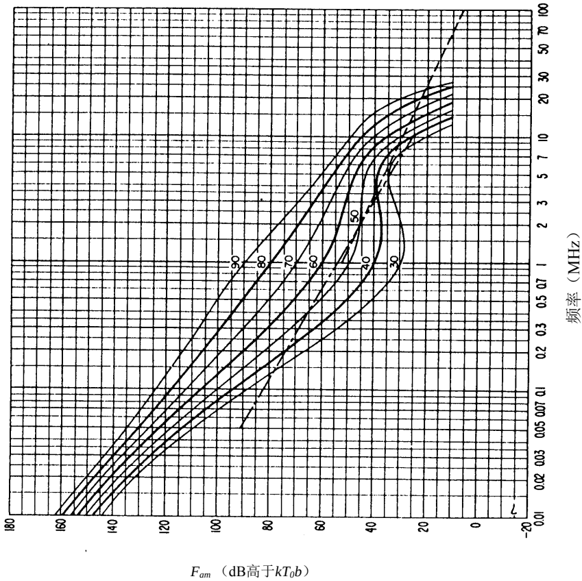
图 20b-无线电噪声随频率的变化 (冬季; 2000-2400LT)
