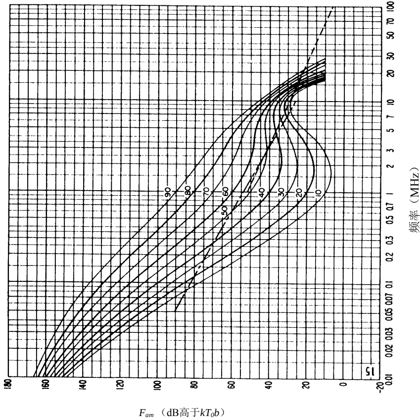
图 28b-无线电噪声随频率的变化 (夏季; 0400-0800LT)
