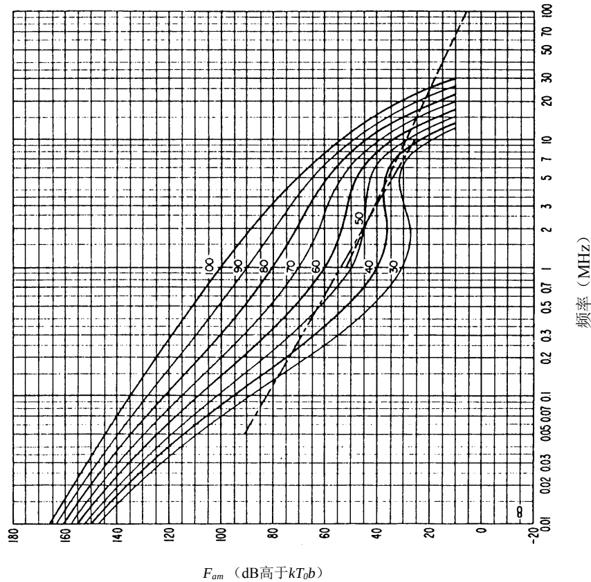
图 21b-无线电噪声随频率的变化 (春季; 0000-0400LT)
