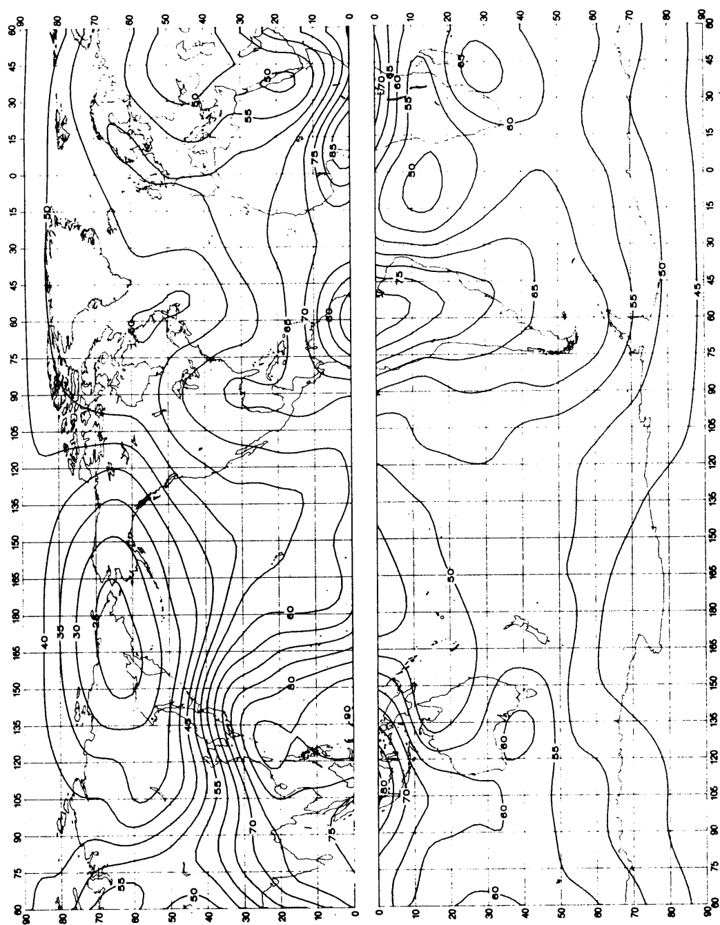
图19a-大气无线电噪声的预计值, F_{am} (1 MHz的dB高于 kT_{0b} ) (冬季; 1600-2000LT)
