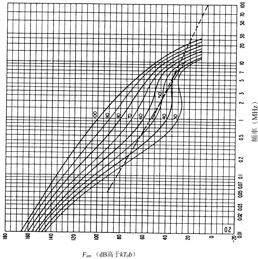
图 33b-无线电噪声随频率的变化 (秋季; 0000-0400LT)
