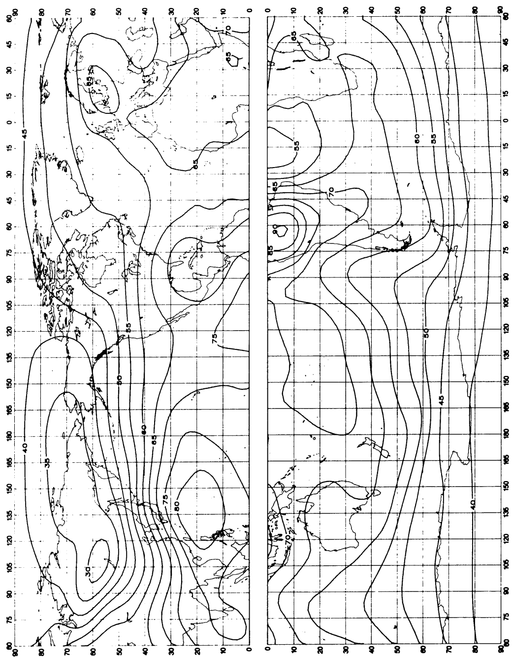
图16a-大气无线电噪声的预计值, F_{am} (1 MHz的dB高于 kT_0b ) (冬季; 0400-0800LT)
