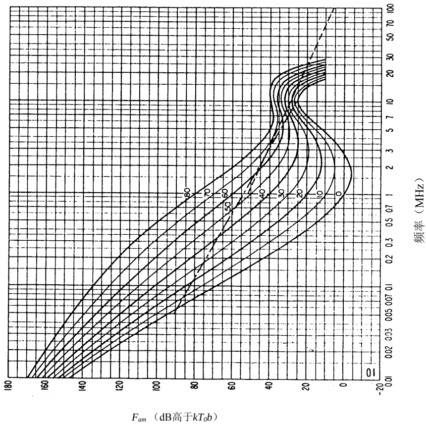
图 23b—无线电噪声随频率的变化 (春季; 0800-1200LT)
