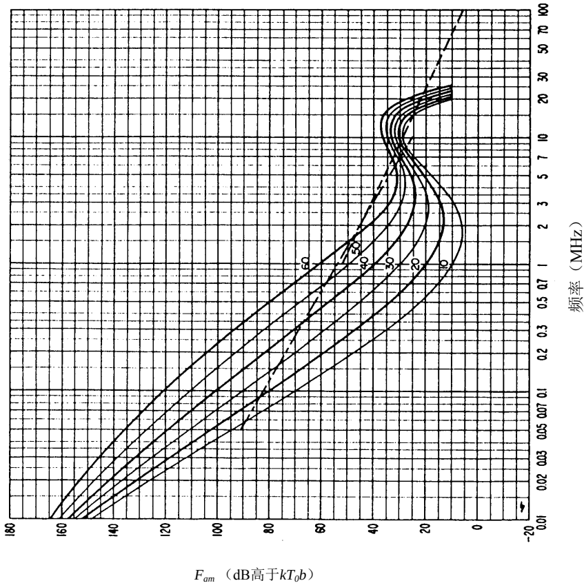
图 17b-无线电噪声随频率的变化 (冬季; 0800-1200LT)
