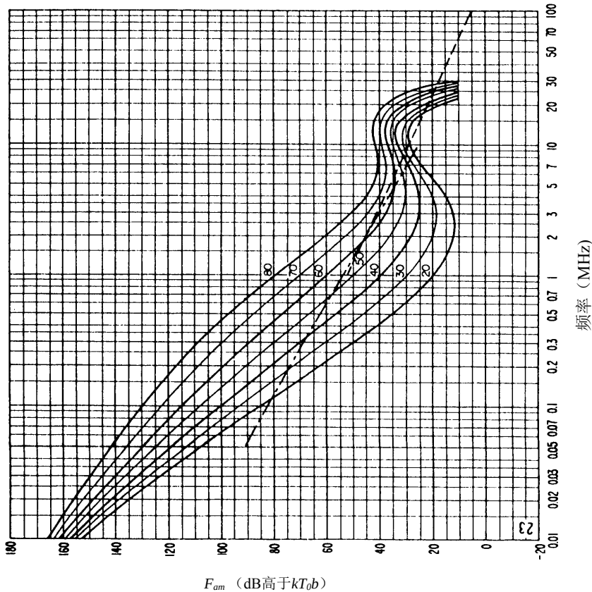
图 36b-无线噪声随频率的变化 (秋季; 1200-1600LT)
