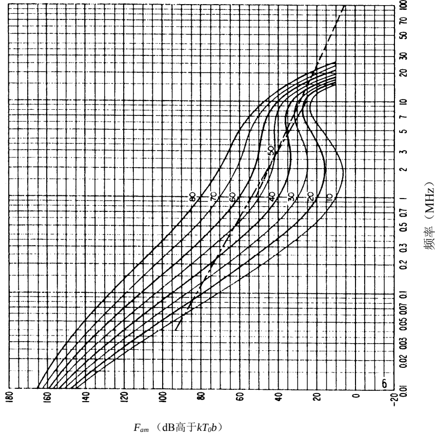
图 22b-无线电噪声随频率的变化 (春季; 0400-0800LT)
