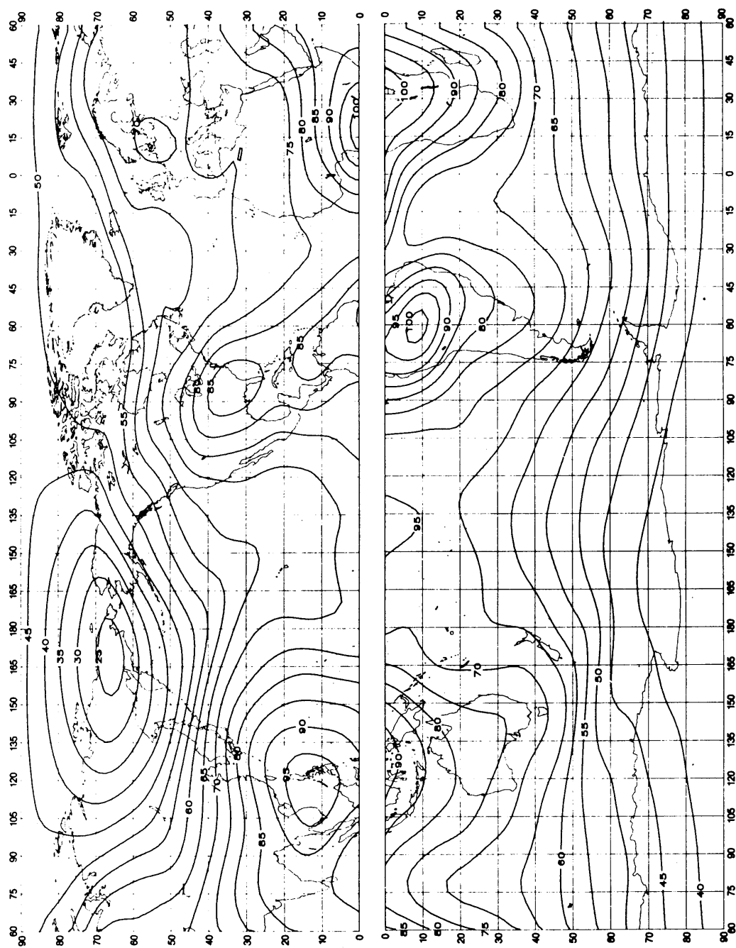
图26a-大气无线电噪声的预计值, F_{am} (1 MHz的dB高于 kT_{0b} ) (春季; 2000-2400LT)
