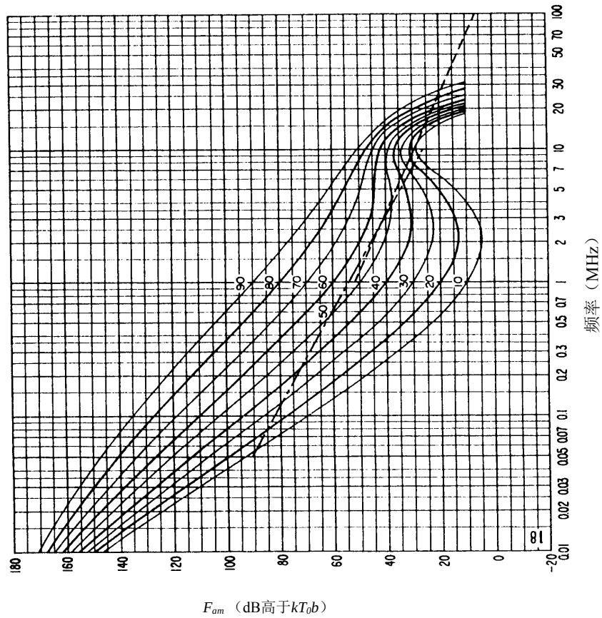
图 31b-无线电噪声随频率的变化 (夏季; 1600-2000LT)
