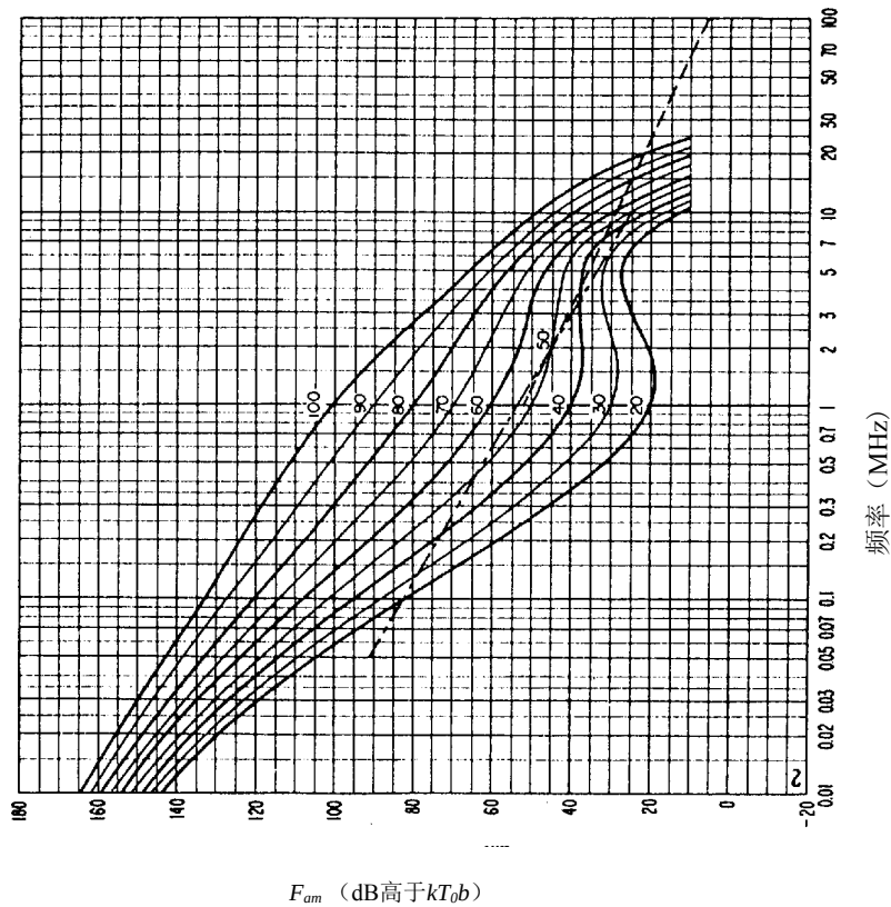
图 15b-无线电噪声随频率的变化
