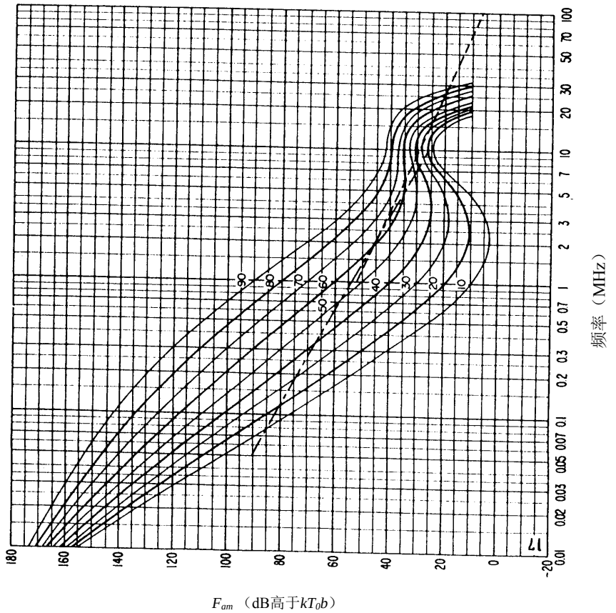
图 30b-无线电噪声随频率的变化 (夏季; 1200-1600LT)
