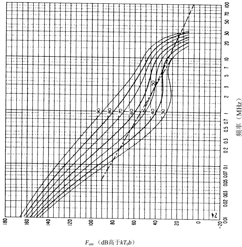
图 37b-无线电噪声随频率的变化 (秋季; 1600-2000LT)
