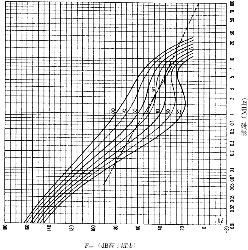
图 34b—无线 电噪声随频率的变化 (秋季; 0400-0800LT)
