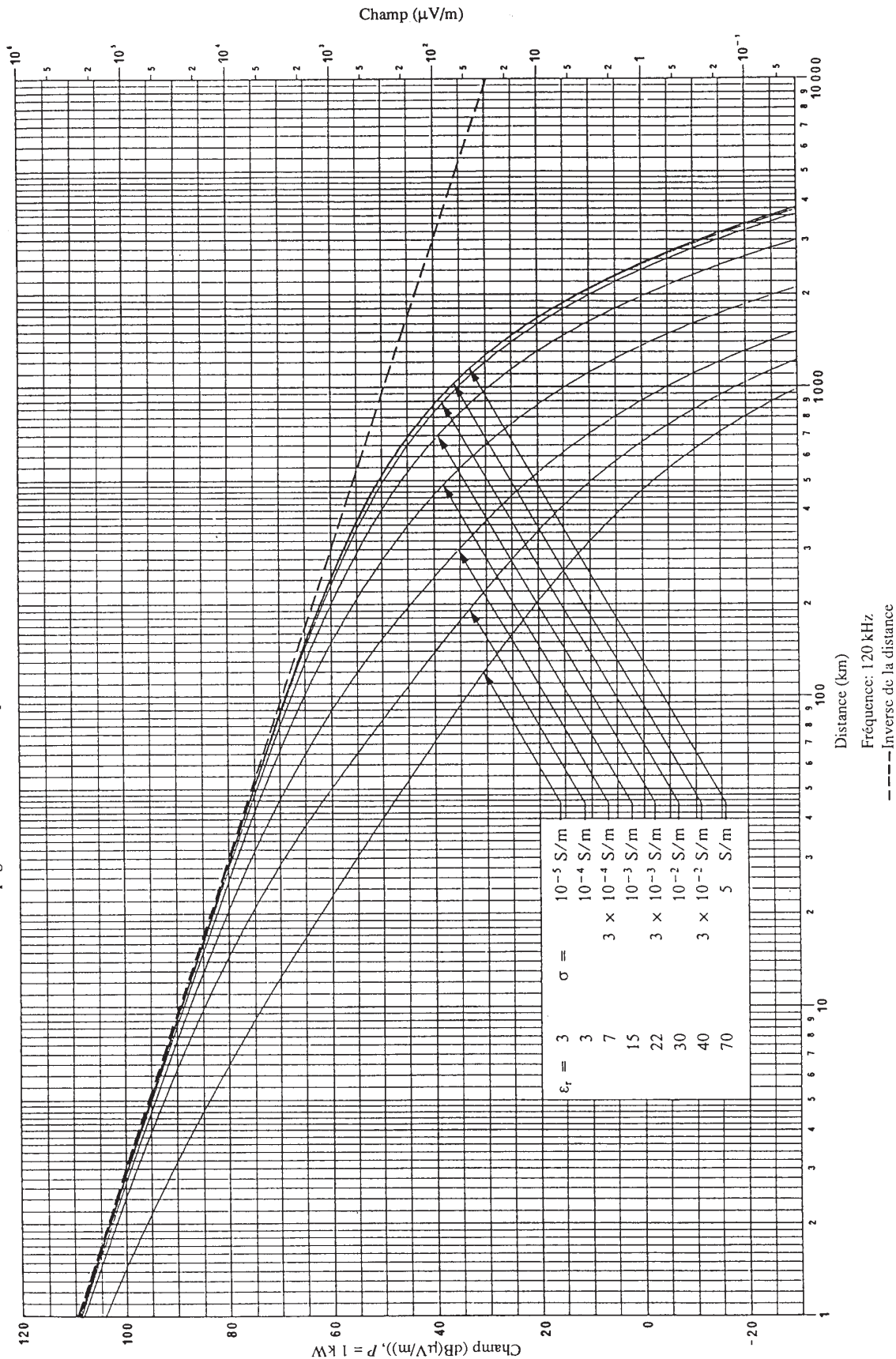
FIGURE 17 Propagation de l'onde de sol pour différentes valeurs de \sigma et \epsilon_r
