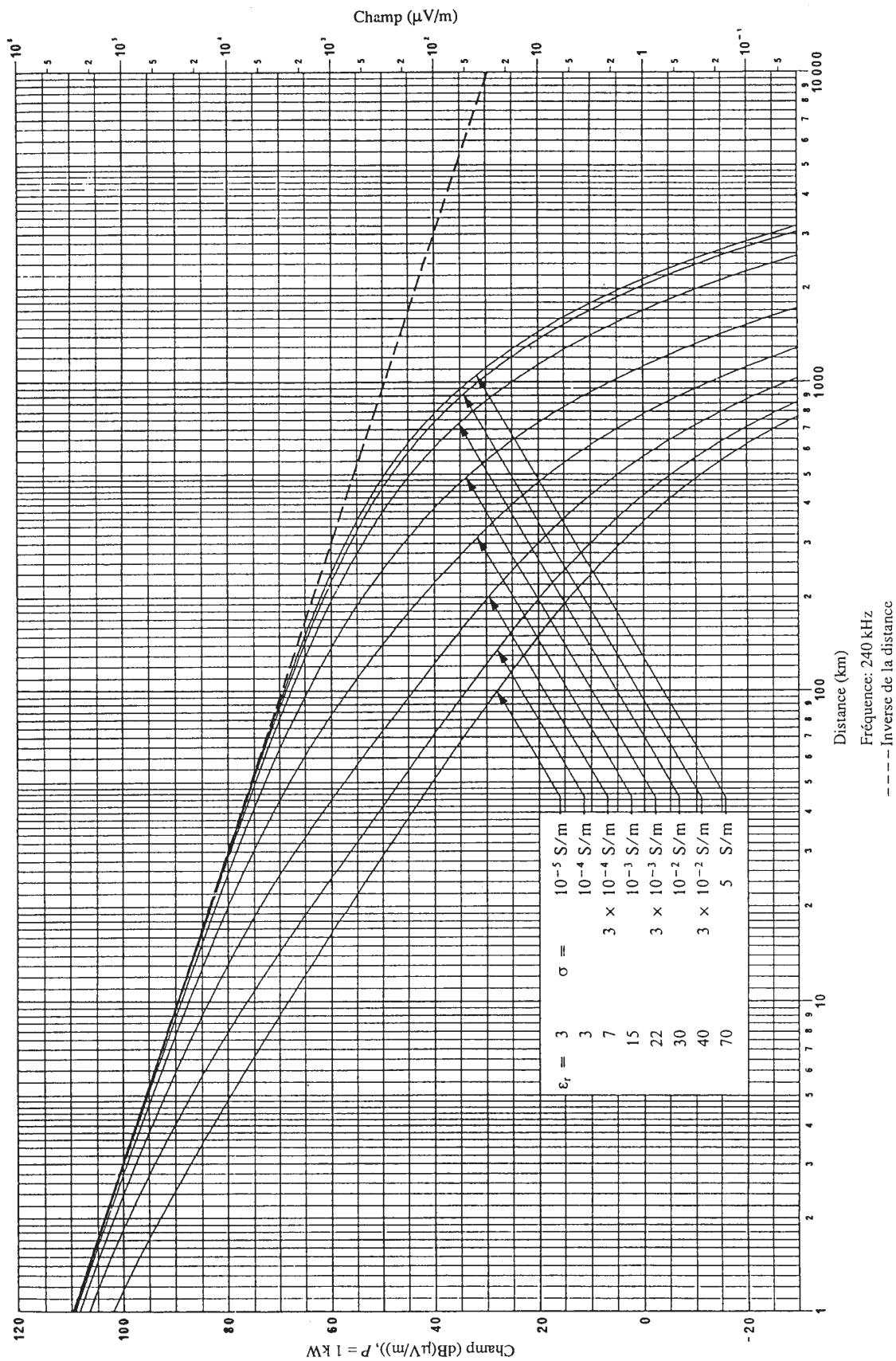
FIGURE 21 Propagation de l'onde de sol pour différentes valeurs de \sigma et \epsilon_r
