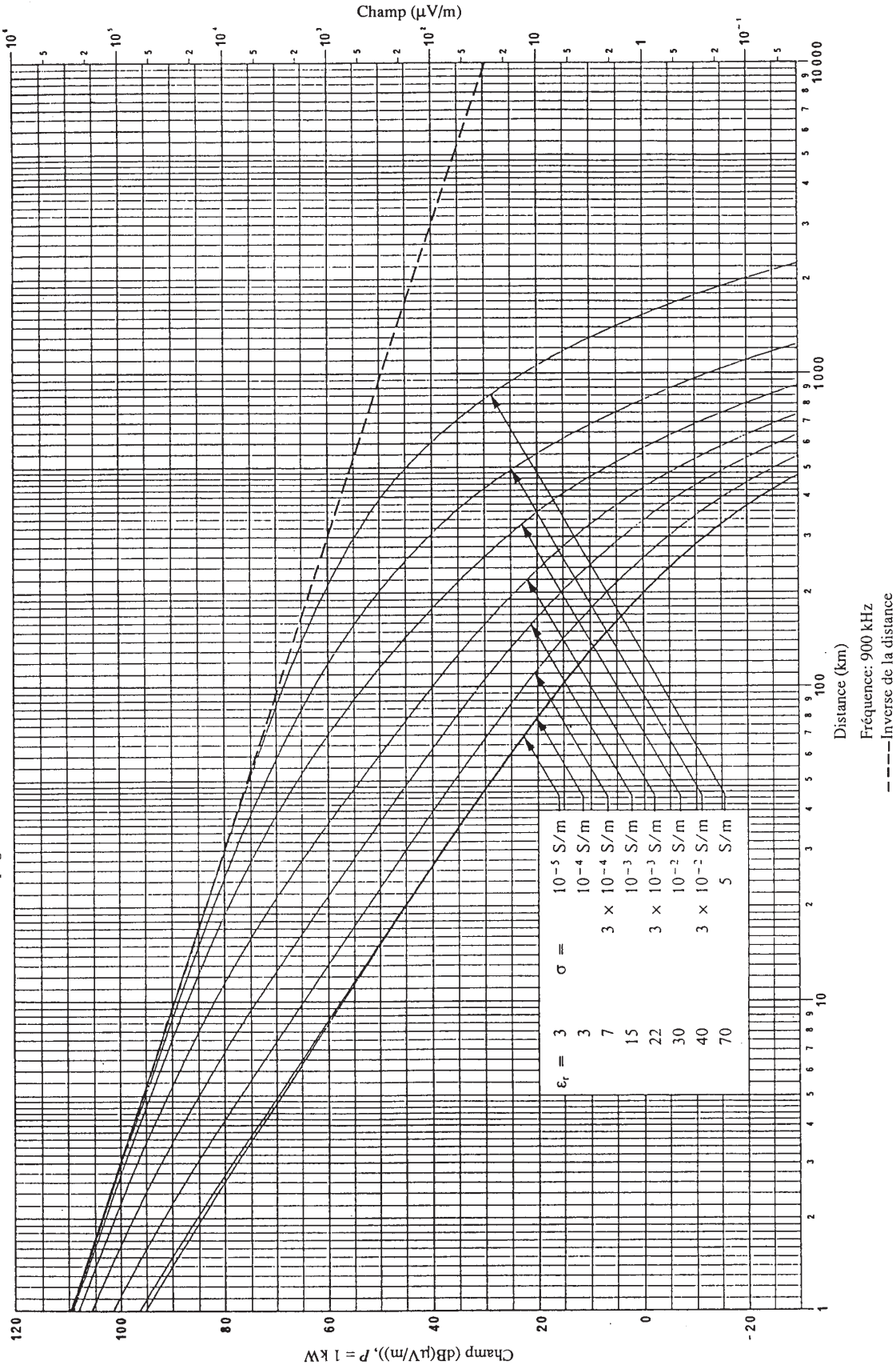
FIGURE 29 Propagation de l'onde de sol pour différentes valeurs de \sigma et \epsilon_r
