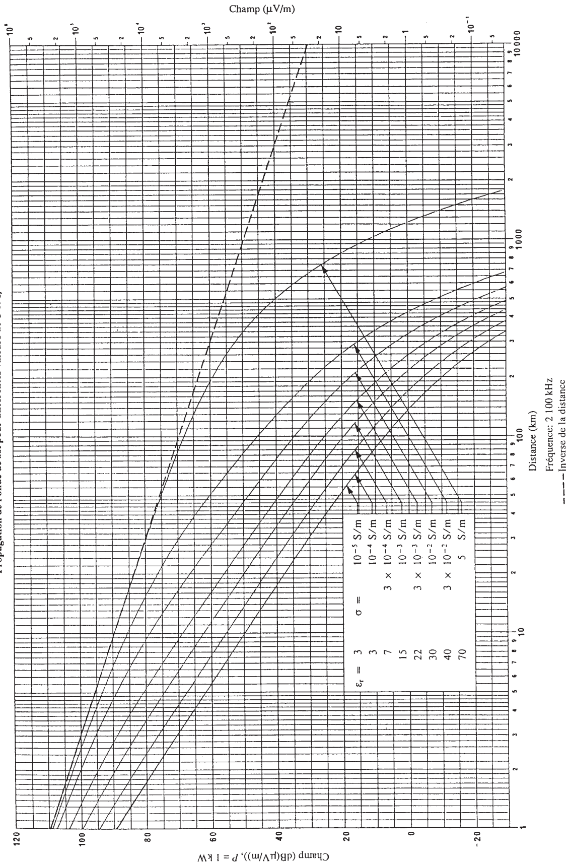
FIGURE 41 Propagation de l'onde de sol pour différentes valeurs de \sigma et \epsilon_r
