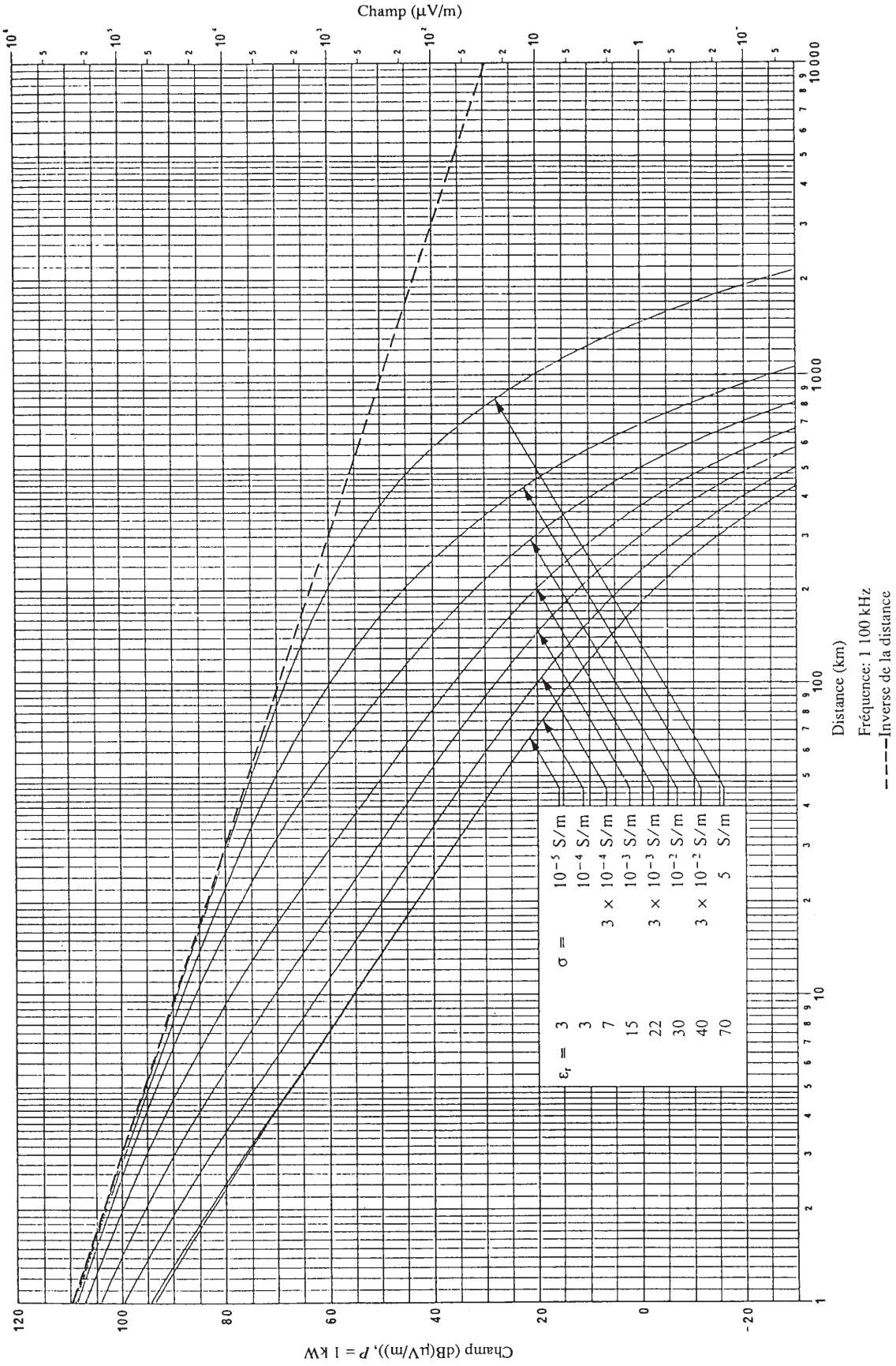
FIGURE 31 Propagation de l'onde de sol pour différentes valeurs de \sigma et \epsilon_r
