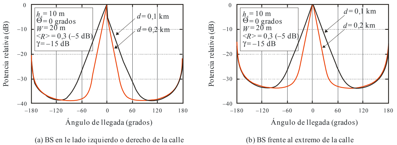
Perfil angular de llegada en la estación móvil para entornos LoS
