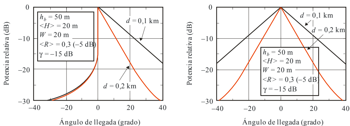
Perfil angular de llegada en la estación de base AOD_{LoS,pow}(\Delta\theta,d) para entornos LoS
