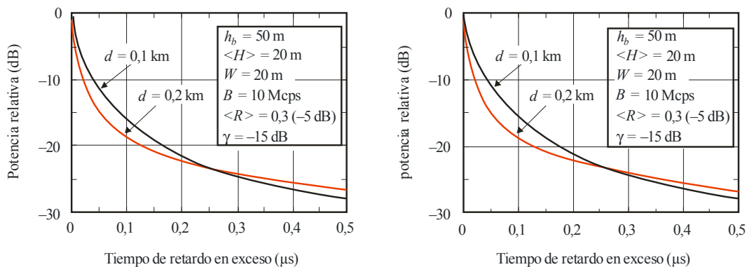
Perfil de envoltura del retardo PDP_{LoS,env}(\tau, d) para entornos LoS
