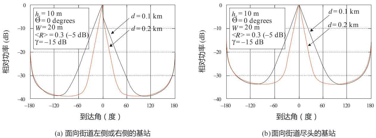
用于 LoS 环境的基站到达角 AOD_{LoS, pow}(\Delta\theta, d)
