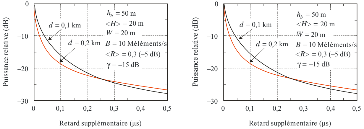
(a) Station de base faisant face au côté gauche ou droit de la rue
