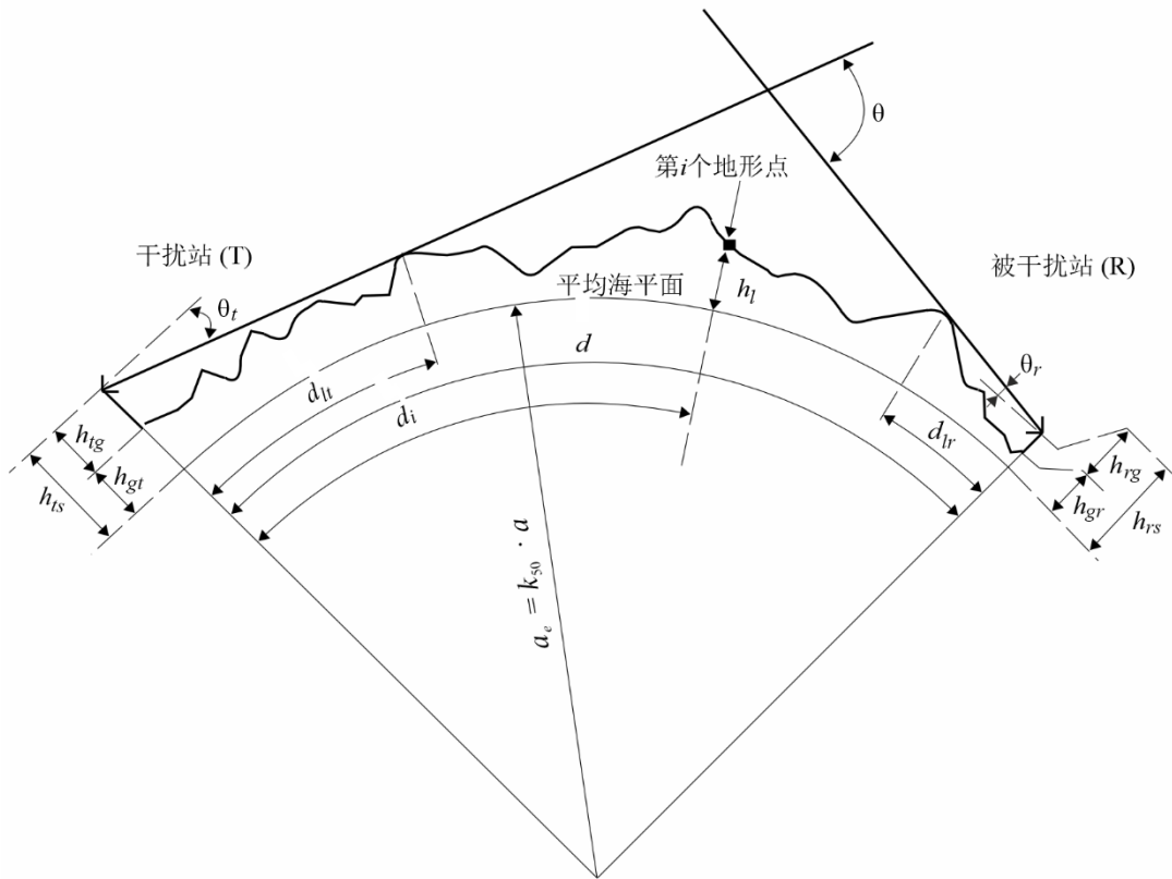
图 1 (超地平线) 路径剖面的一个例子
