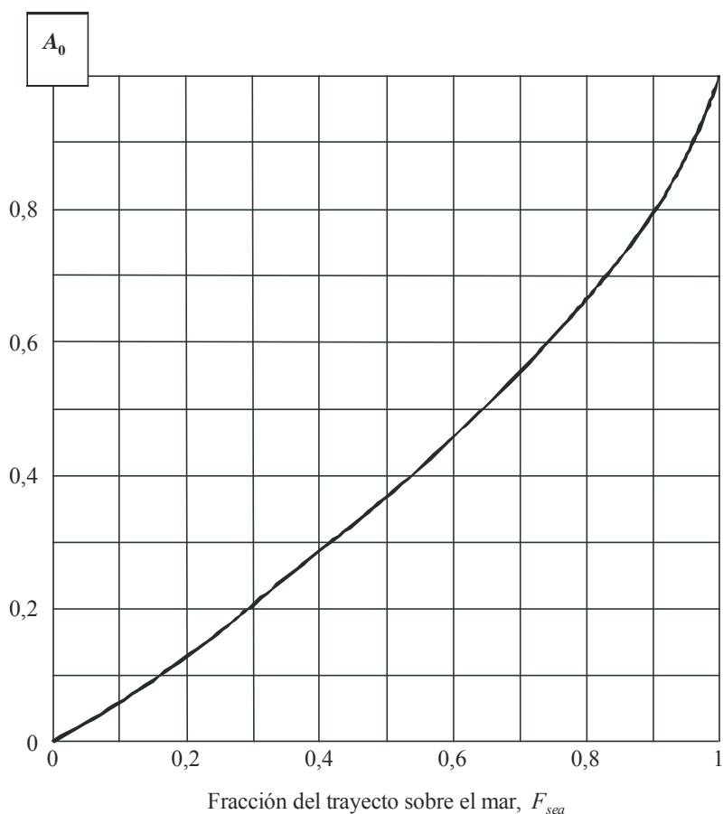
Factor de interpolación básico, A_0 , para propagación mixta
