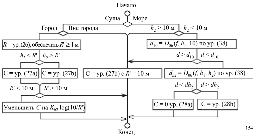
Блок-схема для поправки к высоте приемной/подвижной антенны
