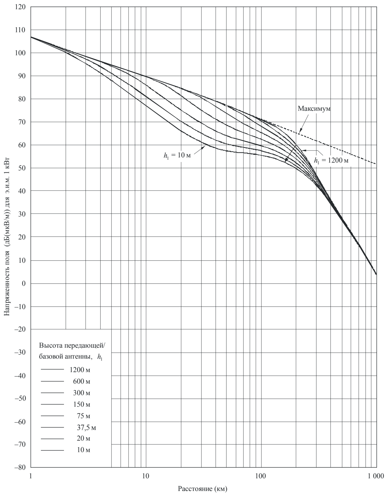
РИСУНОК 14 600 МГц, трасса над холодным морем, 1% времени
