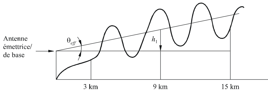
Angle de dégagement équivalent pour h_1 < 0
