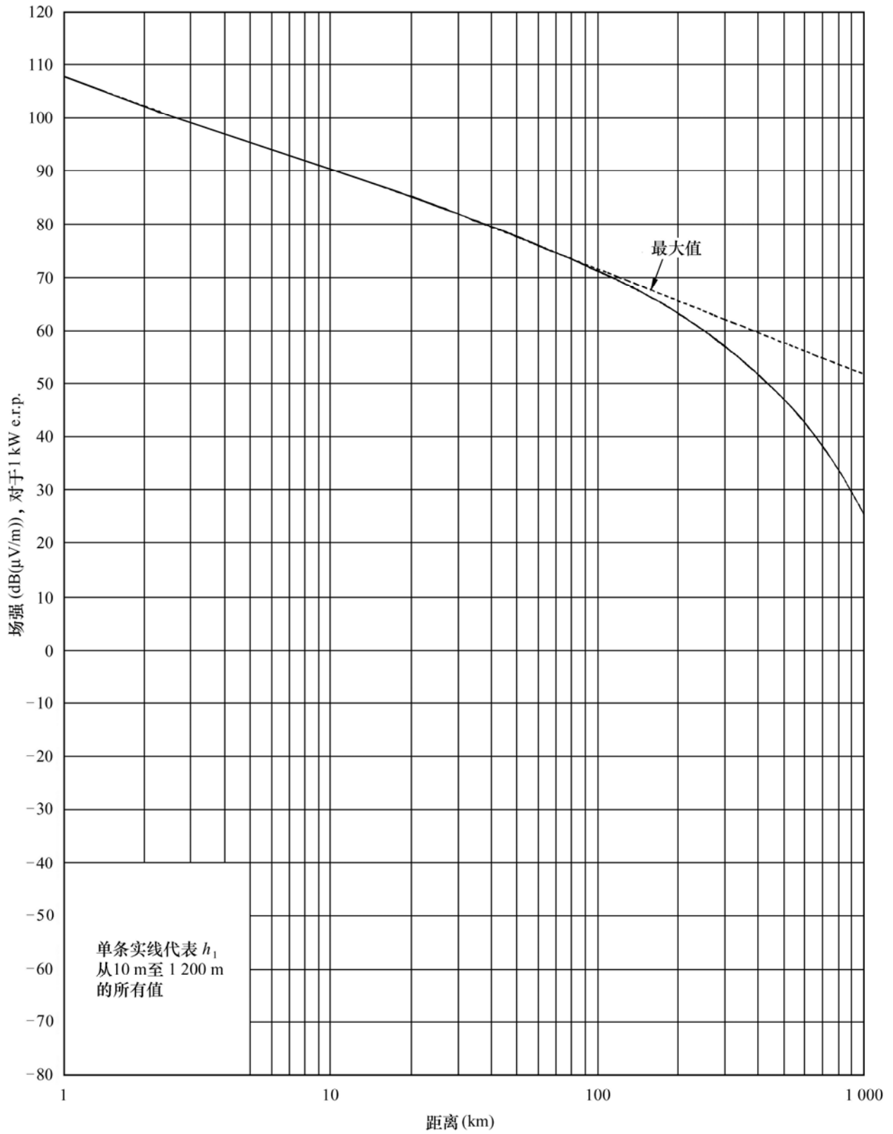
图 24 2 000 MHz, 暖海路径, 1%时间
