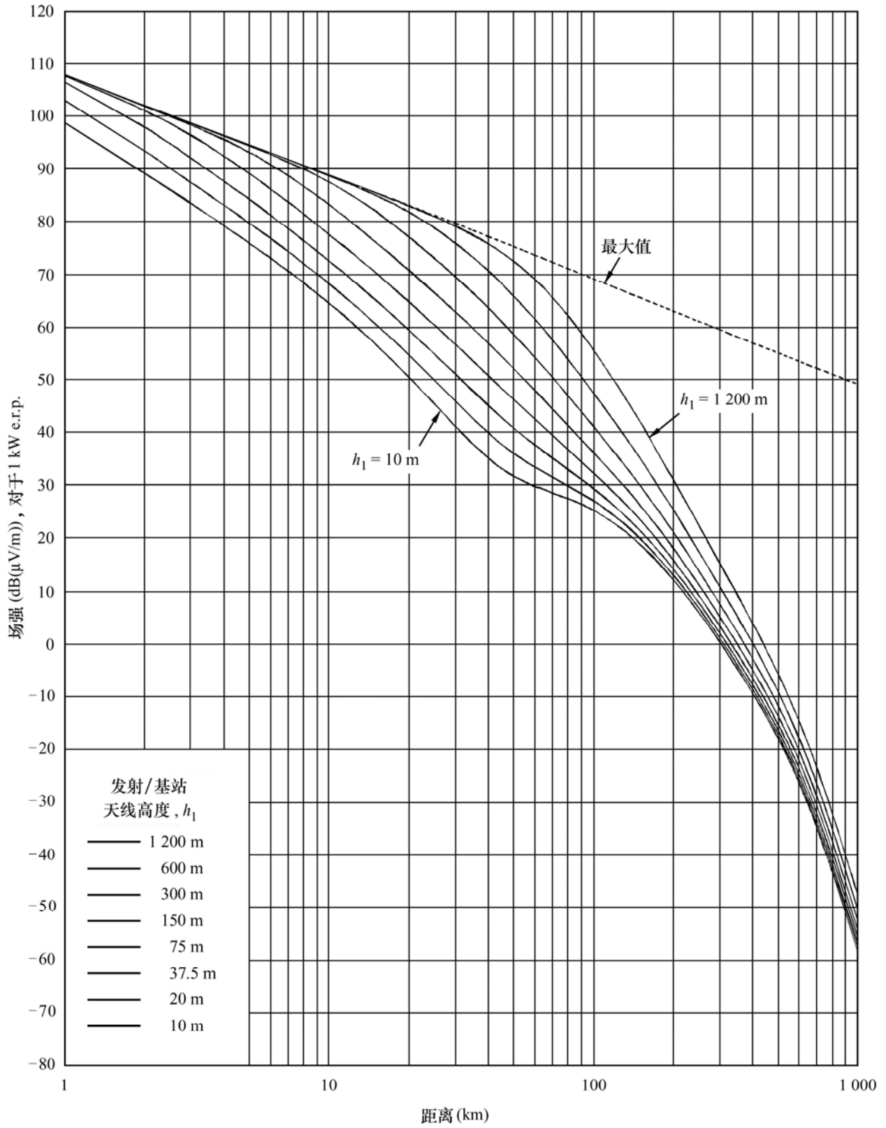
图 5 100 MHz, 冷海路径, 10%时间
