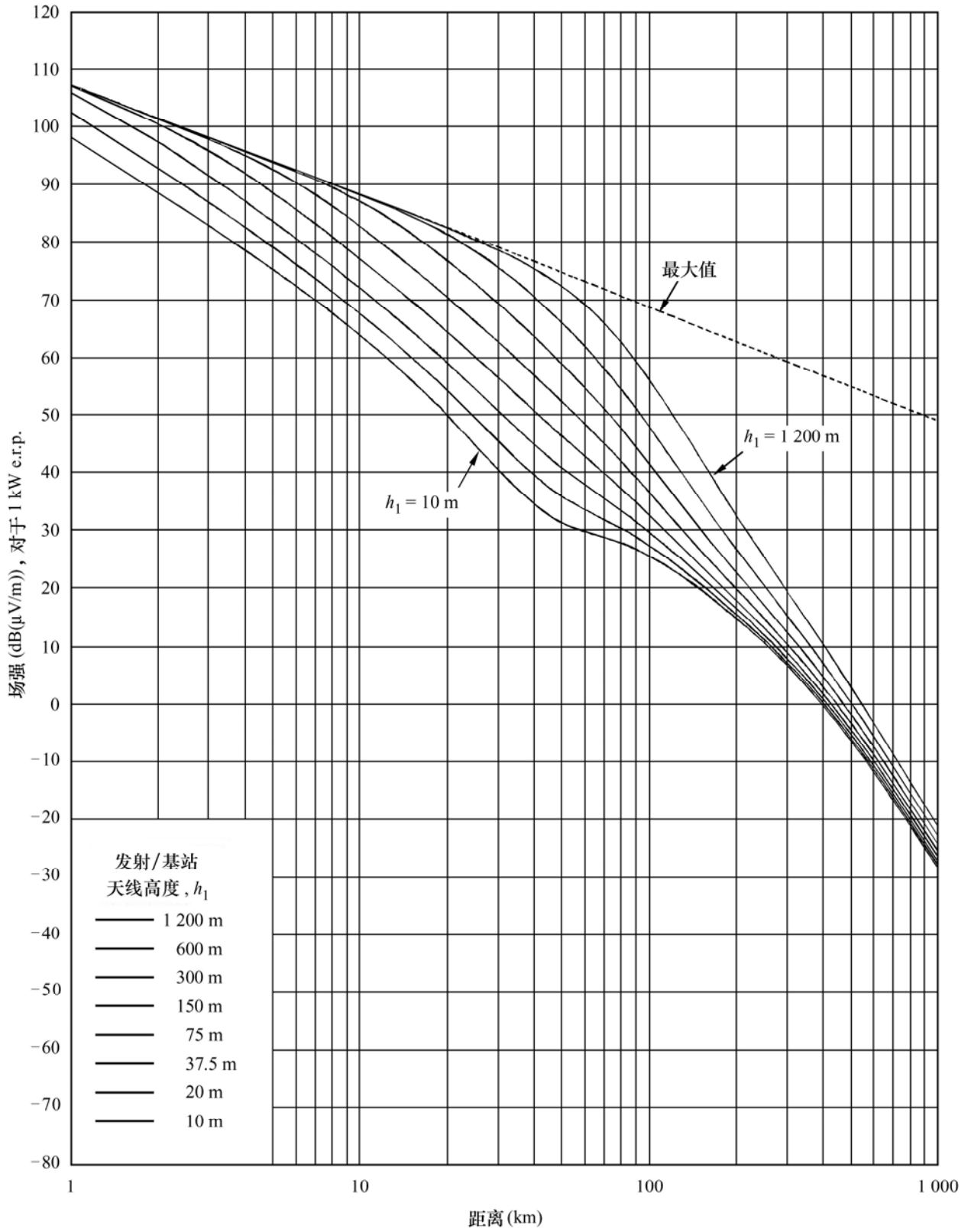
图 7 100 MHz, 暖海路径, 10%时间
