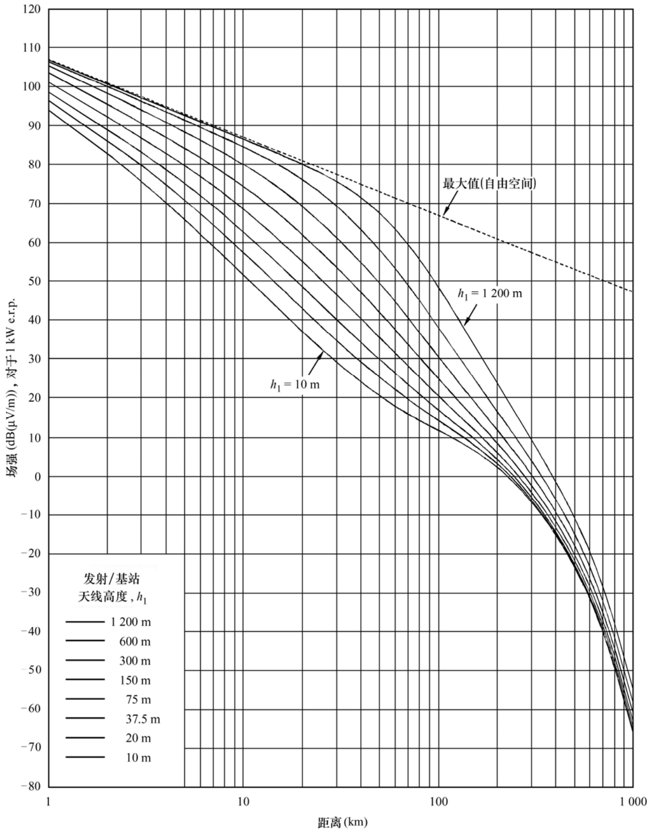
图 19 2 000 MHz, 陆地路径, 1%时间
