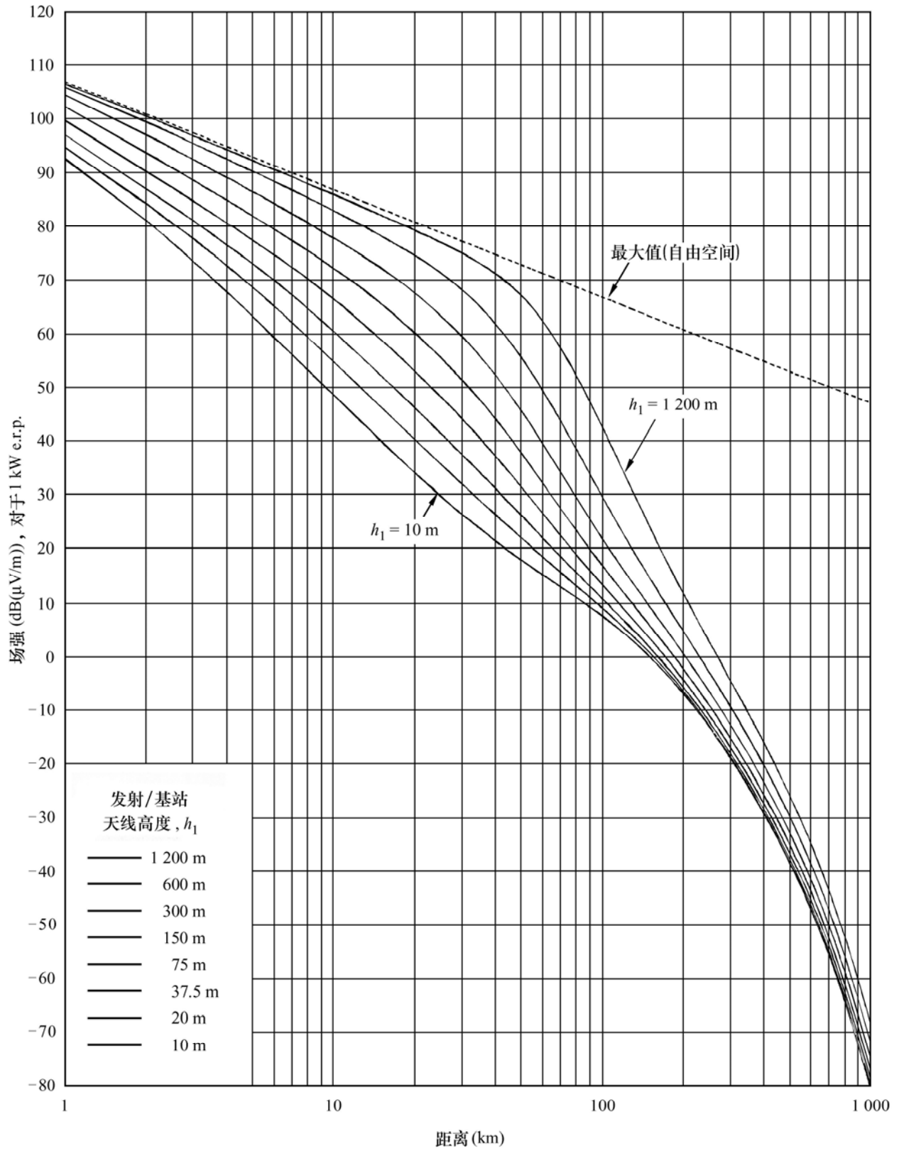
图9 600 MHz, 陆地路径, 50%时间
