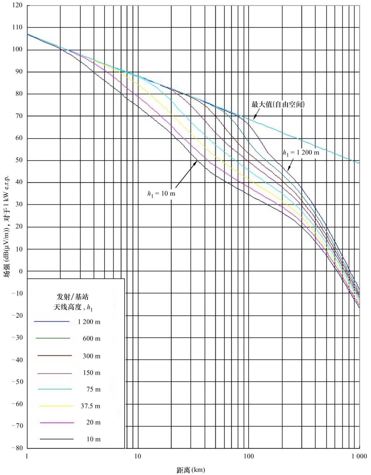
图 15 600 MHz, 暖海路径, 10%时间
