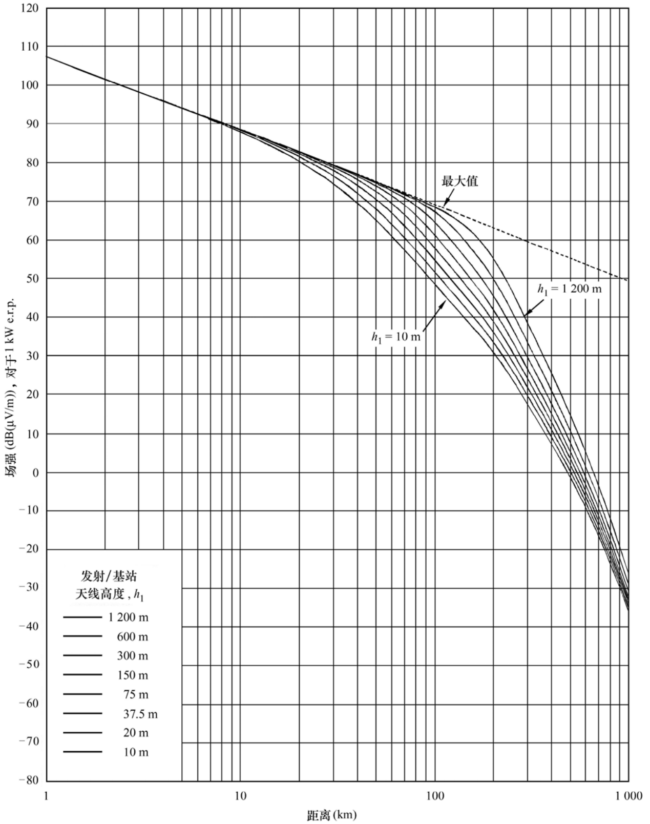
图 21 2 000 MHz, 冷海路径, 10%时间
