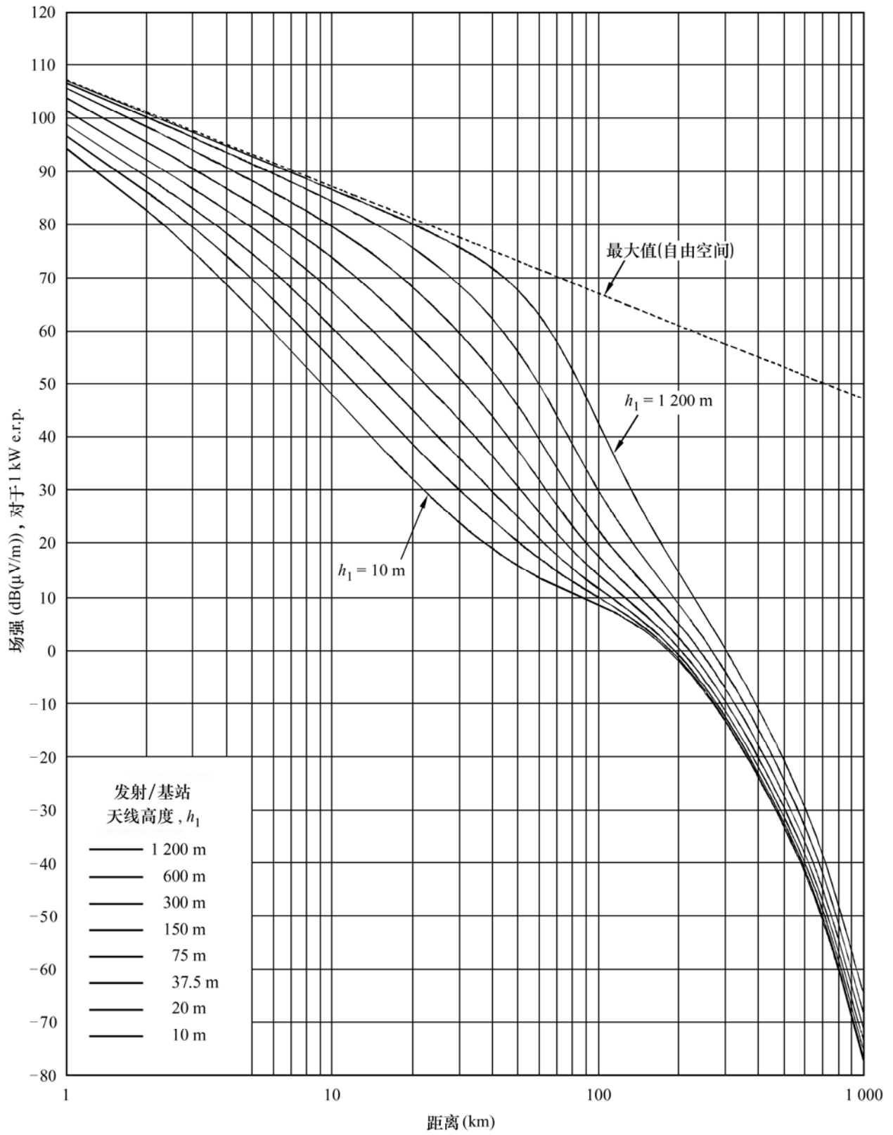
图 18 2 000 MHz, 陆地路径, 10%时间
