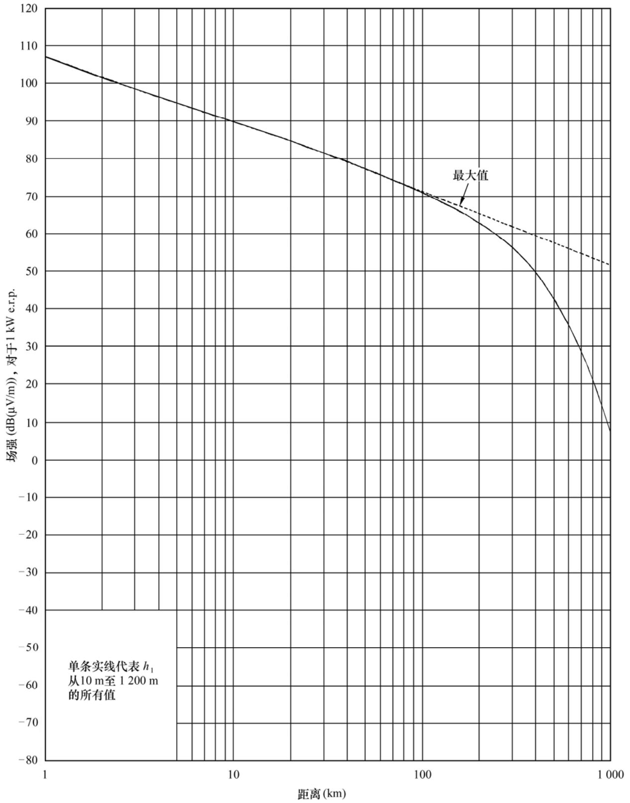
图 22 2 000 MHz, 冷海路径, 1%时间
