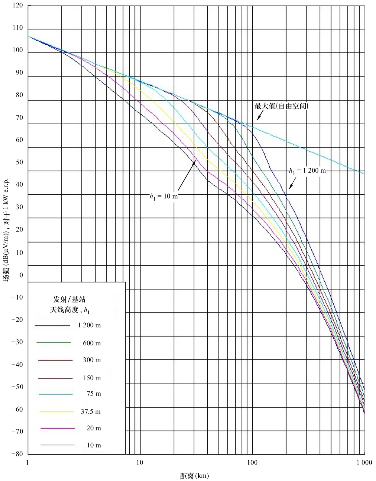
图13 600 MHz, 冷海路径, 10%时间
