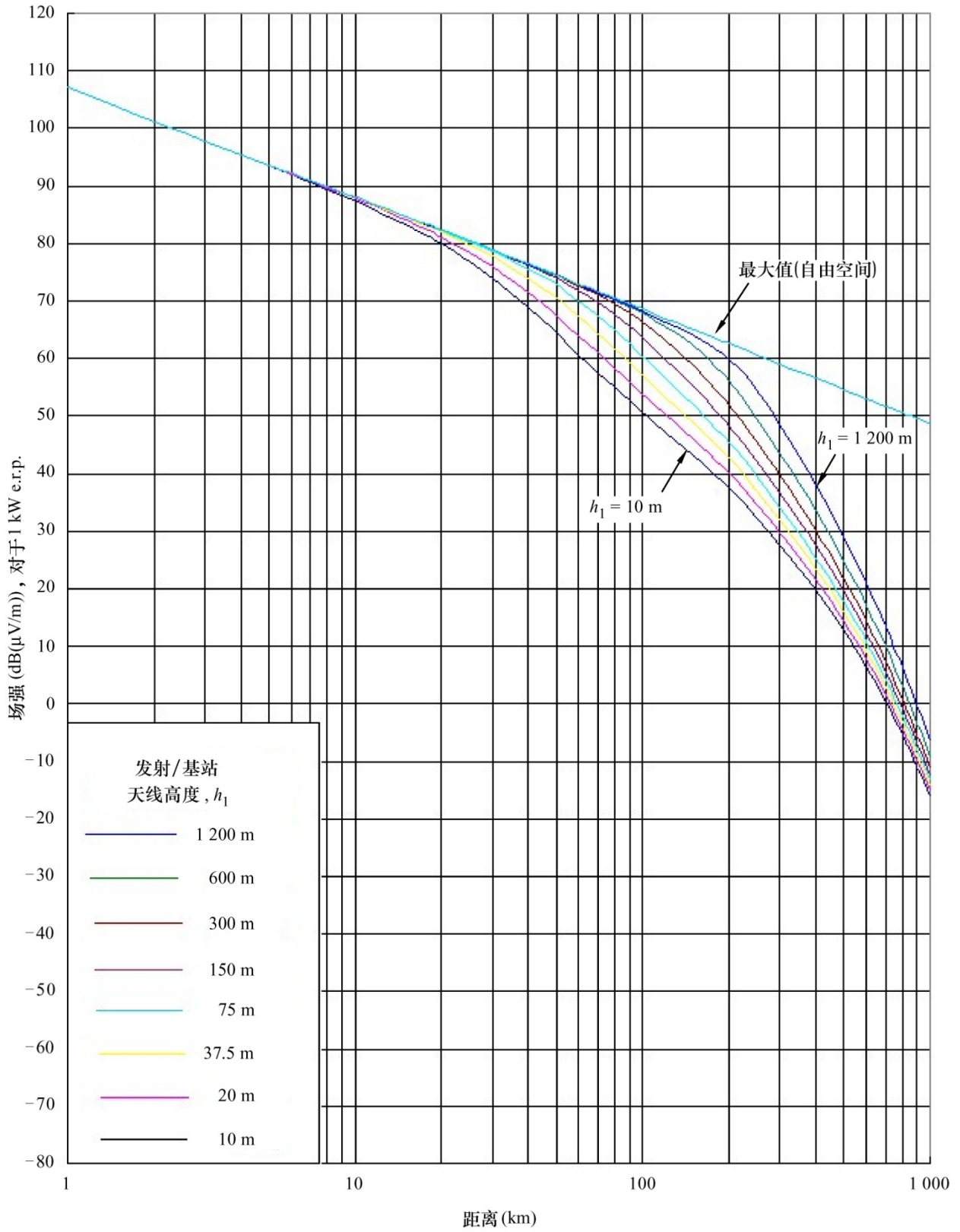
图 23 2 000 MHz, 暖海路径, 10%时间
