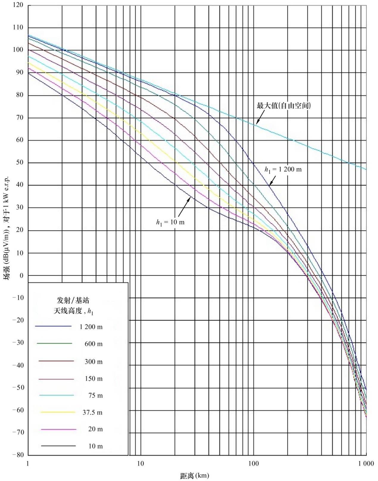
图 2 100 MHz, 陆地路径, 10%时间
