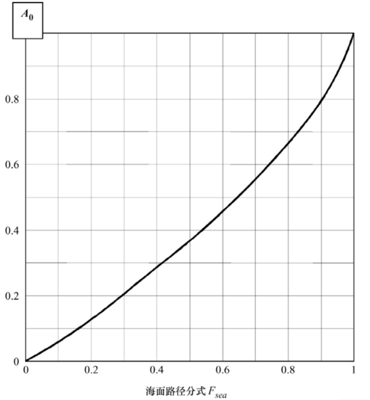
混合传播中海面的基本内插系数 A_0
