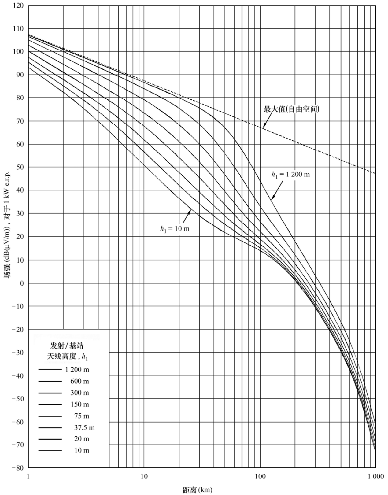
图 10 600 MHz, 陆地路径, 10%时间
